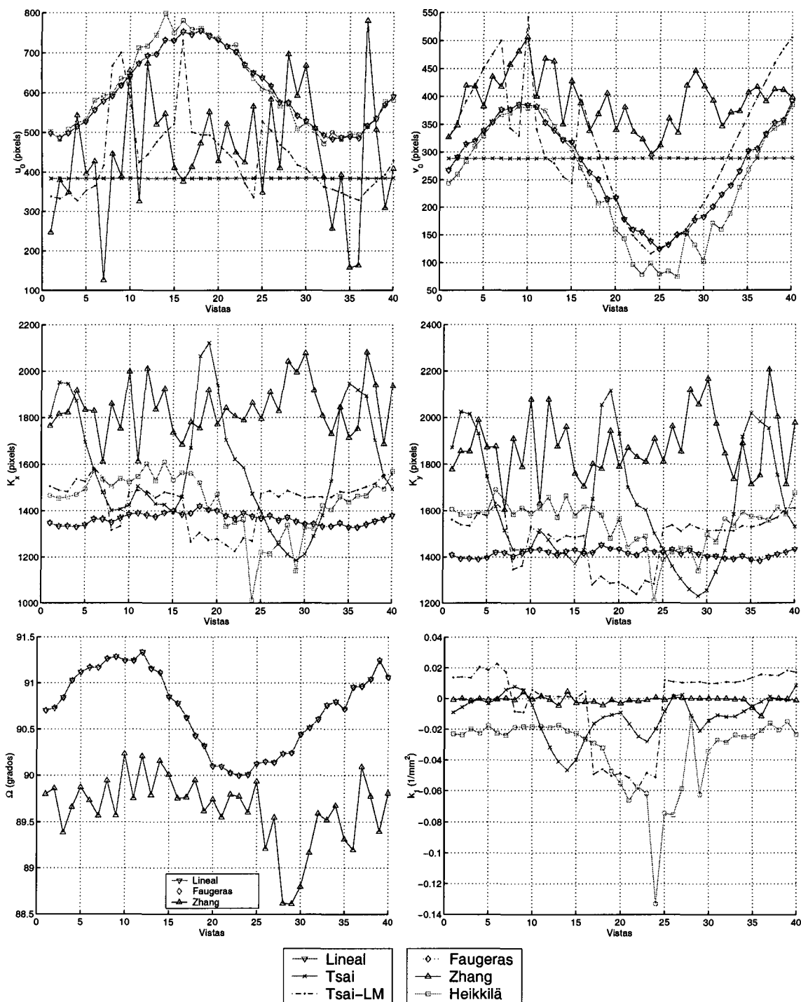
Figura 5.10: Estimación de los parámetros intrínsecos obtenidos por los métodos clásicos al variar los ángulos de azimuth y elevación de la cámara.
