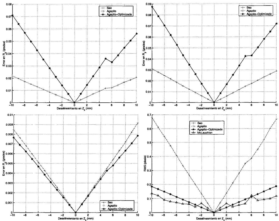
Figura 4.31: Error en la orientación y RMS sobre las coordenadas 2D cuando varía la distancia a lo largo del eje óptico ( Z ) entre el foco y el eje de giro de la cámara. Las imágenes están libres de ruidos.
