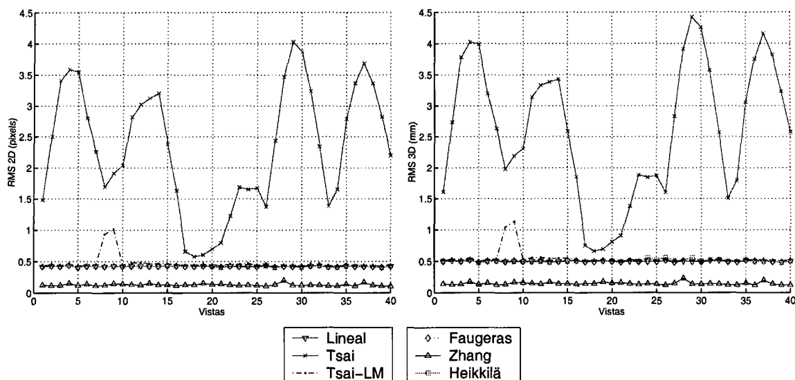
Figura 5.12: Error en la reconstrucción de las coordenadas de los puntos obtenidos por los métodos clásicos al variar los ángulos de azimuth y elevación de la cámara.
