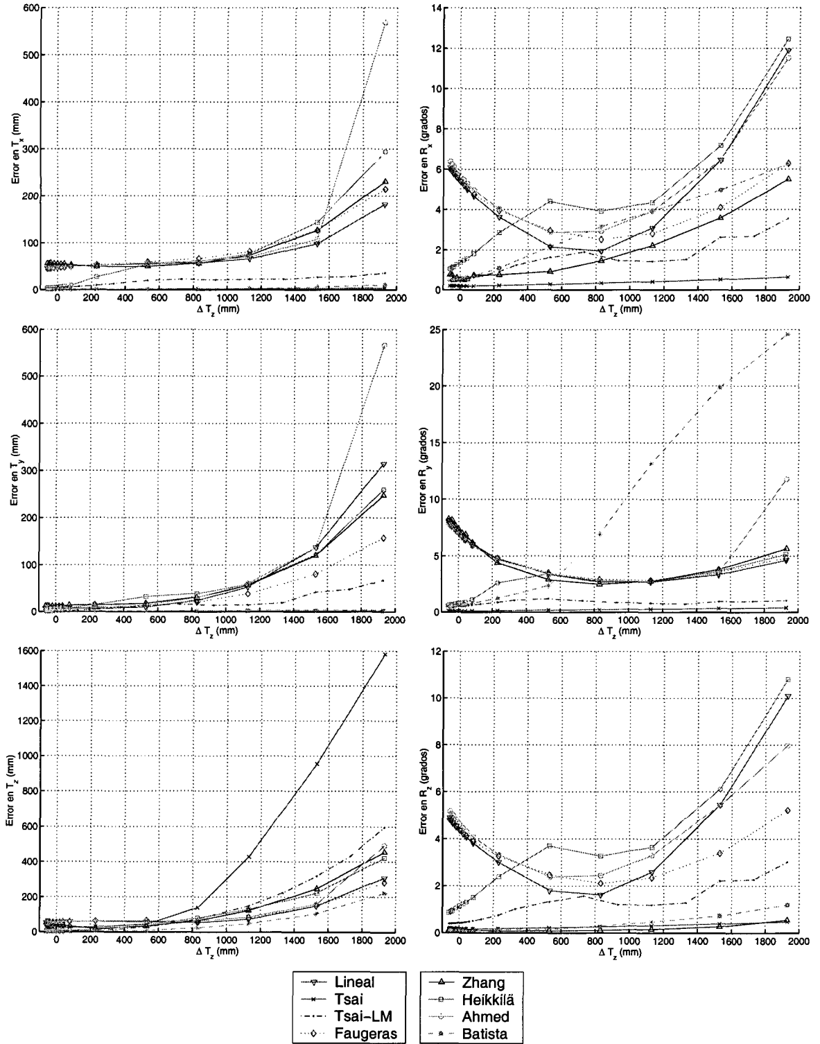
Figura 2.41: Error en el cálculo de los parámetros extrínsecos ante la variación de la distancia entre el patrón y la cámara usando imágenes con ruido de 0.5 pixels en las coordenadas 2D.
