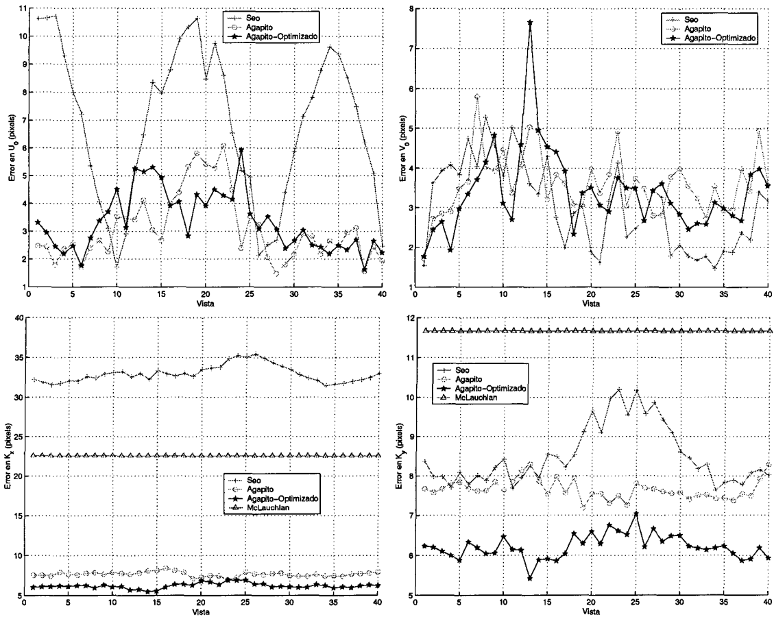
Figura 4.16: Error en la estimación de cada parámetro intrínseco para cada una de las vistas. Las imágenes tienen un ruido gaussiano de 0.5 pixels en sus coordenadas 2D. El centro óptico se incrementa linealmente a lo largo de la secuencia.
