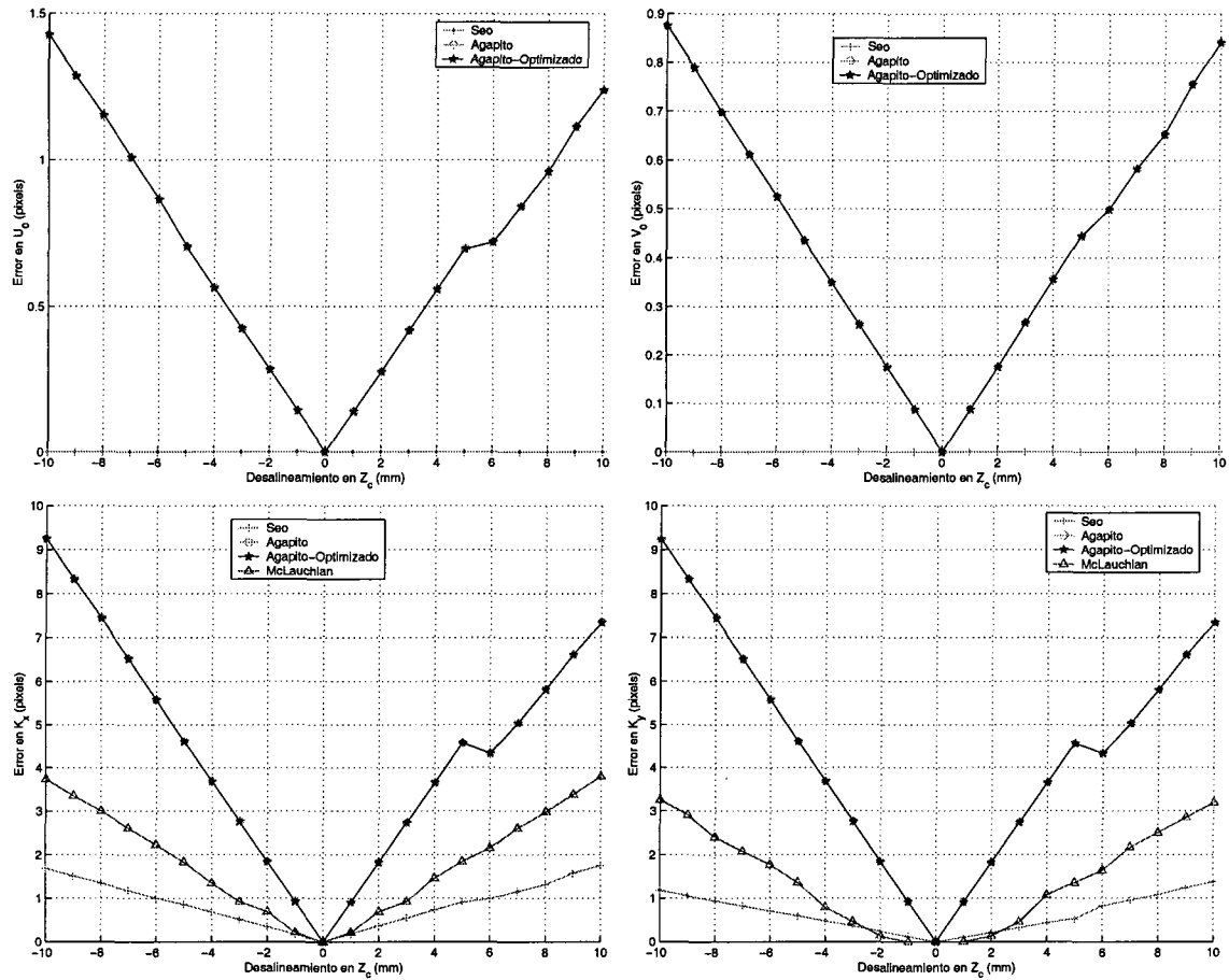
Figura 4.30: Error de cada parámetro intrínseco cuando varía la distancia a lo largo del eje óptico ( Z ) entre el foco y el eje de giro de la cámara. Las imágenes están libres de ruidos.
