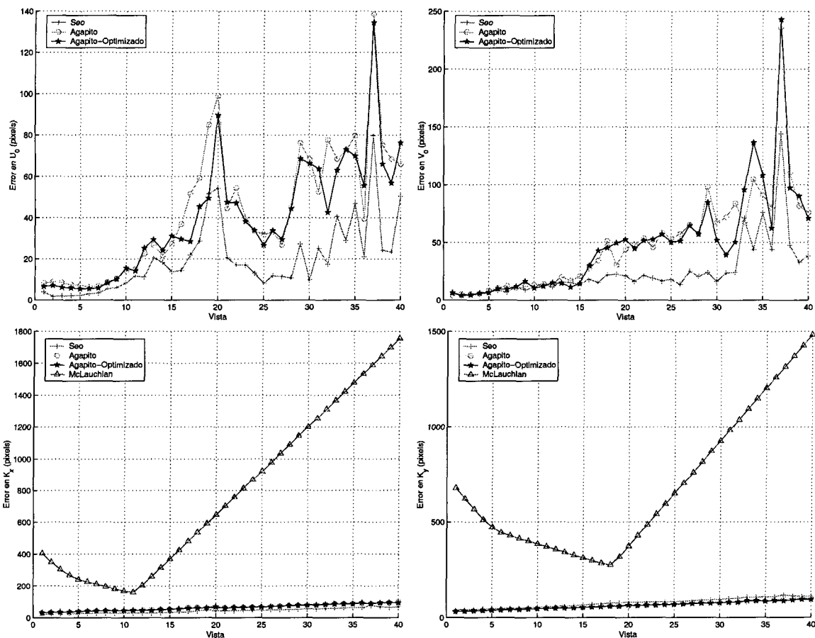
Figura 4.13: Error en la estimación de cada parámetro intrínseco para cada una de las vistas. Las imágenes tienen un ruido gaussiano de 0.5 pixels en sus coordenadas 2D. La distancia focal se incrementa linealmente a lo largo de la secuencia.
