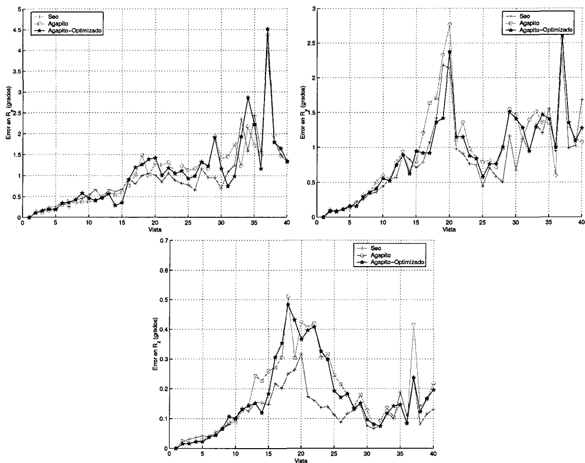
Figura 4.14: Error en la estimación de la orientación para cada una de las vistas. Las imágenes tienen un ruido gaussiano de 0.5 pixels en sus coordenadas 2D. La distancia focal se incrementa linealmente a lo largo de la secuencia.
