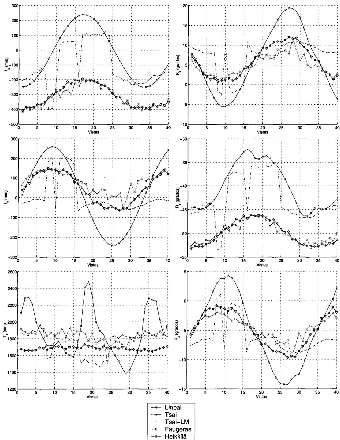
Figura 5.11: Estimación de los parámetros extrínsecos obtenidos por los métodos clásicos al variar los ángulos de azimut y elevación de la cámara.
