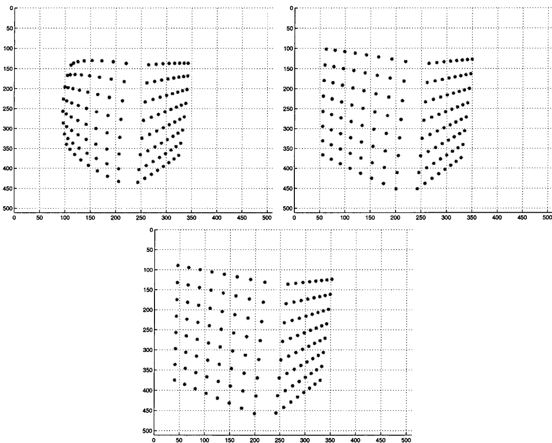
Figura 2.19: Proyección del diedro en la imagen. a) k_1 = -0,02 . b) k_1 = -0,005 . c) k_1 = -10^{-6} .
