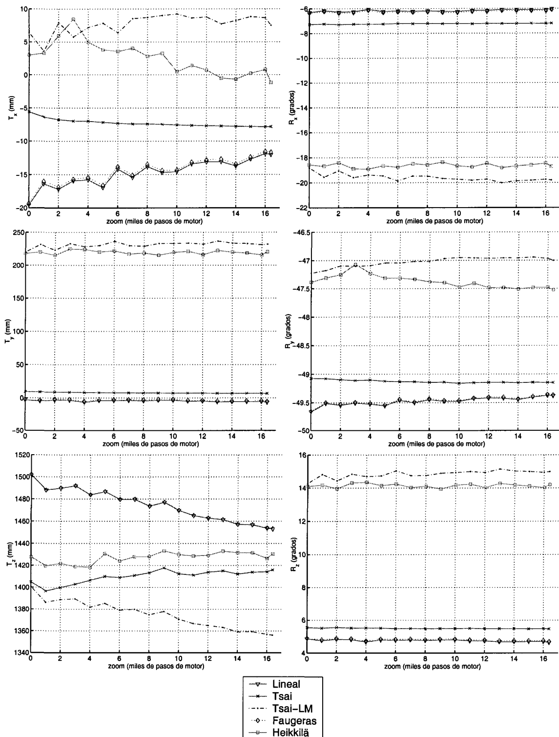
Figura 3.8: Resultados de la calibración del Conjunto 14x20. Valor de los parámetros extrínsecos para cada nivel de zoom.
