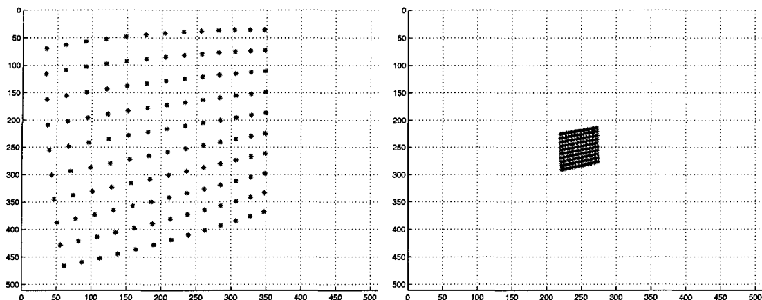
Figura 2.33: Patrón usado en el método de Batista situado a 39.3 cm y a 238.3 cm con distorsión en la imagen ( k_1 = -0,005 ).
