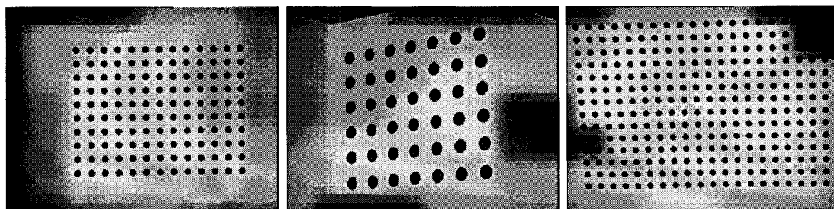
Figura 3.1: a) Patrón monoplano de 13x10 puntos. b) Patrón monoplano de 7x6 puntos. c) Patrón monoplano de 20x14 puntos.
