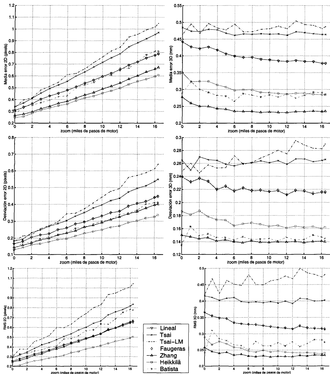
Figura 3.9: Resultados de la calibración del Conjunto 14x20. Error 2D (izquierda) y Error 3D (derecha) para cada nivel de zoom.
