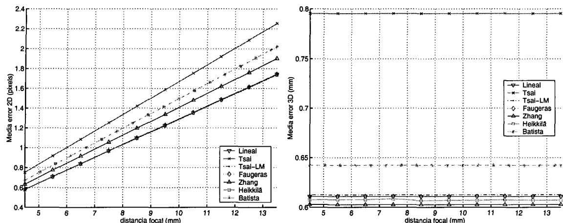
Figura 3.21: Error promedio en la reconstrucción en 2D y en 3D cuando varía la distancia focal en imágenes con ruido gaussiano de media nula y desviación típica de 0.5 mm en las coordenadas 3D.
