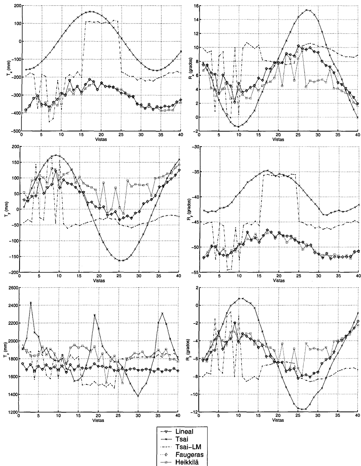
Figura 5.14: Estimación de los parámetros extrínsecos obtenidos al variar los ángulos de azimuth y elevación de la cámara. El zoom varía linealmente.
