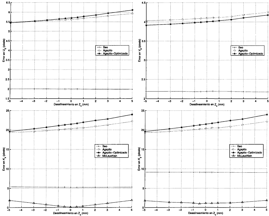
Figura 4.32: Error de cada parámetro intrínseco cuando varía la distancia en la dirección del eje óptico ( Z ) entre el foco y el eje de giro de la cámara. Las imágenes tienen un ruido gaussiano de media cero y desviación de 0.5 pixels.
