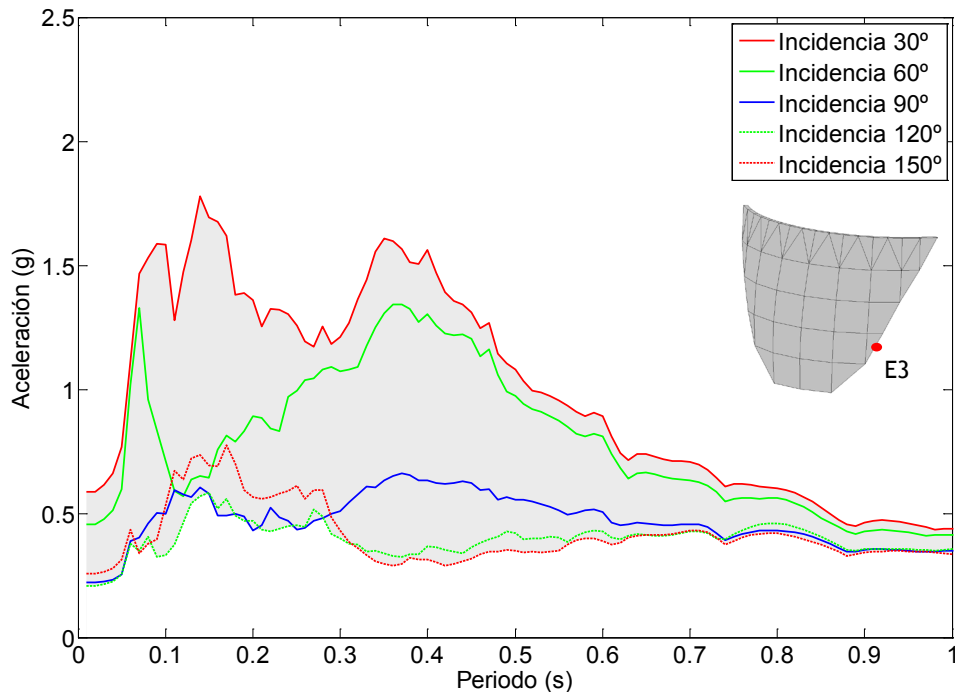
Figura 7.45. Nodo E3. Onda P+SV. Embalse con una capa de sedimentos de espesor 2H/5 . Espectro de aceleraciones en dirección y.
