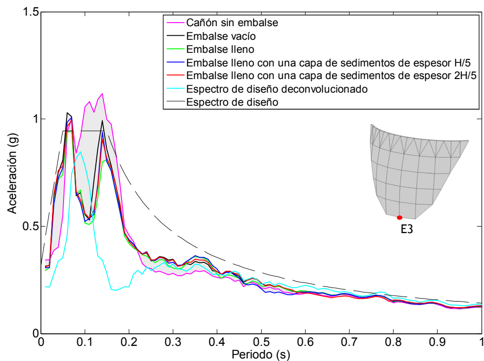
Figura 6.28. Nodo E3. Onda P. Espectro de aceleraciones en dirección z frente a diferentes condiciones del embalse.
