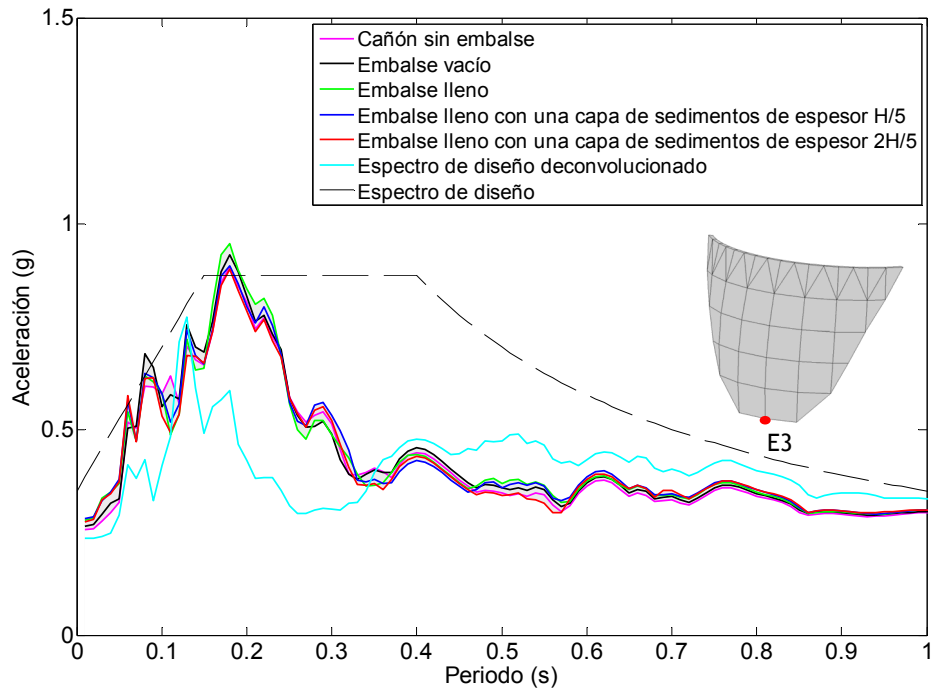
Figura 6.29. Nodo E3. Onda SH. Espectro de aceleraciones en dirección x frente a diferentes condiciones del embalse.
