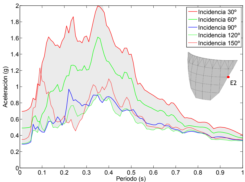
Figura 7.63. Nodo E2. Onda P+SH+SV. Embalse sin sedimentos. Espectro de aceleraciones en dirección x.
