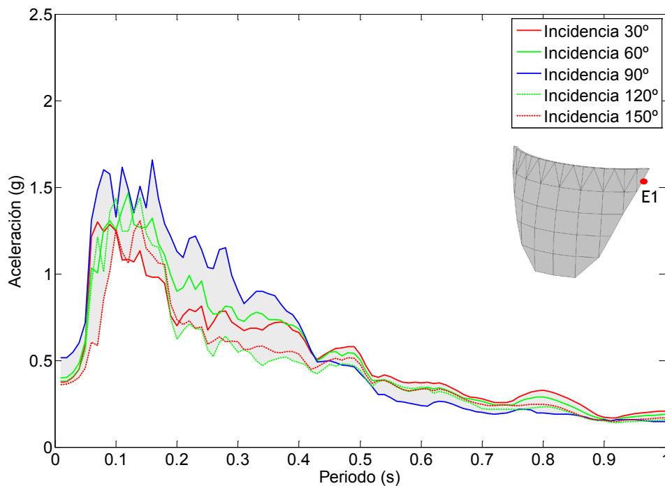
Figura 7.46. Nodo E1. Onda P+SV. Embalse sin sedimentos. Espectro de aceleraciones de campo libre en dirección z.
