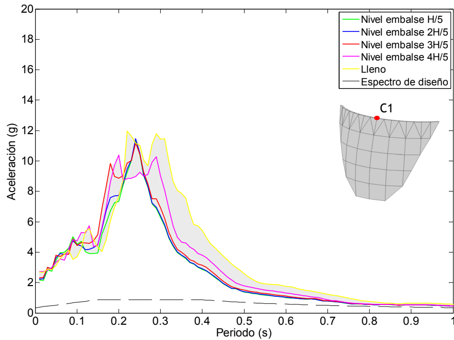
Figura 6.17. Nodo C1. Onda SH. Embalse con una capa de sedimentos de espesor H/5 . Espectro de aceleraciones en dirección x frente diferentes niveles de llenado del embalse.
