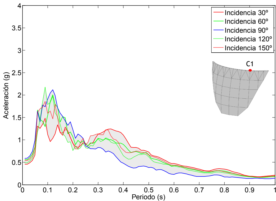
Figura 7.125. Nodo C1. Onda P+SH+SV. Embalse con una capa de sedimentos de espesor H/5 . Espectro de aceleraciones en dirección z.
