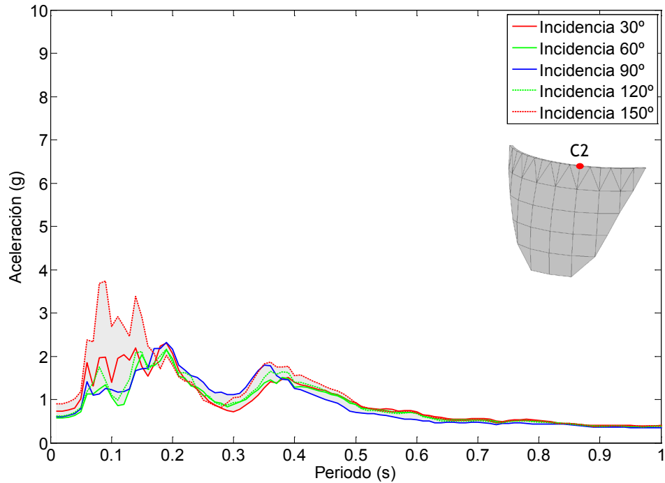
Figura 7.103. Nodo C2. Onda P+SV. Embalse sin sedimentos. Espectro de aceleraciones en dirección y.
