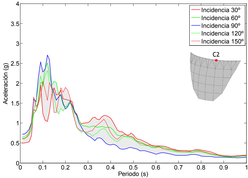
Figura 7.128. Nodo C2. Onda P+SH+SV. Embalse con una capa de sedimentos de espesor H/5 . Espectro de aceleraciones en dirección z.
