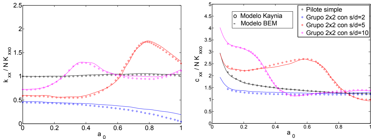
Figura 3.4. Impedancia horizontal de un pilote simple y de un grupo de pilotes 2 \times 2 en un suelo viscoelástico. Comparación con los resultados de Kaynia.
