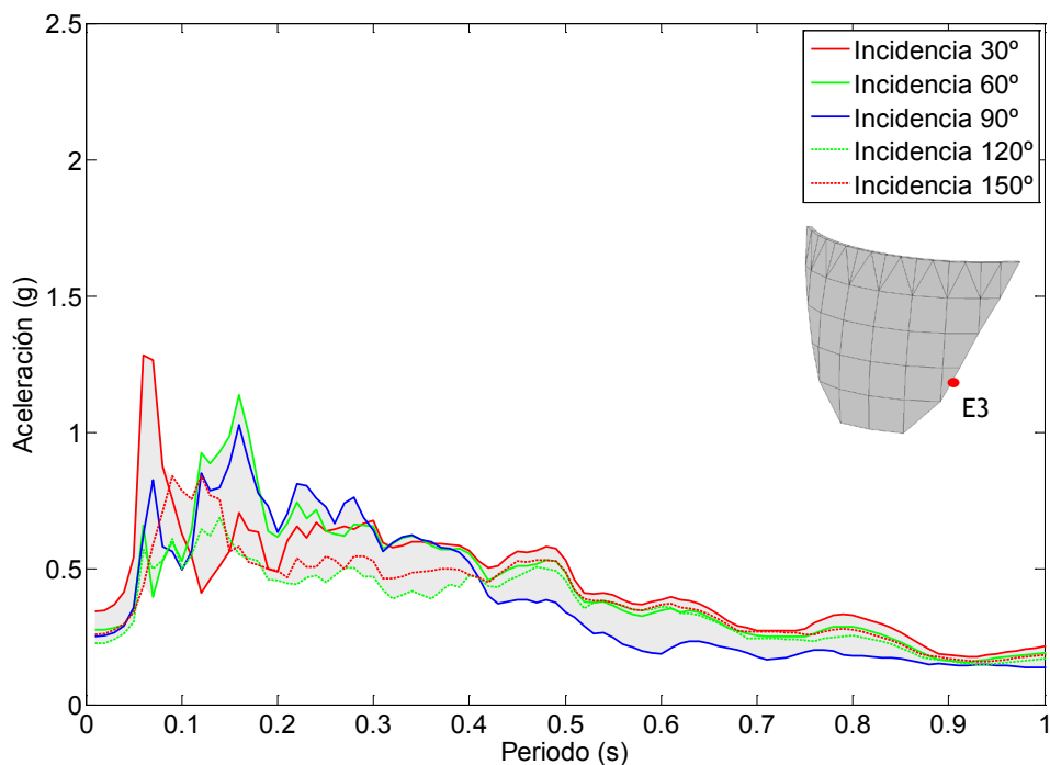
Figura 7.55. Nodo E3. Onda P+SV. Embalse sin sedimentos. Espectro de aceleraciones en dirección z.
