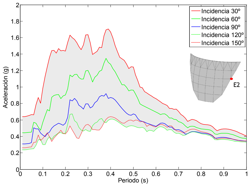
Figura 7.29. Nodo E2. Onda SH. Embalse con una capa de sedimentos de espesor 2H/5 . Espectro de aceleraciones en dirección x.
