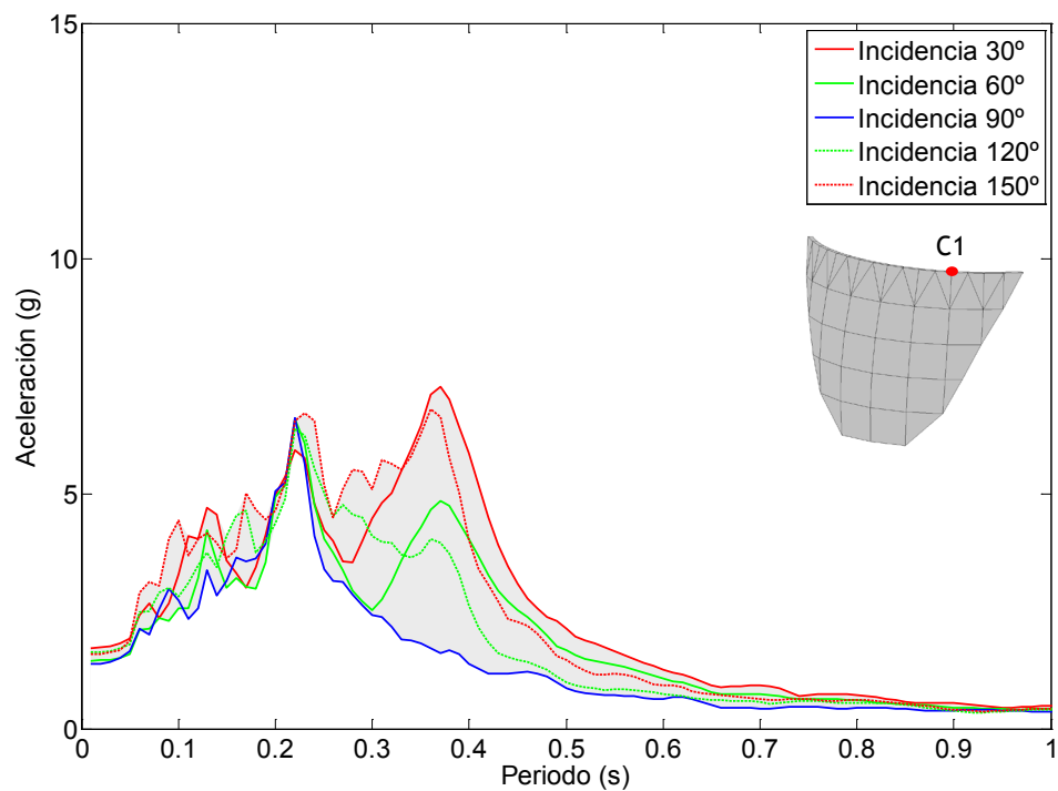
Figura 7.119. Nodo C1. Onda P+SH+SV. Embalse con una capa de sedimentos de espesor H/5 . Espectro de aceleraciones en dirección y.
