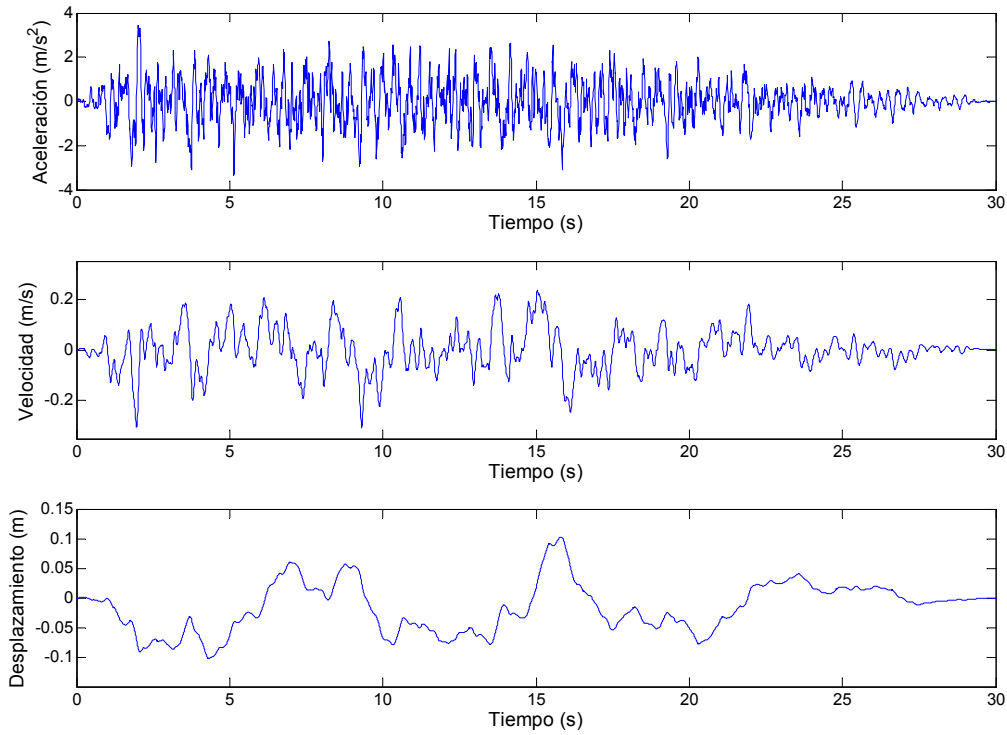
Figura 5.7. Aceleración, velocidad y desplazamiento del registro artificial corregido en dirección ‘x’.
