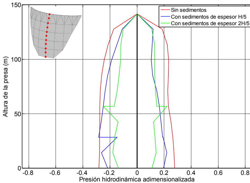
Figura 7.12. Onda SH. Incidencia 30°.
