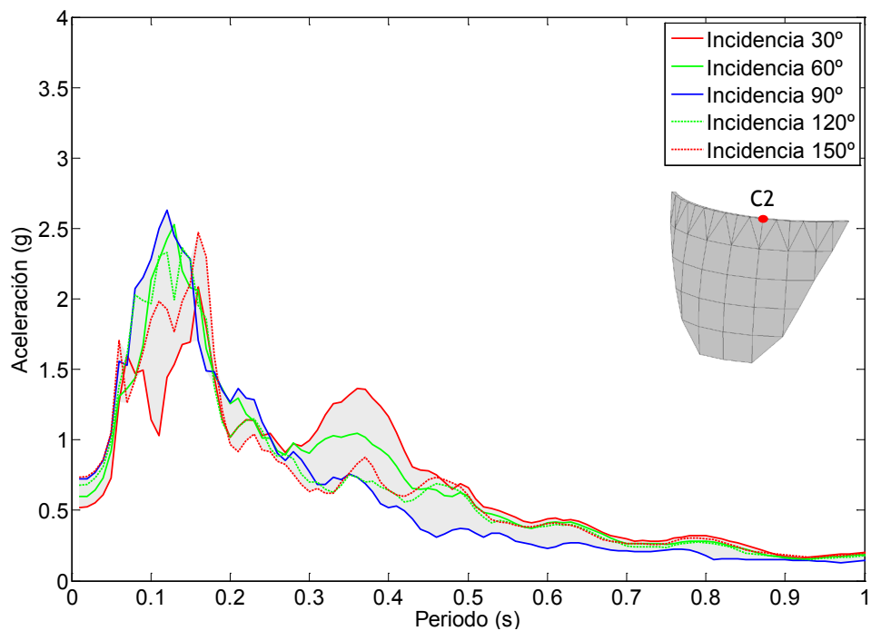
Figura 7.129. Nodo C2. Onda P+SH+SV. Embalse con una capa de sedimentos de espesor 2H/5 . Espectro de aceleraciones en dirección z.
