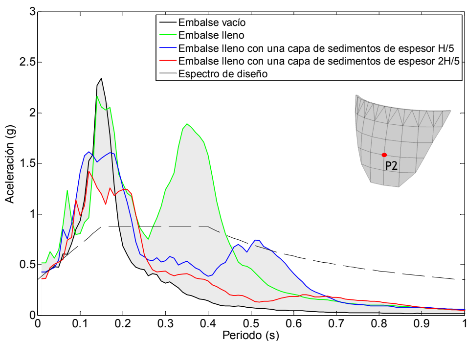
Figura 6.31. Nodo P2. Onda P. Espectro de aceleraciones en dirección x frente a diferentes condiciones del embalse.
