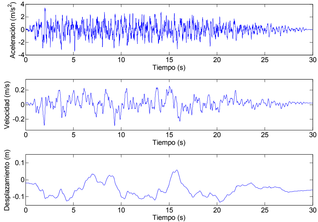
Figura 5.6. Aceleración, velocidad y desplazamiento del registro artificial en dirección 'x' antes de ser corregido.
