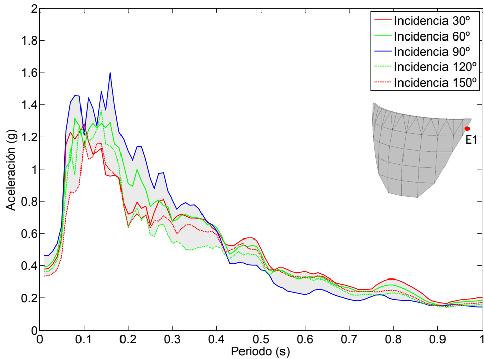
Figura 7.84. Nodo E1. Onda P+SH+SV. Embalse con una capa de sedimentos de espesor H/5 . Espectro de aceleraciones en dirección z.
