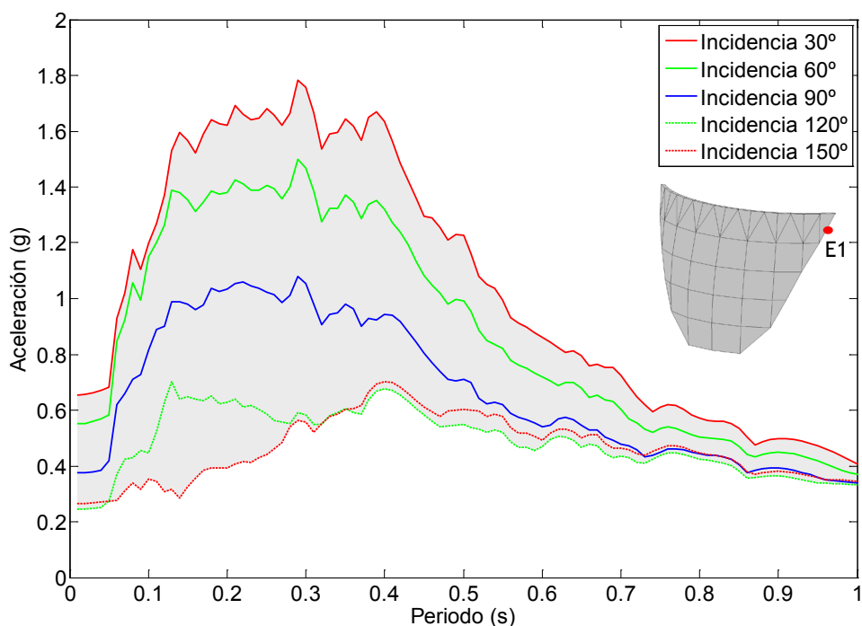
Figura 7.22. Nodo E1. Onda SH. Embalse sin sedimentos. Espectro de aceleraciones de campo libre en dirección x.
