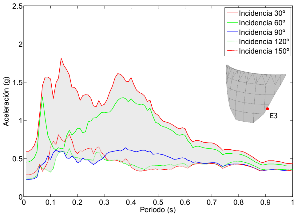
Figura 7.81. Nodo E3. Onda P+SH+SV. Embalse con una capa de sedimentos de espesor 2H/5 . Espectro de aceleraciones en dirección y.
