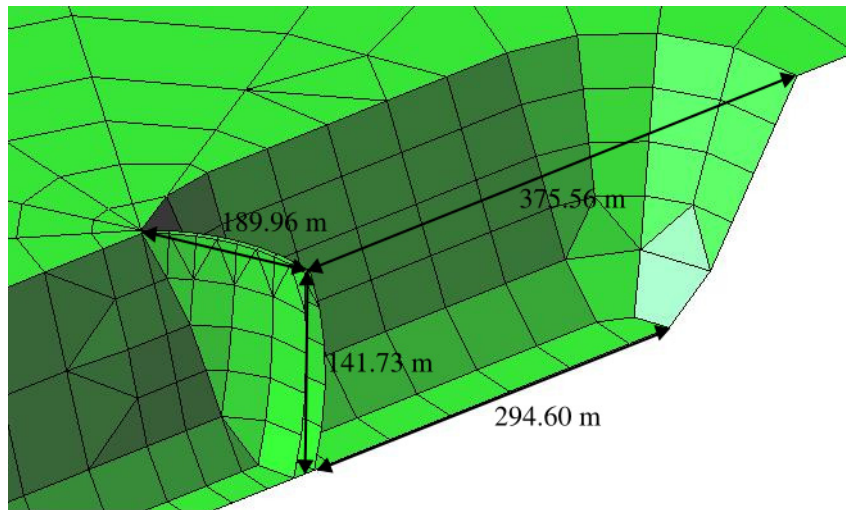
Figura 6.2. Dimensiones principales de la discretización del embalse y la presa.
