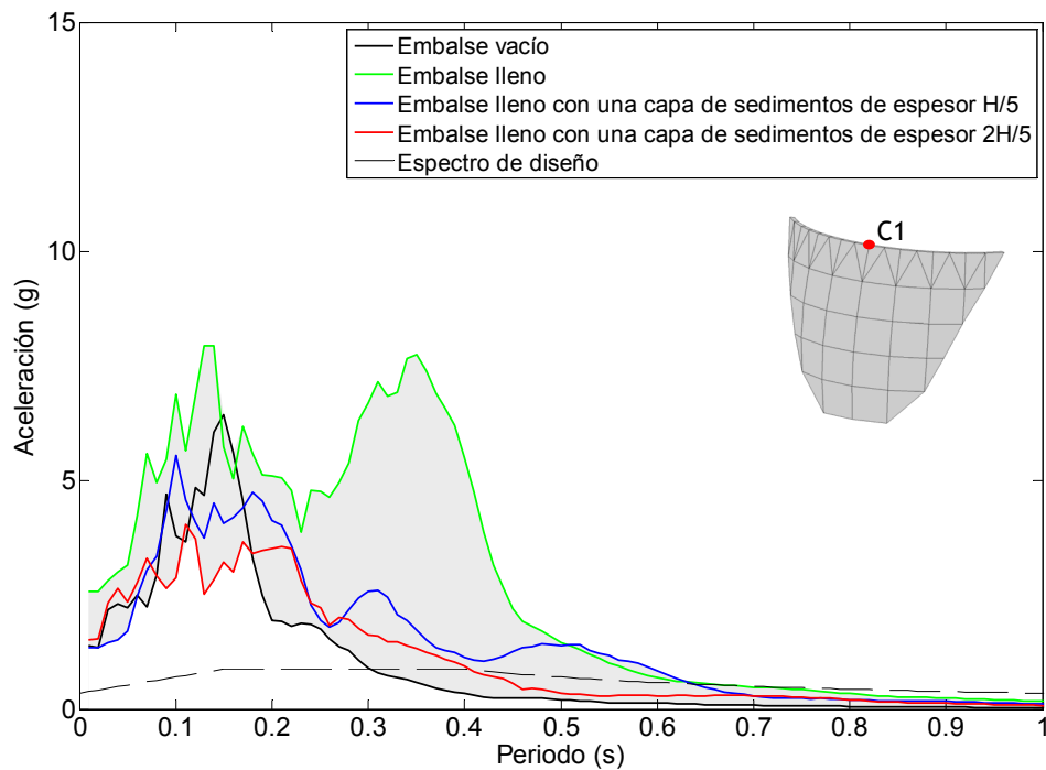
Figura 6.39. Nodo C1. Onda P. Espectro de aceleraciones en dirección x frente a diferentes condiciones del embalse.
