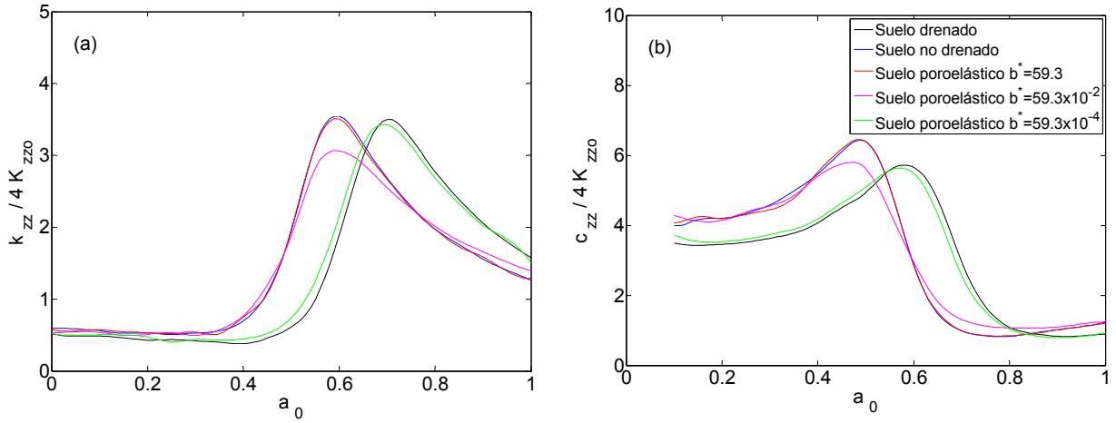
Figura 3.11. Influencia de la permabilidad del suelo. Impedancia vertical. Grupo de pilotes 2 x 2 con s/d = 5 .
