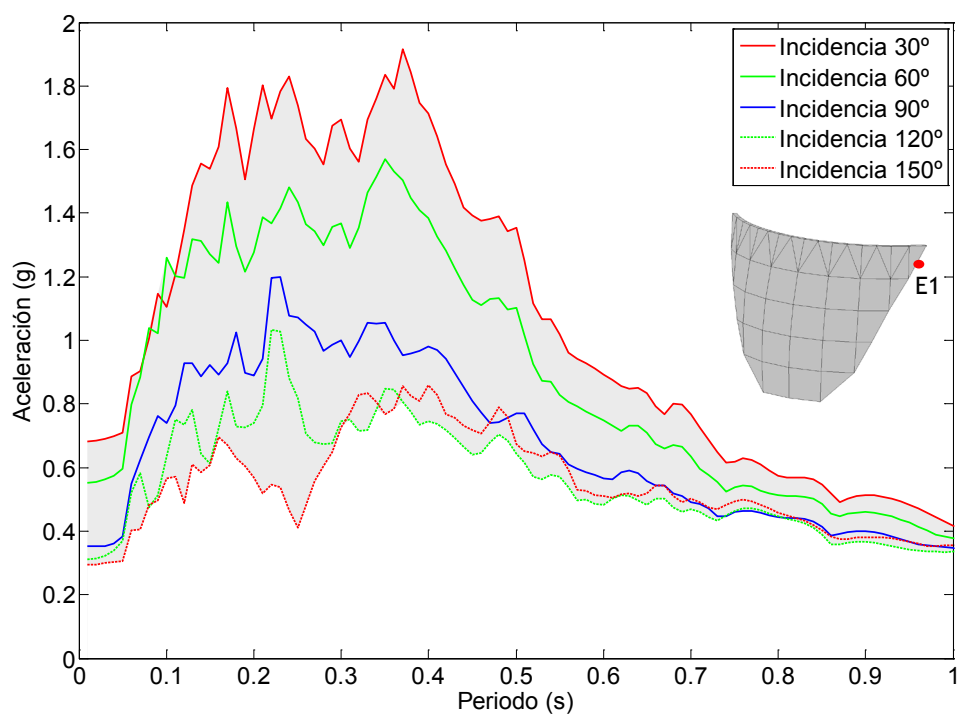
Figura 7.59. Nodo E1. Onda P+SH+SV. Embalse sin sedimentos. Espectro de aceleraciones en dirección x.
