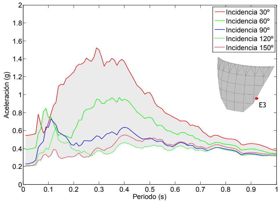
Figura 7.30. Nodo E3. Onda SH. Embalse sin sedimentos. Espectro de aceleraciones de campo libre en dirección x.
