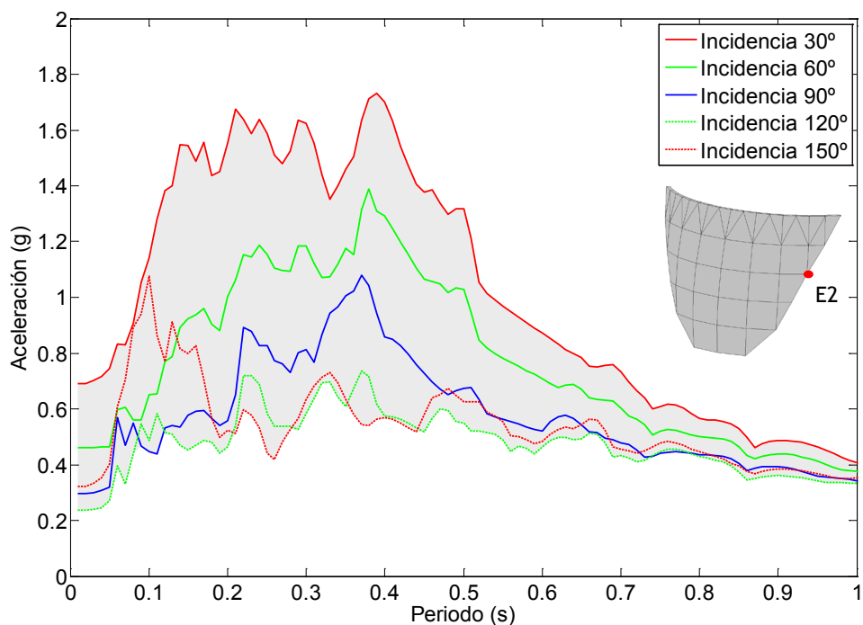
Figura 7.65. Nodo E2. Onda P+SH+SV. Embalse con una capa de sedimentos de espesor 2H/5 . Espectro de aceleraciones en dirección x.
