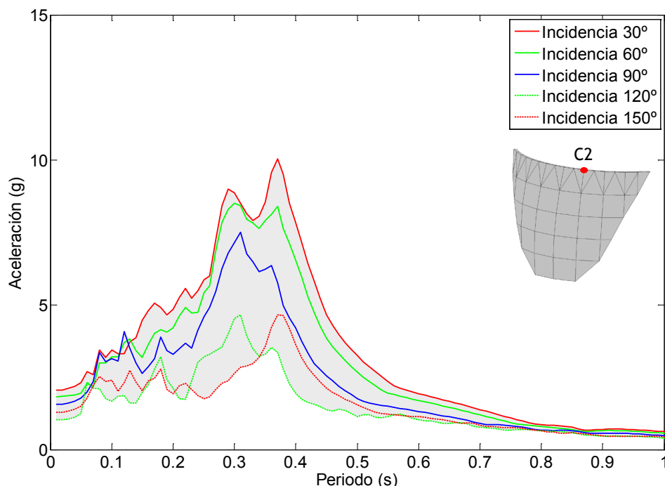
Figura 7.99. Nodo C2. Onda SH. Embalse con una capa de sedimentos de espesor 2H/5 . Espectro de aceleraciones en dirección x.
