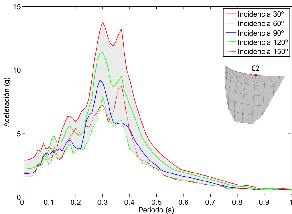
Figura 7.97. Nodo C2. Onda SH. Embalse sin sedimentos. Espectro de aceleraciones en dirección x.
