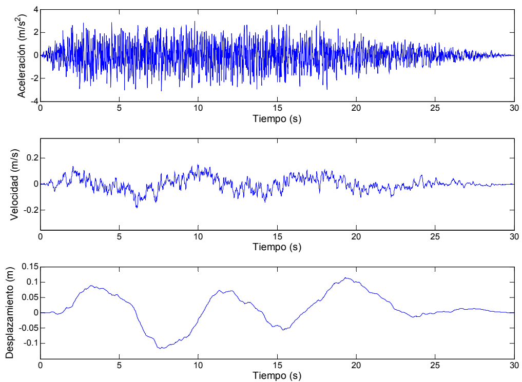
Figura 5.9. Aceleración, velocidad y desplazamiento del registro artificial corregido en dirección 'z'.
