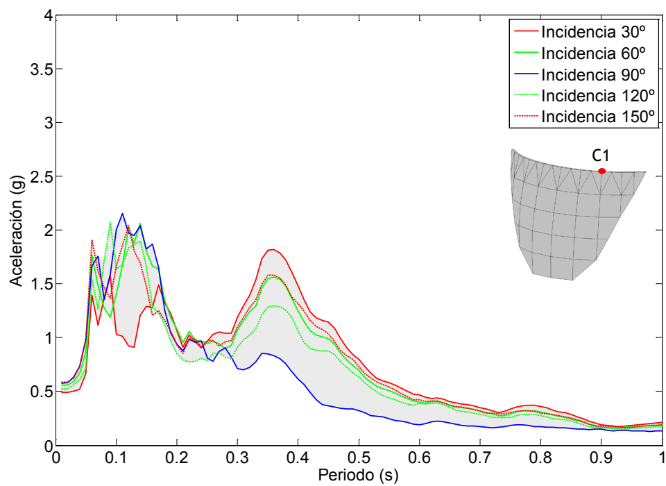
Figura 7.106. Nodo C1. Onda P+SV. Embalse sin sedimentos. Espectro de aceleraciones en dirección z.
