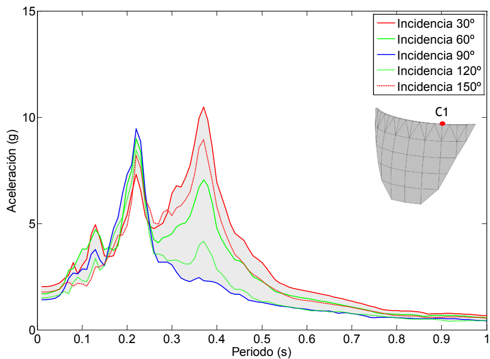
Figura 7.95. Nodo C1. Onda SH. Embalse con una capa de sedimentos de espesor H/5 . Espectro de aceleraciones en dirección x.
