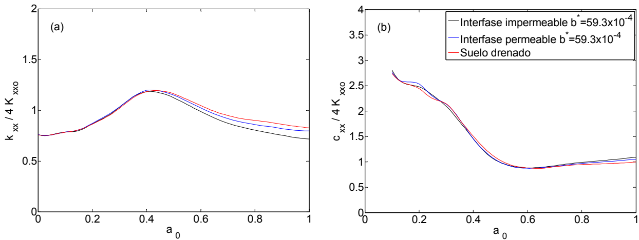
Figura 3.15. Influencia de la condición de contorno hidráulica a lo largo de la interfase pilote-suelo. Impedancia horizontal de un grupo de pilotes 2 x 2 con s/d = 10 y b^* = 59.3 \times 10^{-4} .
