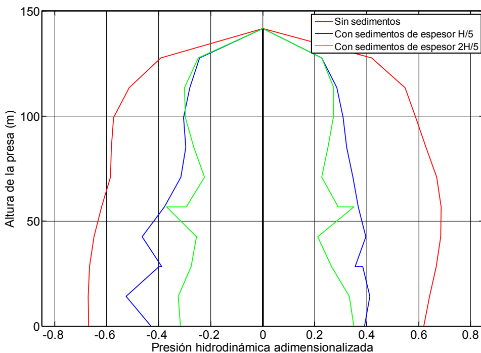
Figura 7.18. Onda P+SH+SV. Incidencia 30°.
