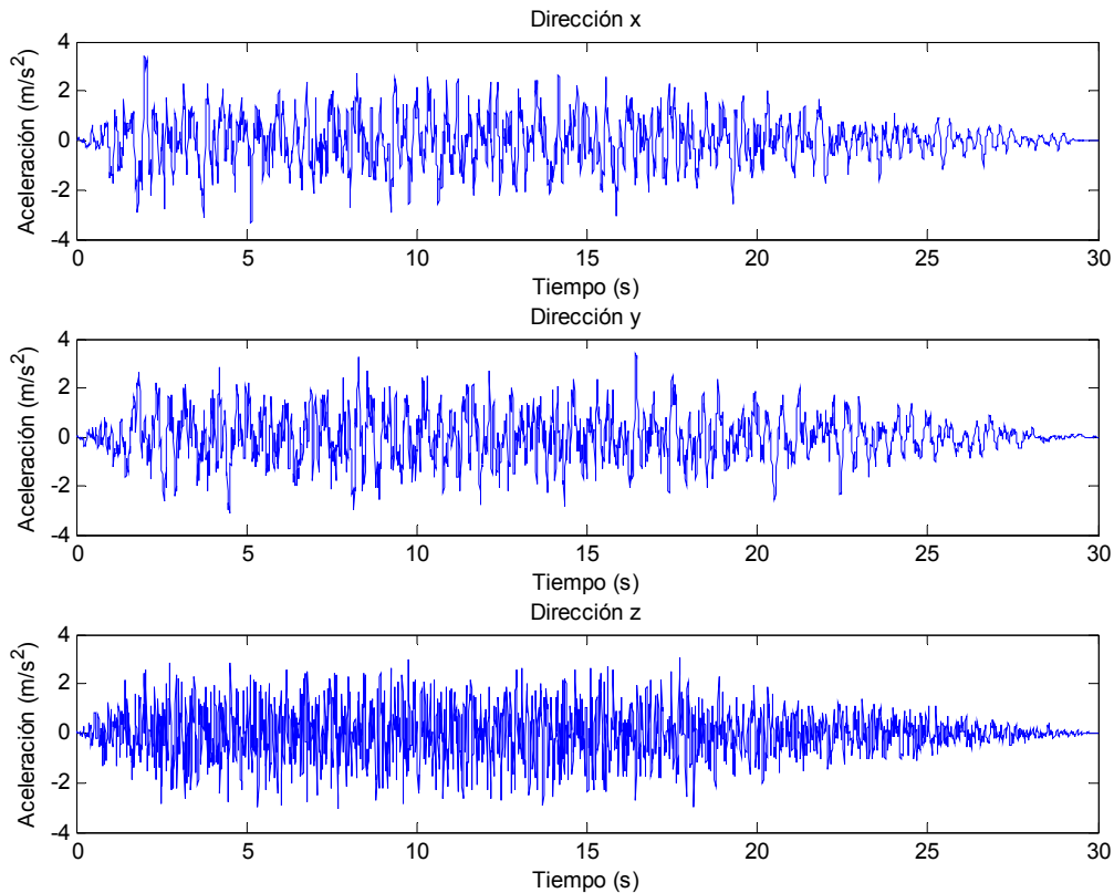
Figura 5.5. Acelerogramas artificiales generados.
