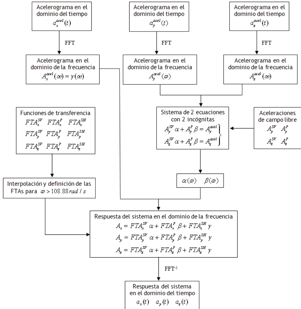
Figura 5.15. Esquema resumen del procedimiento seguido para la obtención de la respuesta del sistema en términos de la evolución temporal de las aceleraciones.
