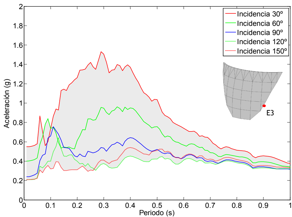
Figura 7.66. Nodo E3. Onda P+SH+SV. Embalse sin sedimentos. Espectro de aceleraciones de campo libre en dirección x.
