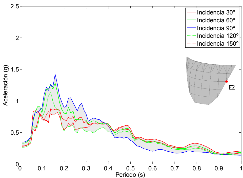
Figura 7.53. Nodo E2. Onda P+SV. Embalse con una capa de sedimentos de espesor 2H/5 . Espectro de aceleraciones en dirección z.
