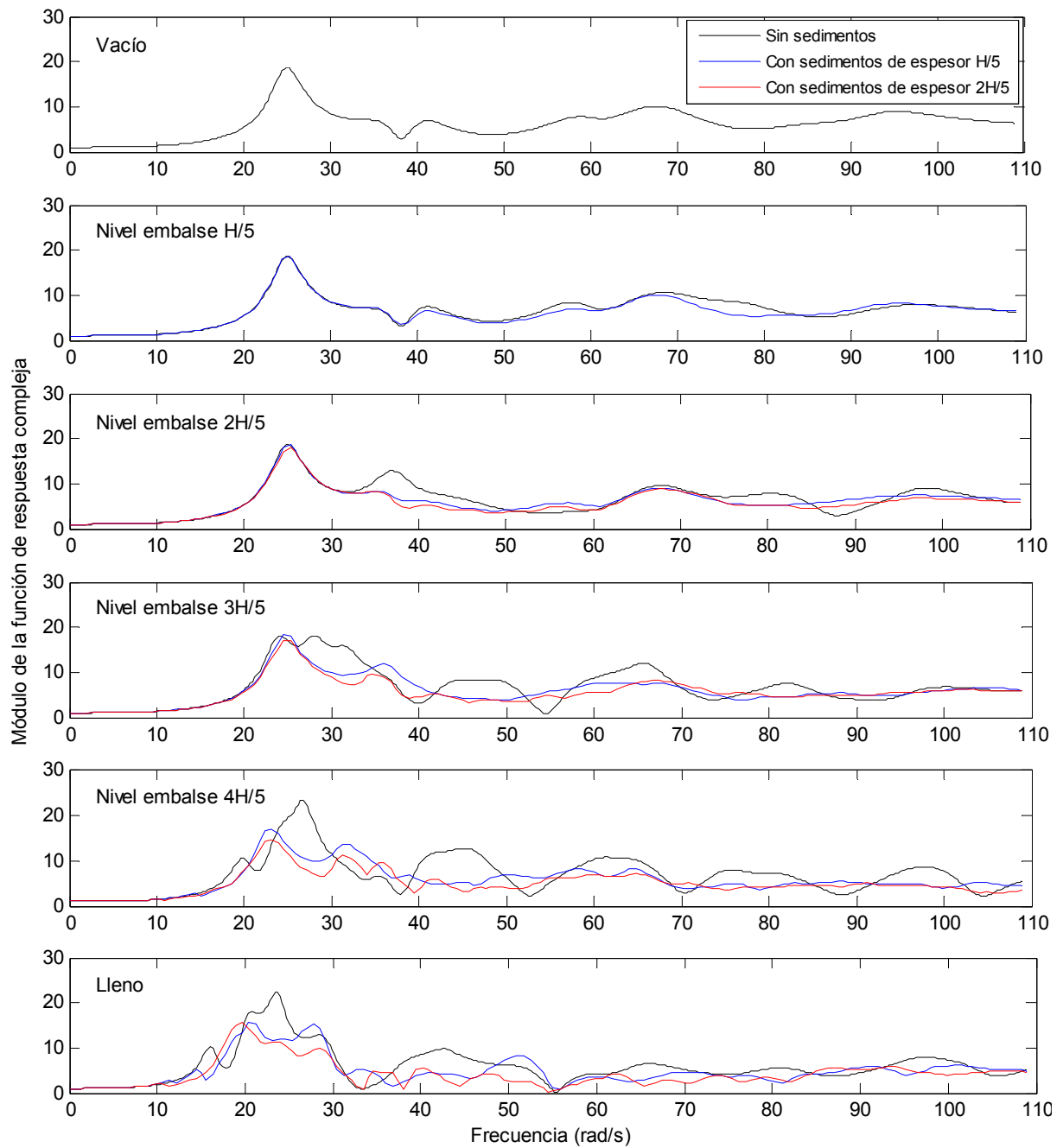
Figura 6.8. Módulo de la función de respuesta compleja en dirección x. Nodo C1. Onda SH con incidencia vertical.
