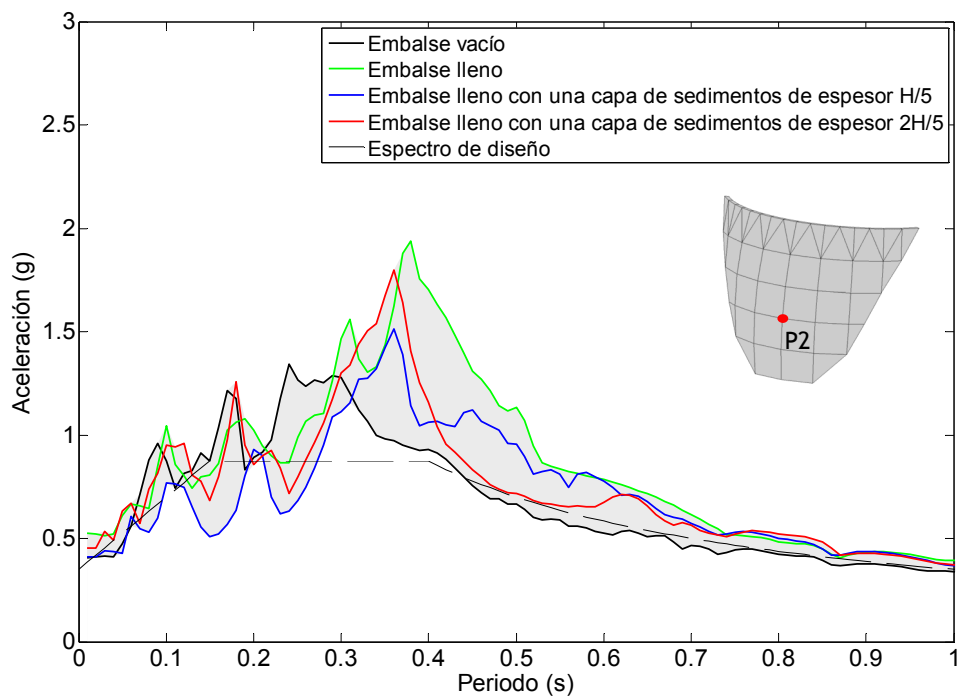
Figura 6.33. Nodo P2. Onda SH. Espectro de aceleraciones en dirección x frente a diferentes condiciones del embalse.
