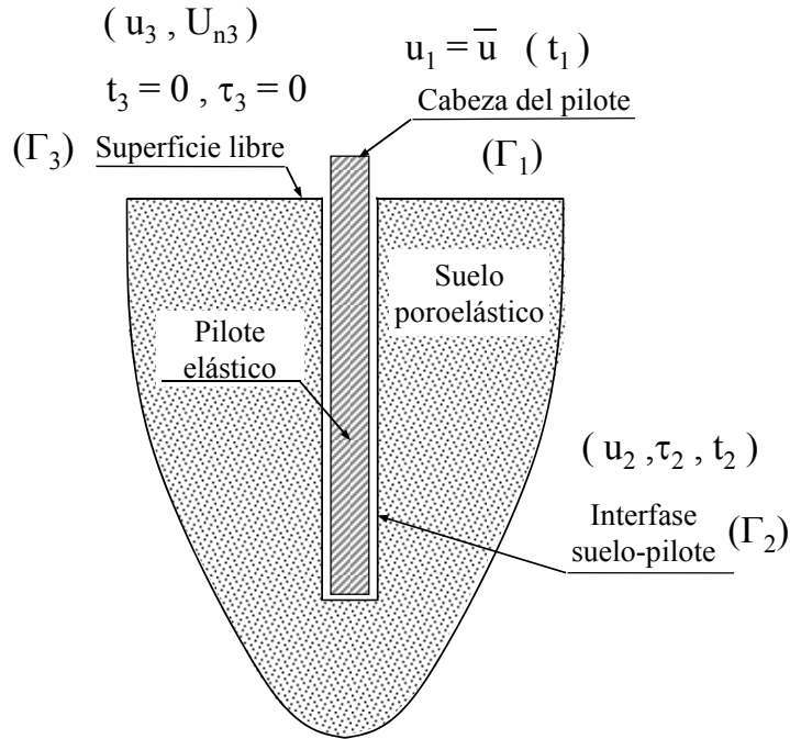
Figura 3.1. Pilote simple impermeable embebido en un semi-espacio poroelástico. Condiciones de contorno y valores desconocidos en las ecuaciones acopladas del problema.
