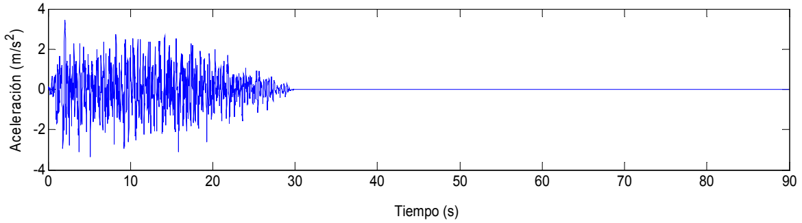
Figura 5.11. Acelerograma modificado antes de calcular su FFT.
