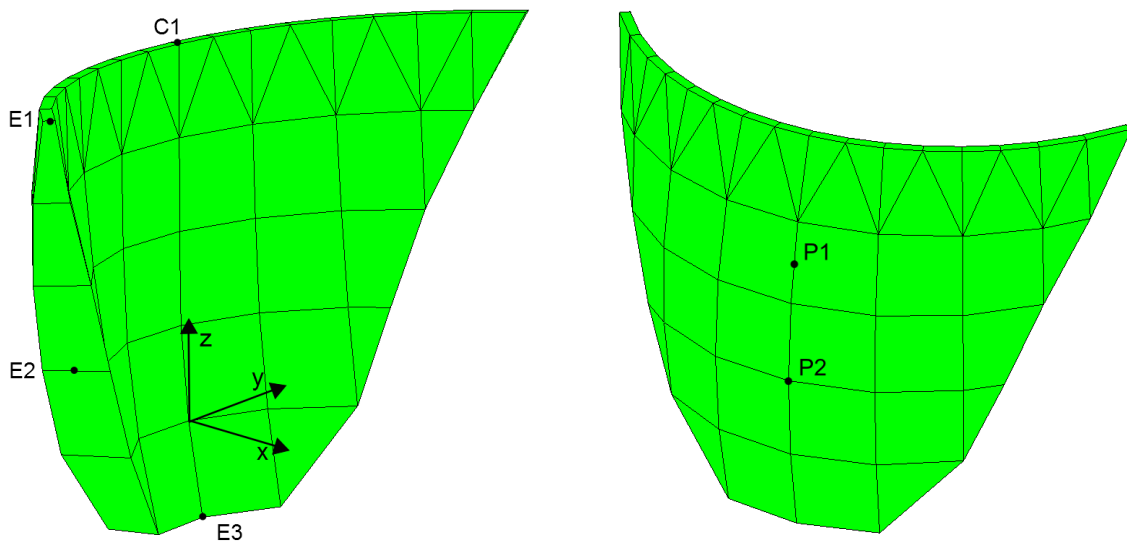
Figura 6.6. Puntos de la presa donde se presentan los resultados.
