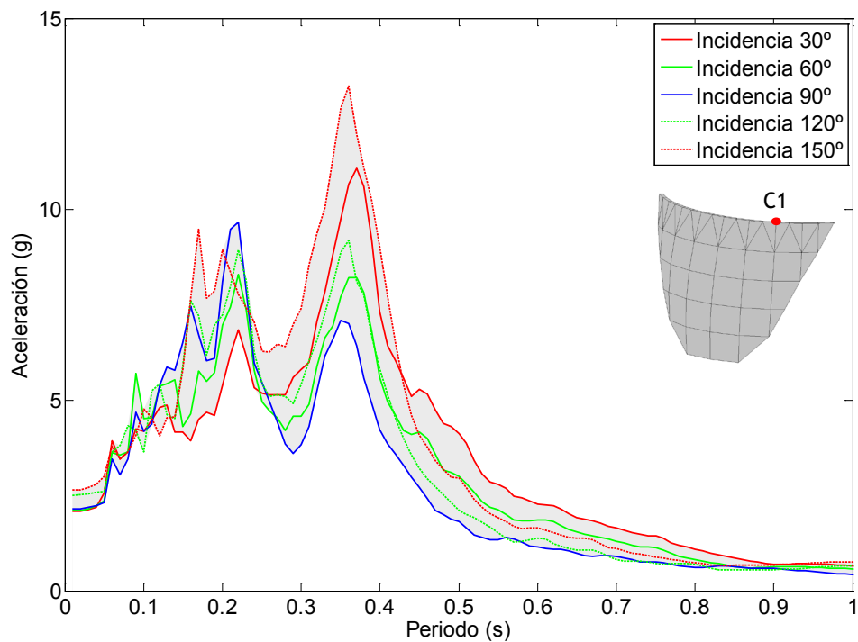
Figura 7.114. Nodo C1. Onda P+SH+SV. Embalse con una capa de sedimentos de espesor 2H/5 . Espectro de aceleraciones en dirección x.
