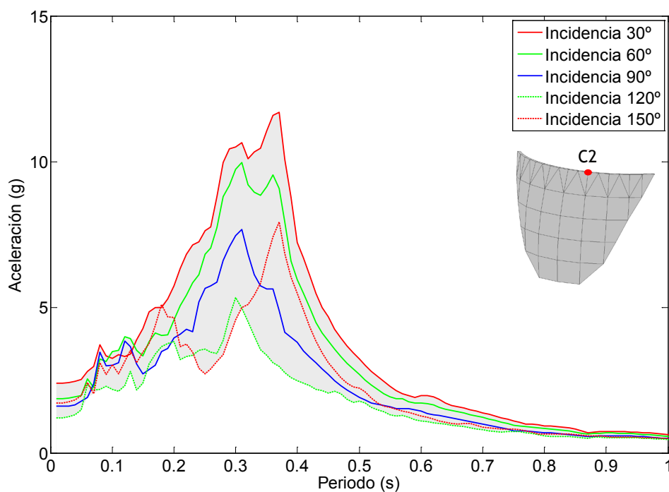
Figura 7.98. Nodo C2. Onda SH. Embalse con una capa de sedimentos de espesor H/5 . Espectro de aceleraciones en dirección x.
