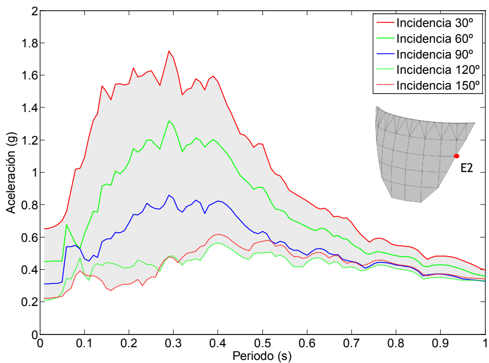
Figura 7.62. Nodo E2. Onda P+SH+SV. Embalse sin sedimentos. Espectro de aceleraciones de campo libre en dirección x.
