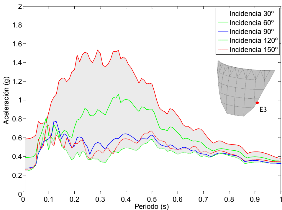
Figura 7.68. Nodo E3. Onda P+SH+SV. Embalse con una capa de sedimentos de espesor H/5 . Espectro de aceleraciones en dirección x.
