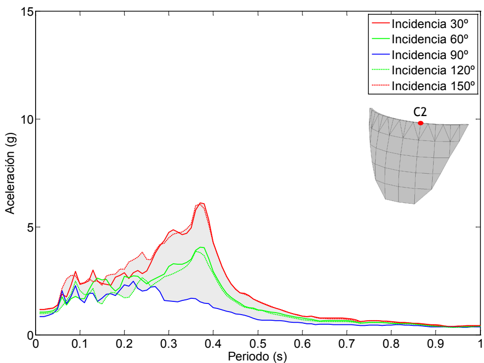
Figura 7.122. Nodo C2. Onda P+SH+SV. Embalse con una capa de sedimentos de espesor H/5 . Espectro de aceleraciones en dirección y.
