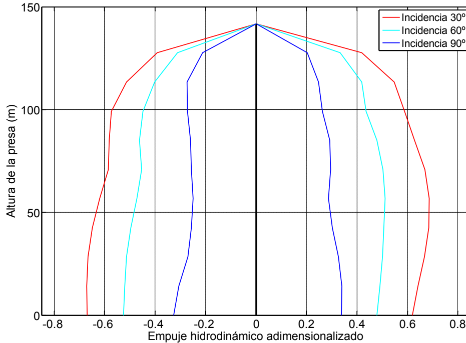
Figura 7.9. Onda P+SH+SV. Embalse lleno de agua sin sedimentos.
