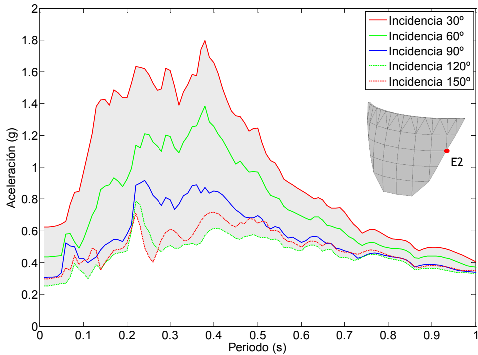
Figura 7.28. Nodo E2. Onda SH. Embalse con una capa de sedimentos de espesor H/5 . Espectro de aceleraciones en dirección x.
