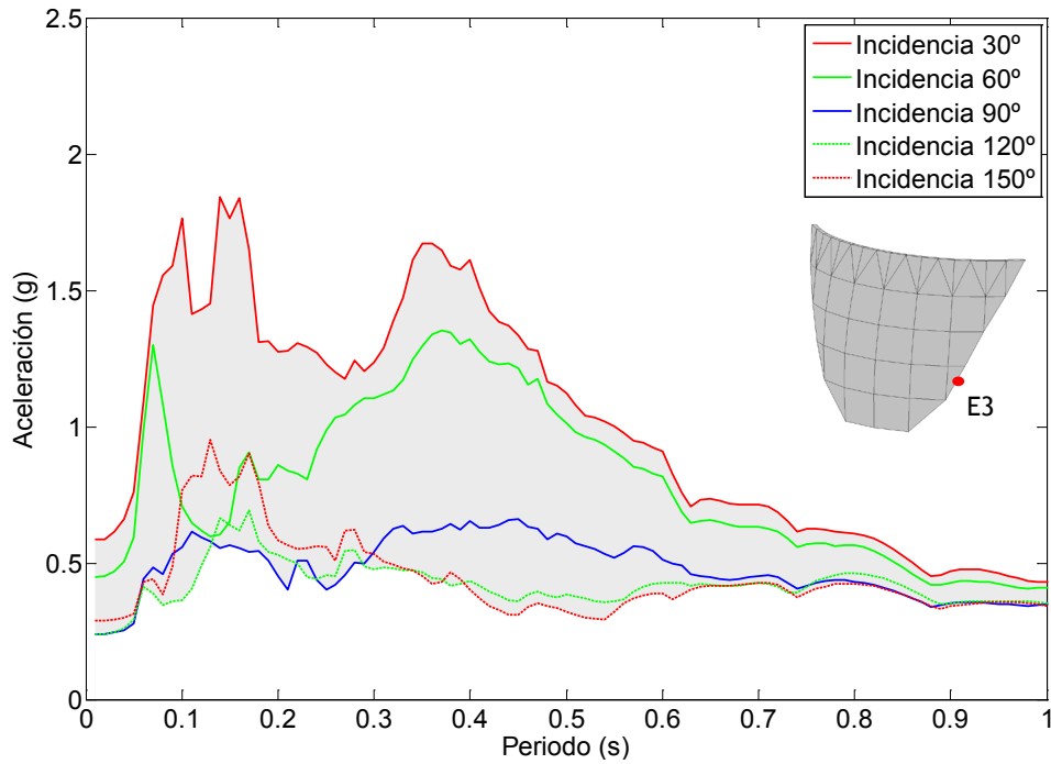
Figura 7.80. Nodo E3. Onda P+SH+SV. Embalse con una capa de sedimentos de espesor H/5 . Espectro de aceleraciones en dirección y.
