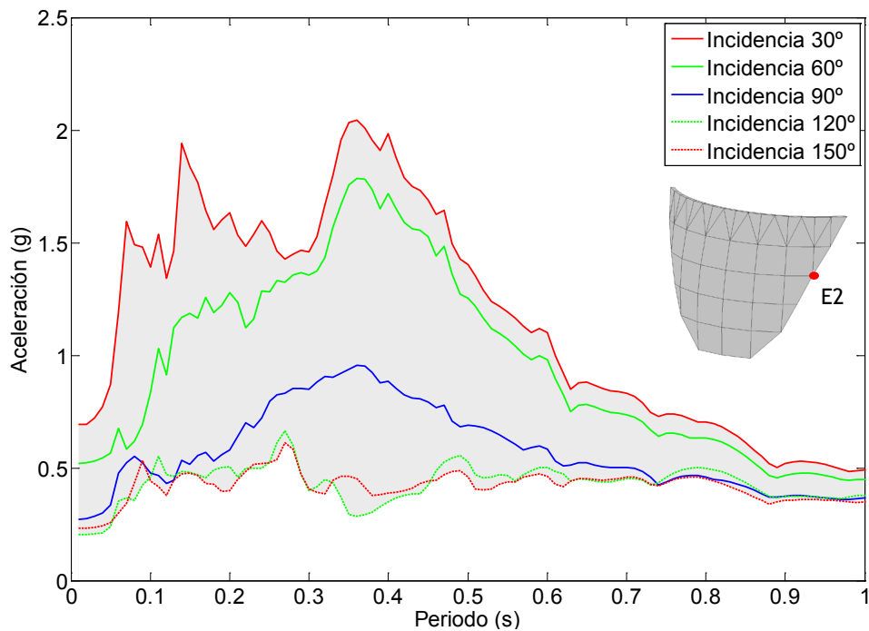
Figura 7.41. Nodo E2. Onda P+SV. Embalse con una capa de sedimentos de espesor 2H/5 . Espectro de aceleraciones en dirección y.
