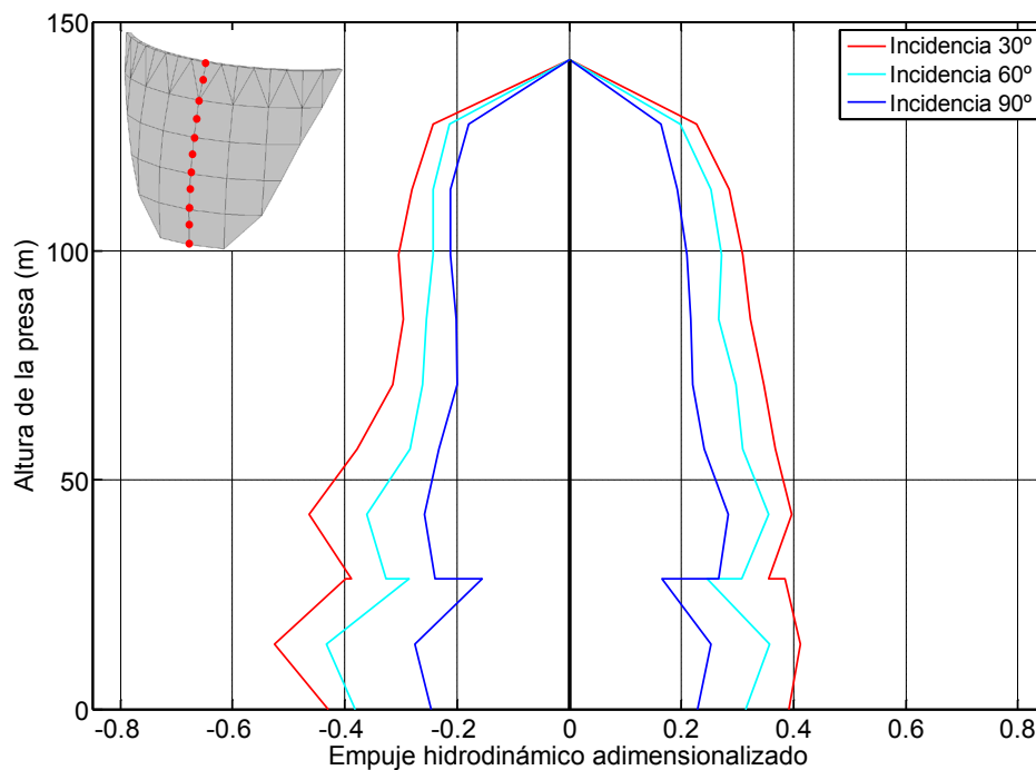
Figura 7.10. Onda P+SH+SV. Embalse lleno de agua con una capa de sedimentos de espesor H/5 .
