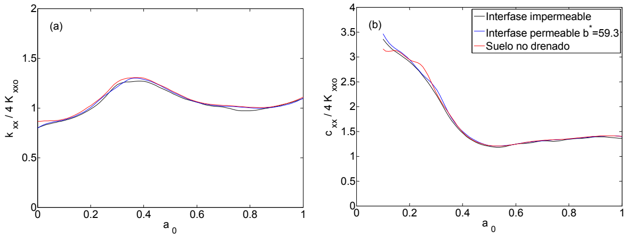
Figura 3.14. Influencia de la condición de contorno hidráulica a lo largo de la interfase pilote-suelo. Impedancia horizontal de un grupo de pilotes 2 x 2 con s/d = 10 y b^* = 59.3 .
