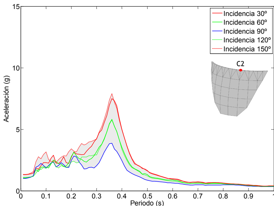
Figura 7.123. Nodo C2. Onda P+SH+SV. Embalse con una capa de sedimentos de espesor 2H/5 . Espectro de aceleraciones en dirección y.
