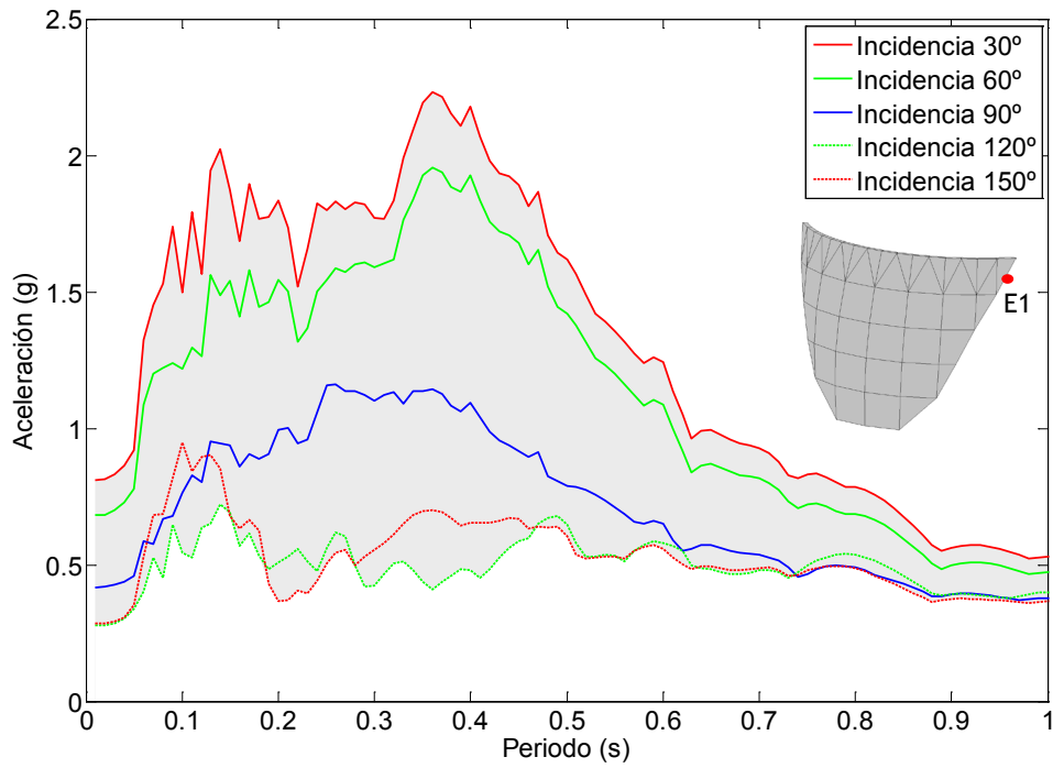
Figura 7.37. Nodo E1. Onda P+SV. Embalse con una capa de sedimentos de espesor 2H/5 . Espectro de aceleraciones en dirección y.
