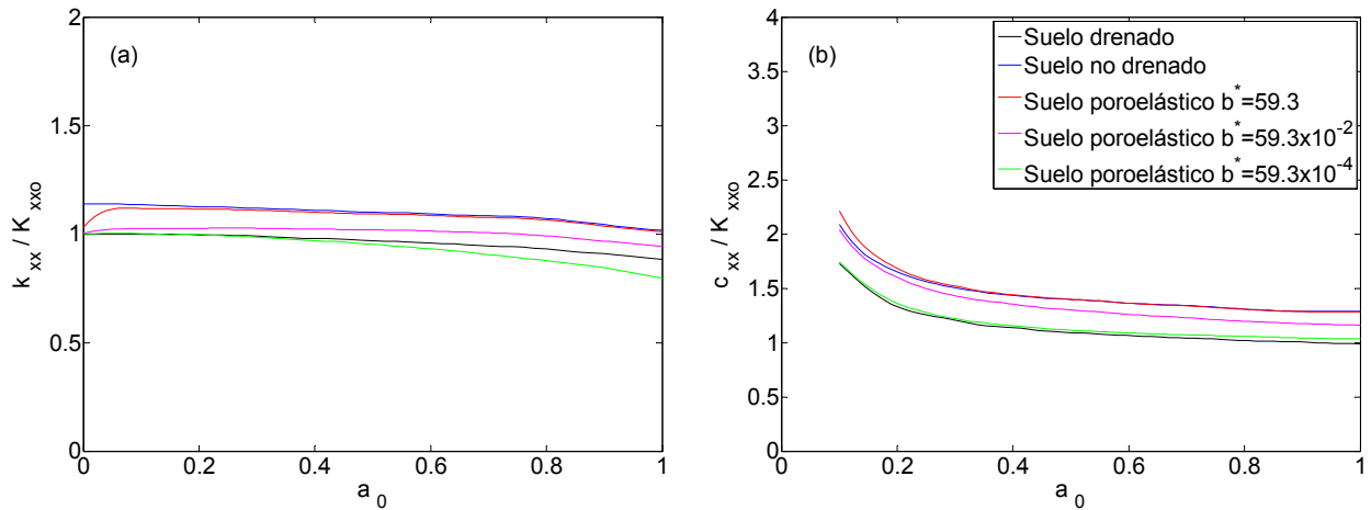
Figura 3.8. Influencia de la permeabilidad del suelo. Impedancia horizontal. Pilote simple.
