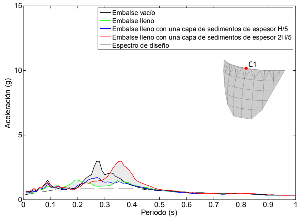
Figura 6.42. Nodo C1. Onda SV. Espectro de aceleraciones en dirección y frente a diferentes condiciones del embalse.
