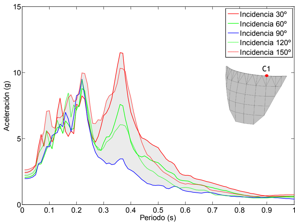
Figura 7.112. Nodo C1. Onda P+SH+SV. Embalse sin sedimentos. Espectro de aceleraciones en dirección x.
