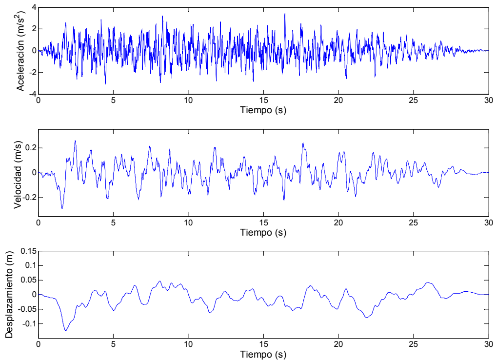
Figura 5.8. Aceleración, velocidad y desplazamiento del registro artificial corregido en dirección 'y'.
