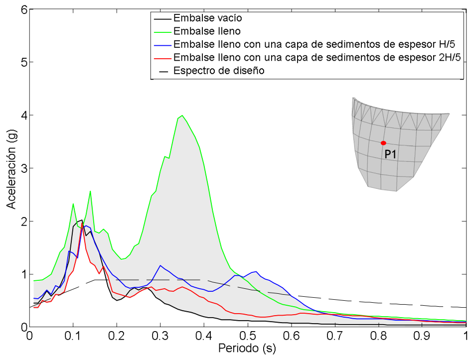
Figura 6.35. Nodo P1. Onda P. Espectro de aceleraciones en dirección x frente a diferentes condiciones del embalse.
