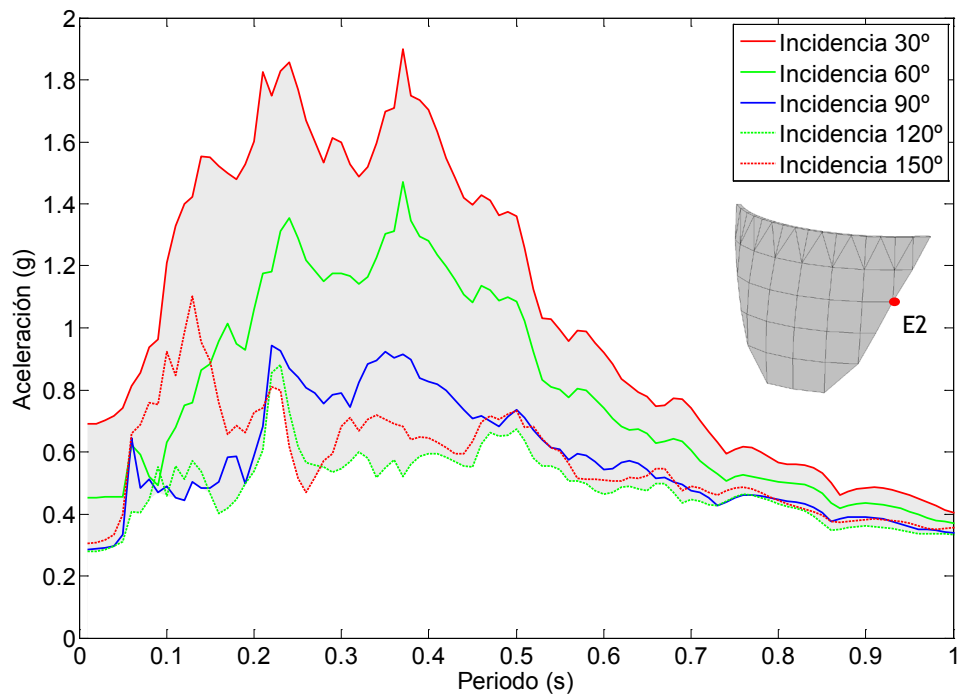
Figura 7.64. Nodo E2. Onda P+SH+SV. Embalse con una capa de sedimentos de espesor H/5 . Espectro de aceleraciones en dirección x.
