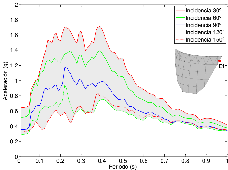
Figura 7.23. Nodo E1. Onda SH. Embalse sin sedimentos. Espectro de aceleraciones en dirección x.
