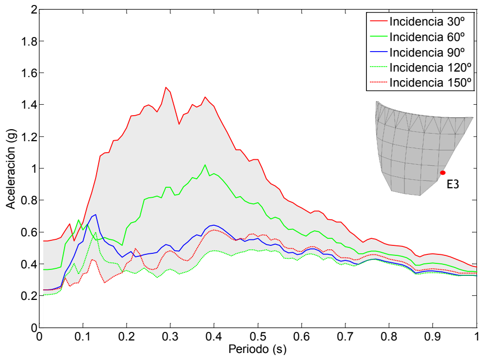
Figura 7.32. Nodo E3. Onda SH. Embalse con una capa de sedimentos de espesor H/5 . Espectro de aceleraciones en dirección x.
