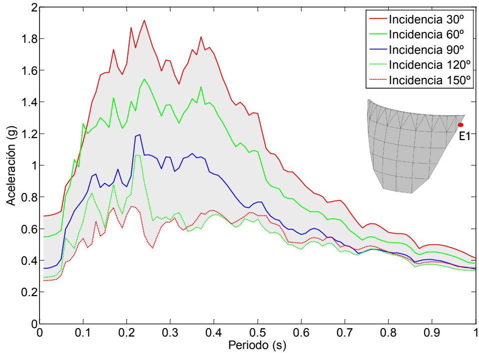
Figura 7.60. Nodo E1. Onda P+SH+SV. Embalse con una capa de sedimentos de espesor H/5 . Espectro de aceleraciones en dirección x.
