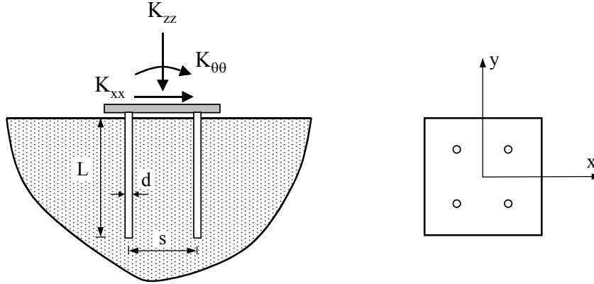
Figura 3.2. Grupo de pilotes 2x2 embebidos en un semi-espacio. Definición de la geometría del problema.
