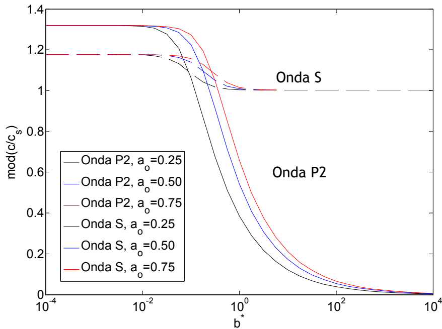
Figura 3.7. Amplitudes de las velocidades de propagación de las ondas en el suelo poroelástico frente a la constante de disipación.
