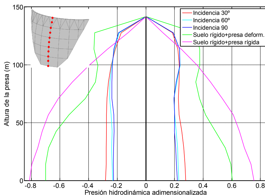
Figura 7.3. Onda SH. Embalse lleno de agua sin sedimentos.
