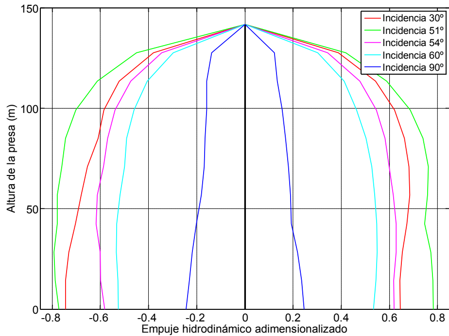
Figura 7.6. Onda P+SV. Embalse lleno de agua sin sedimentos.
