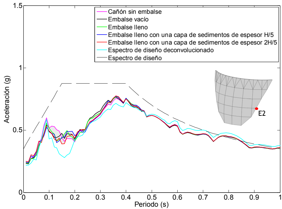
Figura 6.26. Nodo E2. Onda SV. Espectro de aceleraciones en dirección y frente a diferentes condiciones del embalse.
