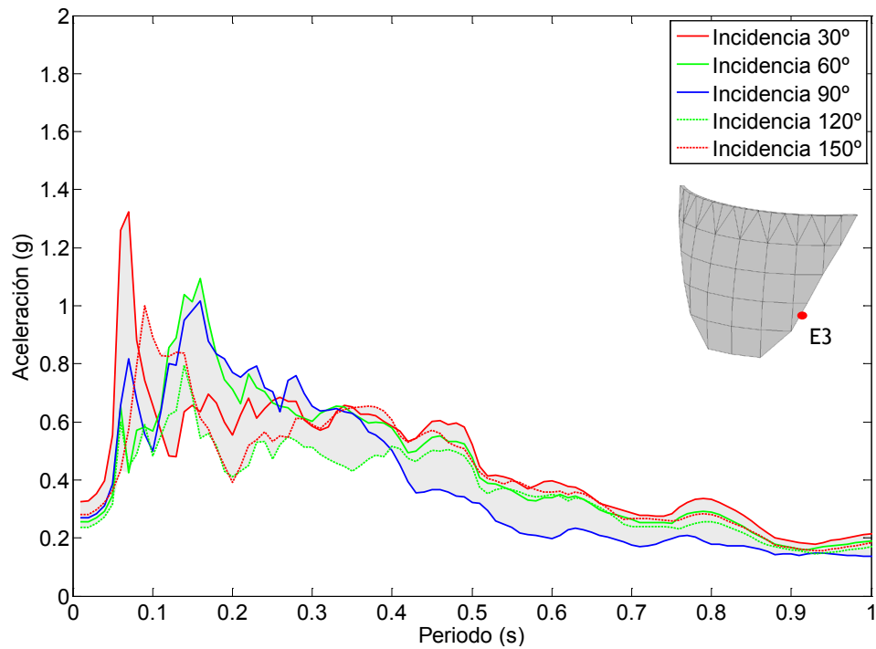
Figura 7.92. Nodo E3. Onda P+SH+SV. Embalse con una capa de sedimentos de espesor H/5 . Espectro de aceleraciones en dirección z.
