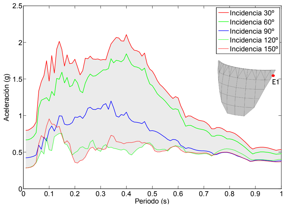
Figura 7.73. Nodo E1. Onda P+SH+SV. Embalse con una capa de sedimentos de espesor 2H/5 . Espectro de aceleraciones en dirección y.
