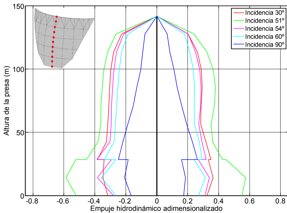
Figura 7.7. Onda P+SV. Embalse lleno de agua con una capa de sedimentos de espesor H/5 .
