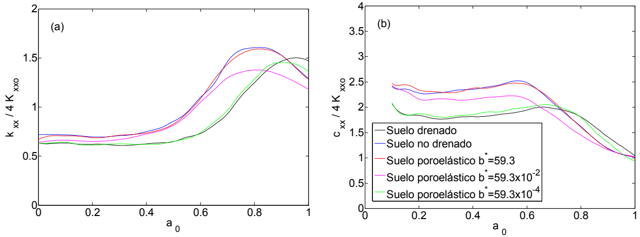
Figura 3.10. Influencia de la permabilidad del suelo. Impedancia horizontal. Grupo de pilotes 2 x 2 con s/d = 5 .
