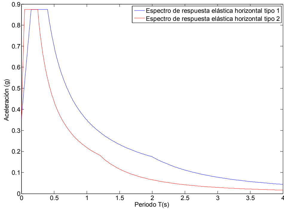
Figura 5.2. Comparativa entre los espectros de respuesta elástica horizontal tipo 1 y tipo 2 para una aceleración de diseño de 0.35g.
