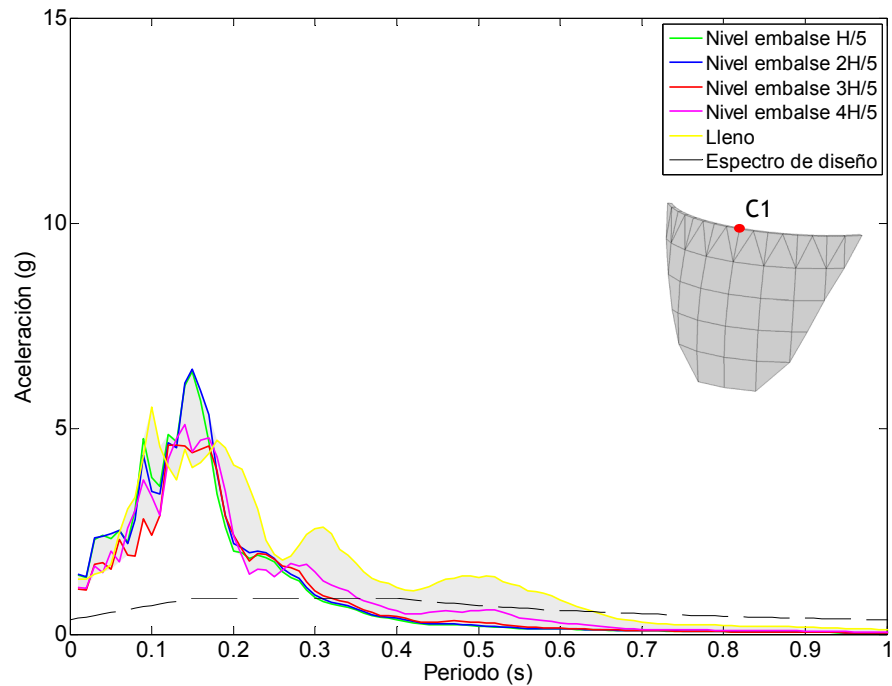
Figura 6.14. Nodo C1. Onda P. Embalse con una capa de sedimentos de espesor H/5 . Espectro de aceleraciones en dirección x frente diferentes niveles de llenado del embalse.
