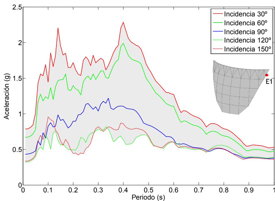
Figura 7.71. Nodo E1. Onda P+SH+SV. Embalse sin sedimentos. Espectro de aceleraciones en dirección y.
