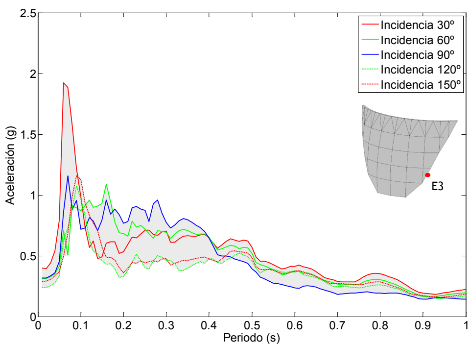
Figura 7.54. Nodo E3. Onda P+SV. Embalse sin sedimentos. Espectro de aceleraciones de campo libre en dirección z.
