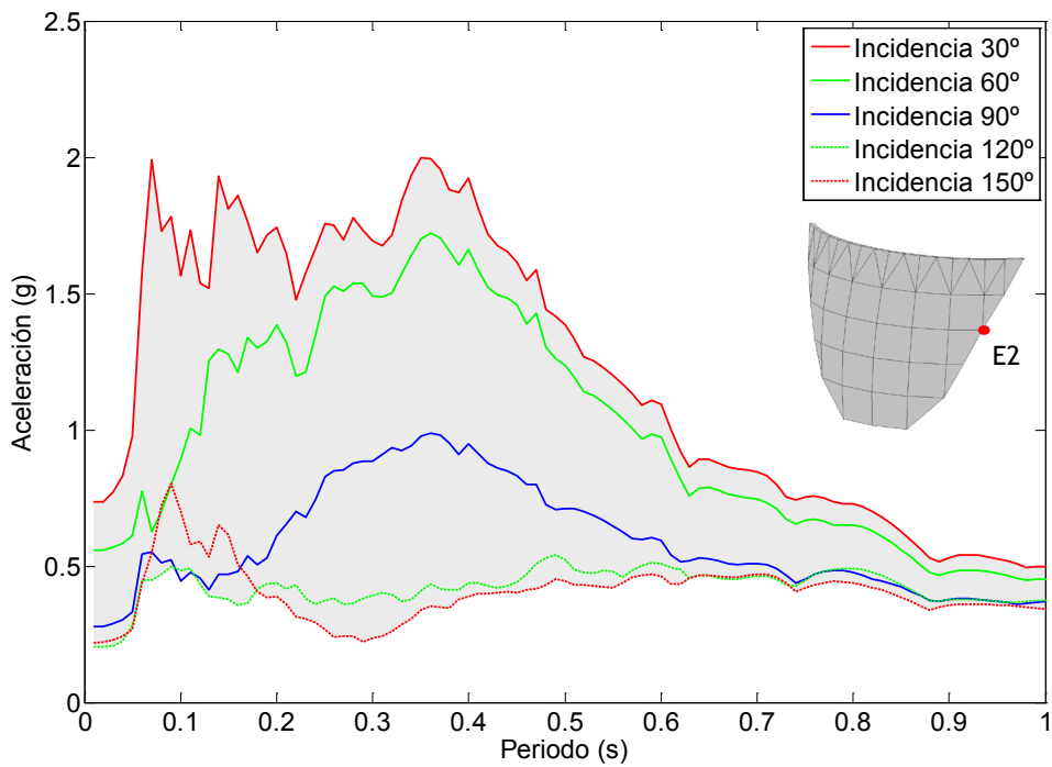
Figura 7.38. Nodo E2. Onda P+SV. Embalse sin sedimentos. Espectro de aceleraciones de campo libre en dirección y.
