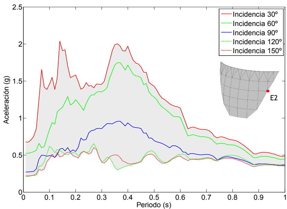
Figura 7.40. Nodo E2. Onda P+SV. Embalse con una capa de sedimentos de espesor H/5 . Espectro de aceleraciones en dirección y.
