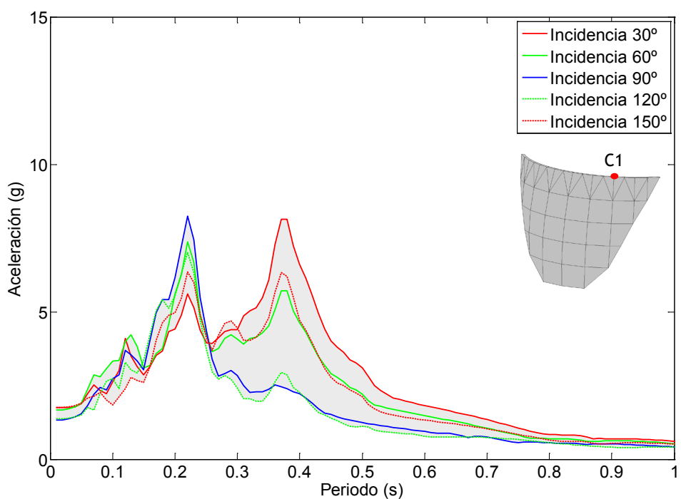
Figura 7.96. Nodo C1. Onda SH. Embalse con una capa de sedimentos de espesor 2H/5 . Espectro de aceleraciones en dirección x.
