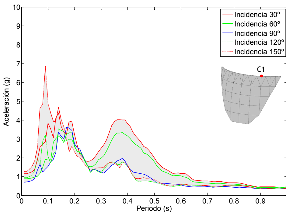
Figura 7.100. Nodo C1. Onda P+SV. Embalse sin sedimentos. Espectro de aceleraciones en dirección y.
