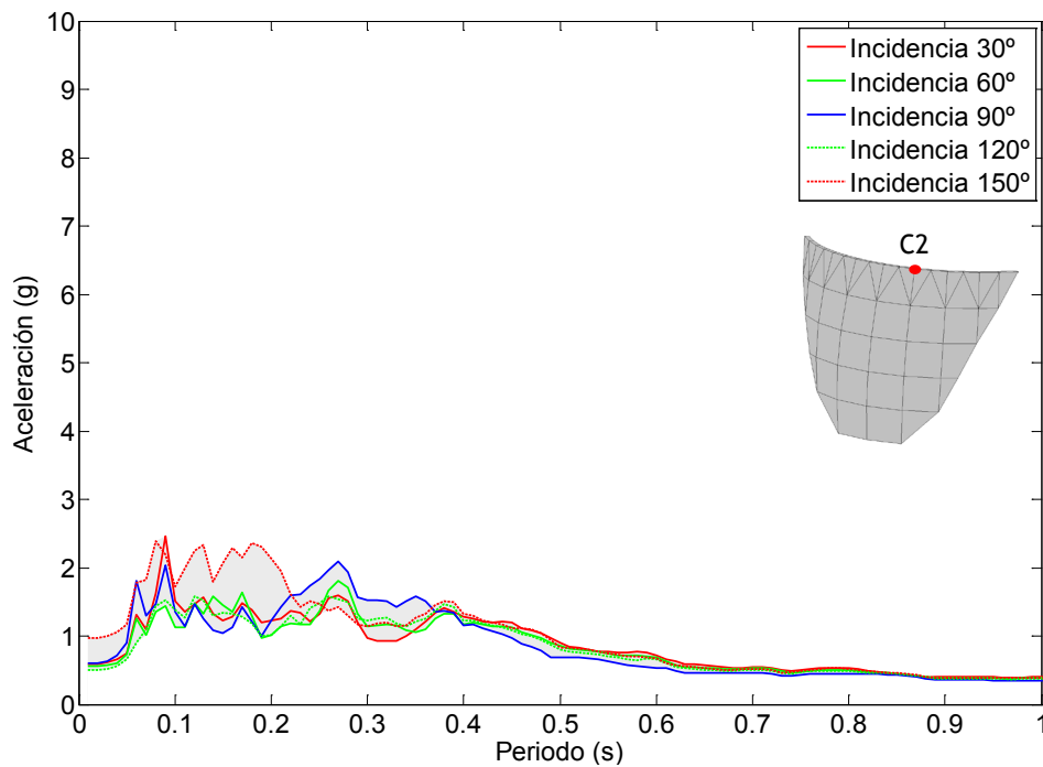
Figura 7.104. Nodo C2. Onda P+SV. Embalse con una capa de sedimentos de espesor H/5. Espectro de aceleraciones en dirección y.
