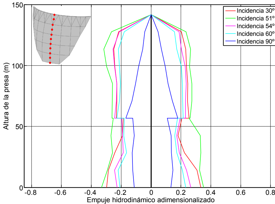
Figura 7.8. Onda P+SV. Embalse lleno de agua con una capa de sedimentos de espesor 2H/5 .
