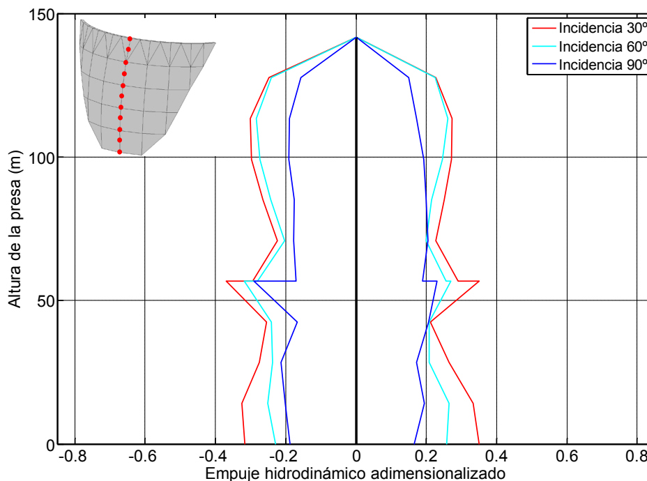
Figura 7.11. Onda P+SH+SV. Embalse lleno de agua con una capa de sedimentos de espesor 2H/5 .
