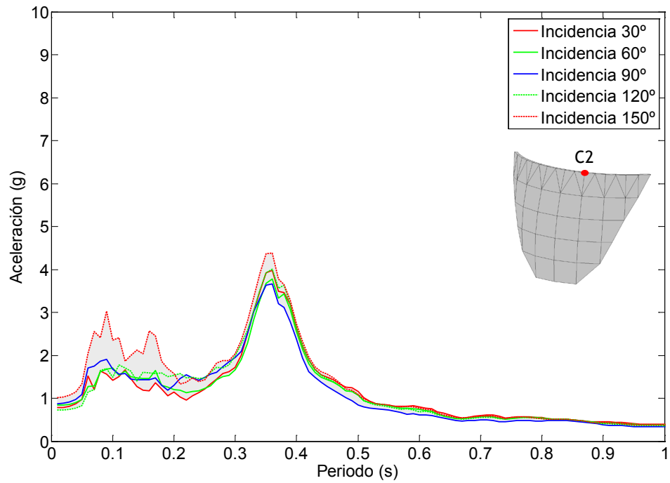
Figura 7.105. Nodo C2. Onda P+SV. Embalse con una capa de sedimentos de espesor 2H/5 . Espectro de aceleraciones en dirección y.
