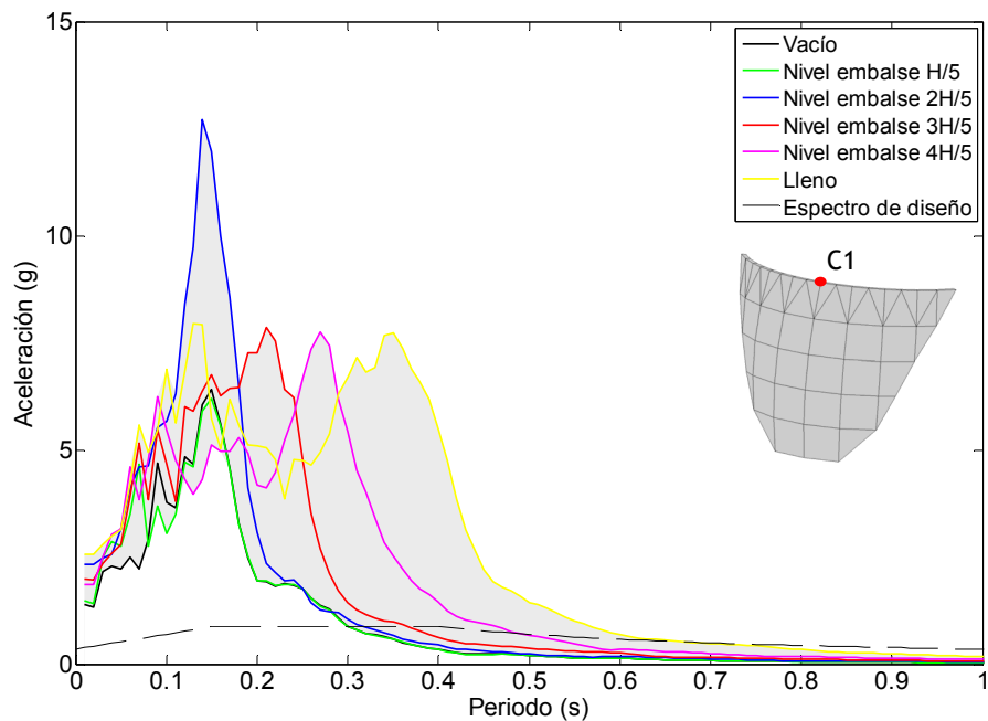
Figura 6.13. Nodo C1. Onda P. Embalse sin sedimentos. Espectro de aceleraciones en dirección x frente a diferentes niveles de llenado del embalse.
