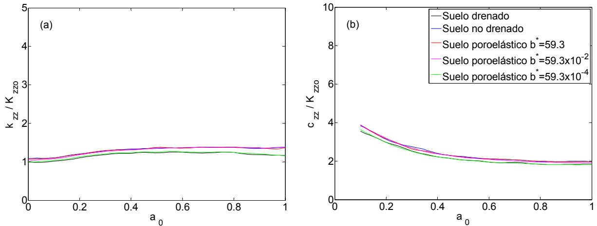
Figura 3.9. Influencia de la permeabilidad del suelo. Impedancia vertical. Pilote simple.
