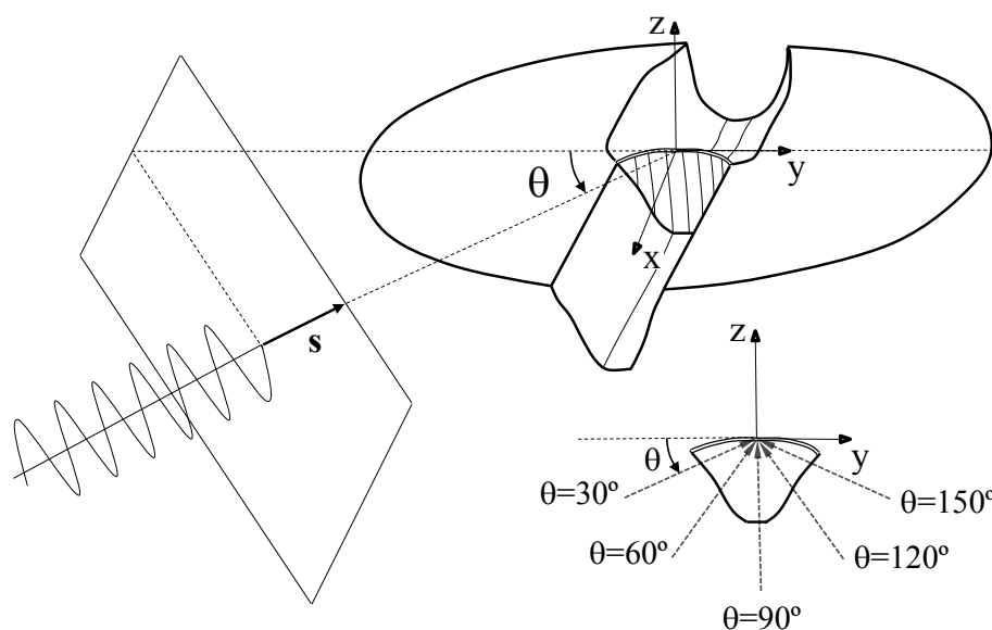
Figura 7.21. Definición de las incidencias estudiadas, todas ellas contenidas en el plano y-z.
