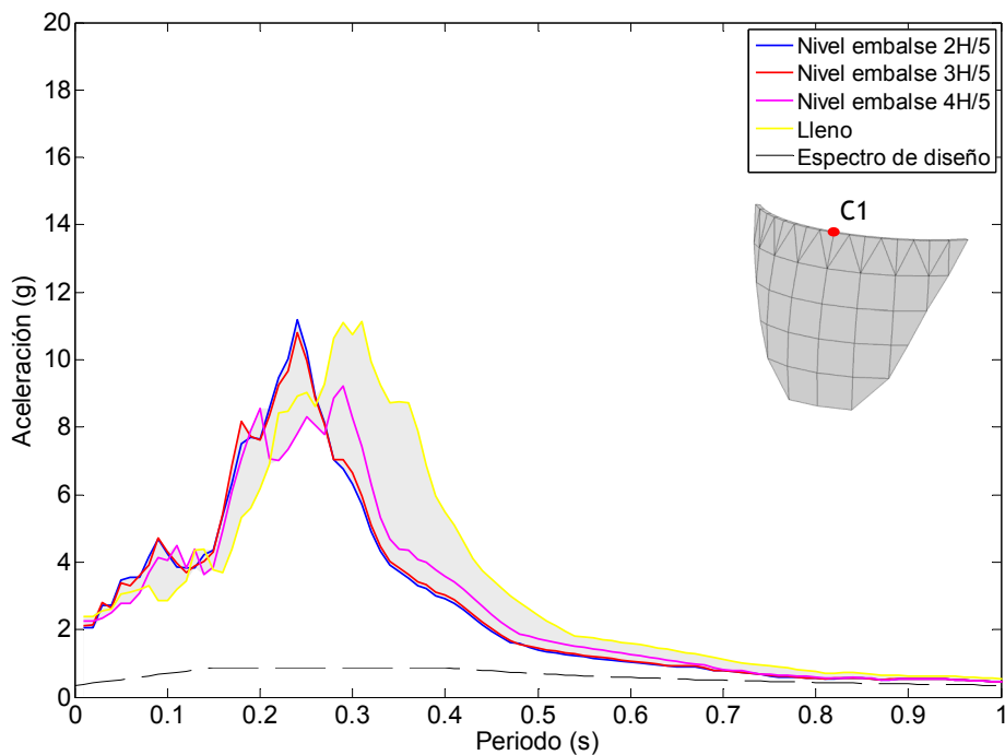
Figura 6.18. Nodo C1. Onda SH. Embalse con una capa de sedimentos de espesor 2H/5 . Espectro de aceleraciones en dirección x frente diferentes niveles de llenado del embalse.
