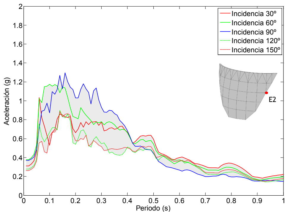
Figura 7.86. Nodo E2. Onda P+SH+SV. Embalse sin sedimentos. Espectro de aceleraciones de campo libre en dirección z.
