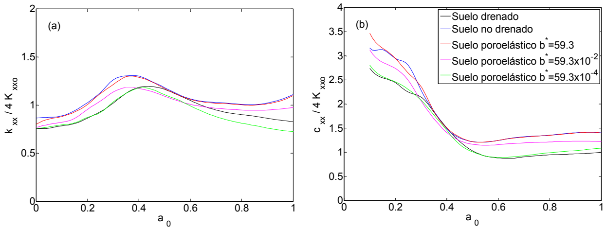
Figura 3.12. Influencia de la permabilidad del suelo. Impedancia horizontal. Grupo de pilotes 2 x 2 con s/d = 10 .
