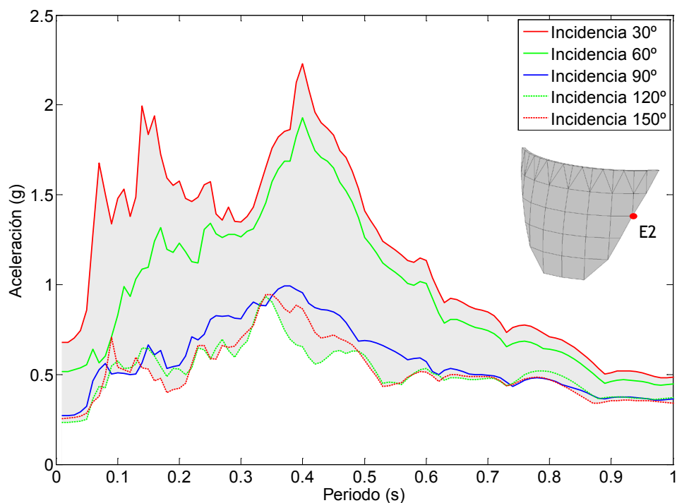
Figura 7.39. Nodo E2. Onda P+SV. Embalse sin sedimentos. Espectro de aceleraciones en dirección y.
