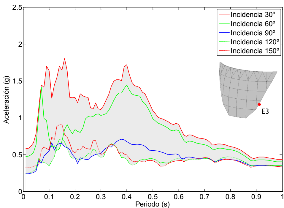
Figura 7.43. Nodo E3. Onda P+SV. Embalse sin sedimentos. Espectro de aceleraciones en dirección y.
