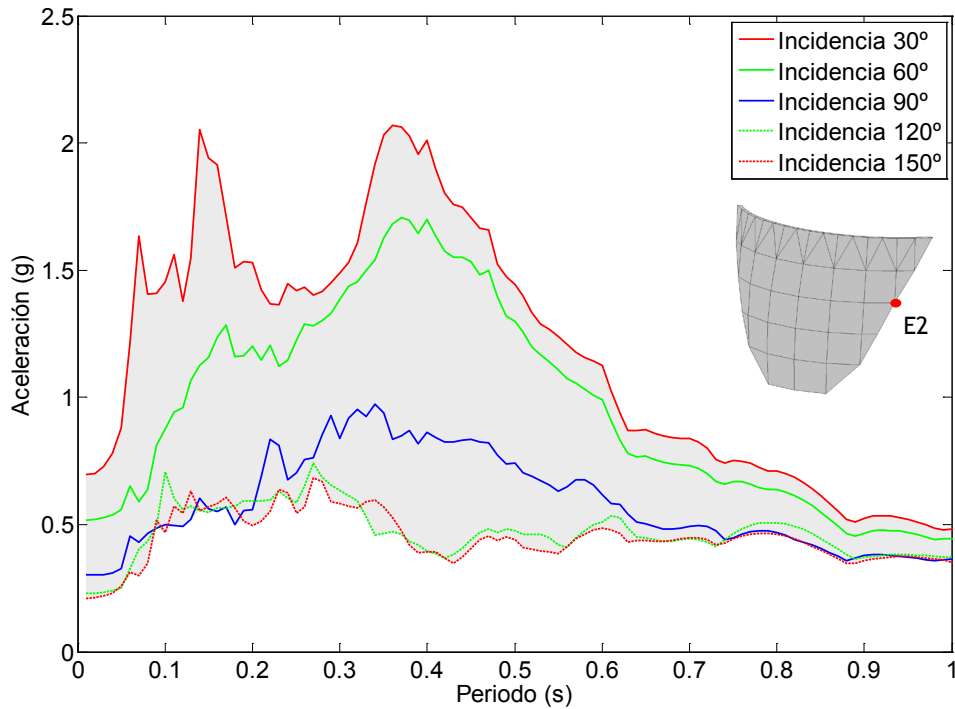
Figura 7.76. Nodo E2. Onda P+SH+SV. Embalse con una capa de sedimentos de espesor H/5 . Espectro de aceleraciones en dirección y.
