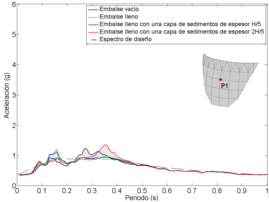
Figura 6.38. Nodo P1. Onda SV. Espectro de aceleraciones en dirección y frente a diferentes condiciones del embalse.
