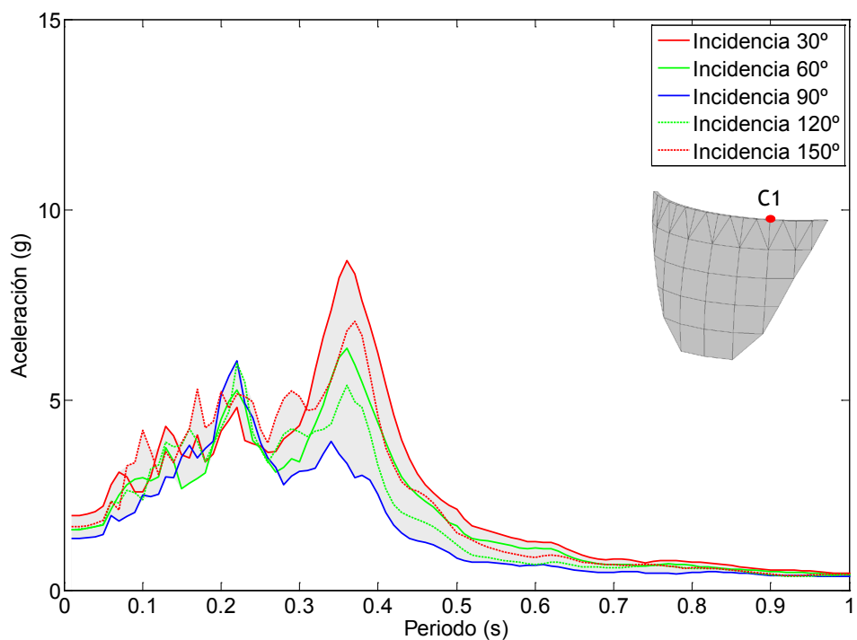
Figura 7.120. Nodo C1. Onda P+SH+SV. Embalse con una capa de sedimentos de espesor 2H/5 . Espectro de aceleraciones en dirección y.
