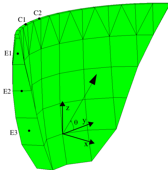
Figura 7.1. Puntos del estribo de la presa (E1, E2, E3) y de la coronación (C1, C2) de la bóveda en los que se han calculado los espectros de respuesta máxima de aceleraciones.
