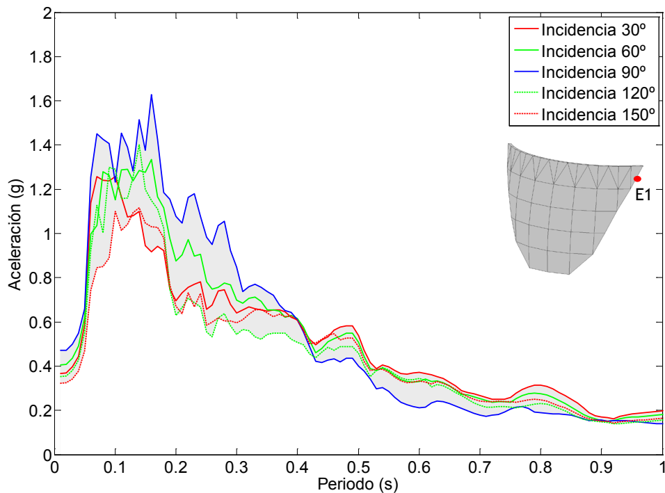
Figura 7.85. Nodo E1. Onda P+SH+SV. Embalse con una capa de sedimentos de espesor 2H/5 . Espectro de aceleraciones en dirección z.
