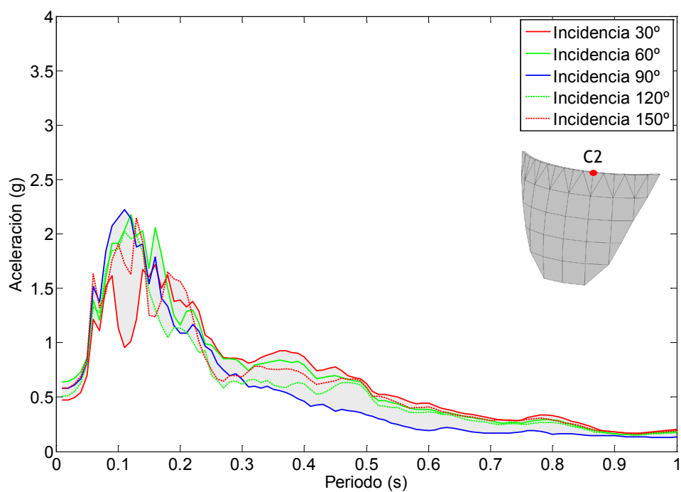
Figura 7.110. Nodo C2. Onda P+SV. Embalse con una capa de sedimentos de espesor H/5 . Espectro de aceleraciones en dirección z.
