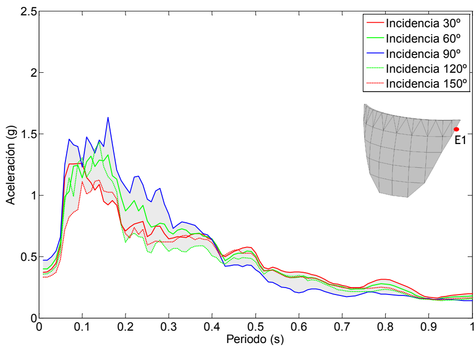
Figura 7.49. Nodo E1. Onda P+SV. Embalse con una capa de sedimentos de espesor 2H/5 . Espectro de aceleraciones en dirección z.
