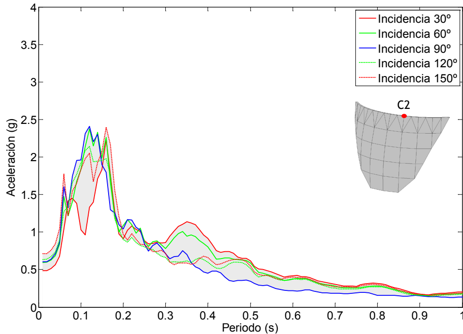
Figura 7.111. Nodo C2. Onda P+SV. Embalse con una capa de sedimentos de espesor 2H/5 . Espectro de aceleraciones en dirección z.
