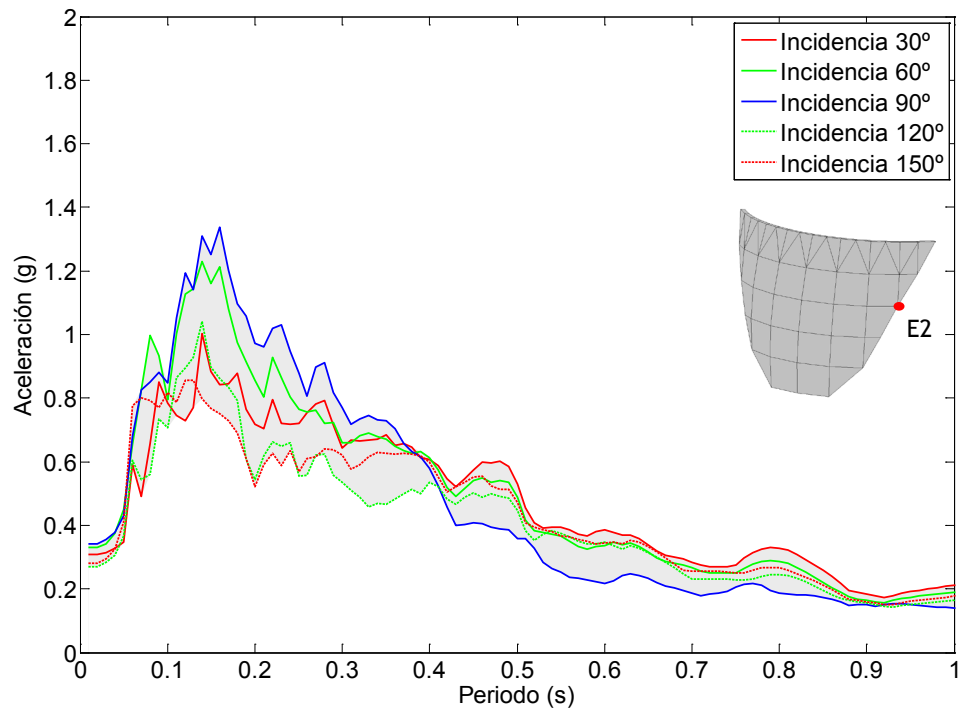
Figura 7.88. Nodo E2. Onda P+SH+SV. Embalse con una capa de sedimentos de espesor H/5 . Espectro de aceleraciones en dirección z.
