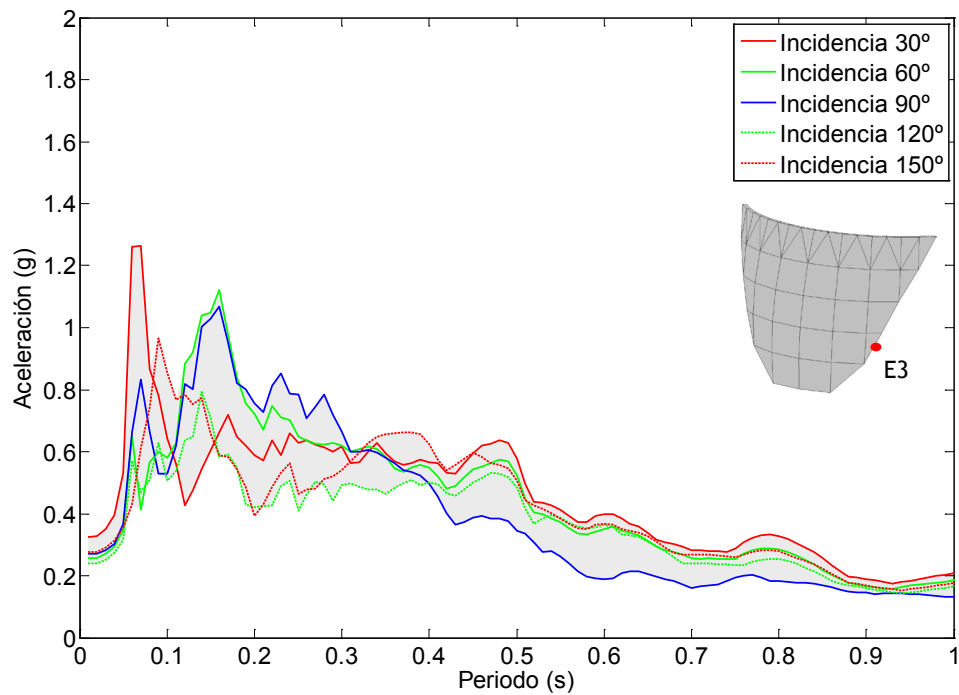
Figura 7.93. Nodo E3. Onda P+SH+SV. Embalse con una capa de sedimentos de espesor 2H/5 . Espectro de aceleraciones en dirección z.
