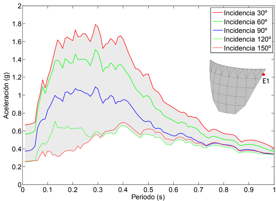
Figura 7.58. Nodo E1. Onda P+SH+SV. Embalse sin sedimentos. Espectro de aceleraciones de campo libre en dirección x.
