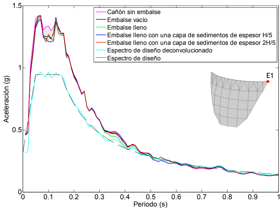
Figura 6.20. Nodo E1. Onda P. Espectro de aceleraciones en dirección z frente a diferentes condiciones del embalse.
