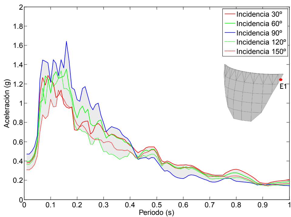
Figura 7.83. Nodo E1. Onda P+SH+SV. Embalse sin sedimentos. Espectro de aceleraciones en dirección z.
