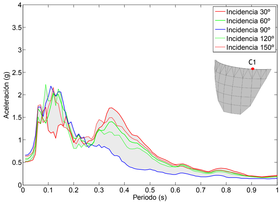
Figura 7.124. Nodo C1. Onda P+SH+SV. Embalse sin sedimentos. Espectro de aceleraciones en dirección z.
