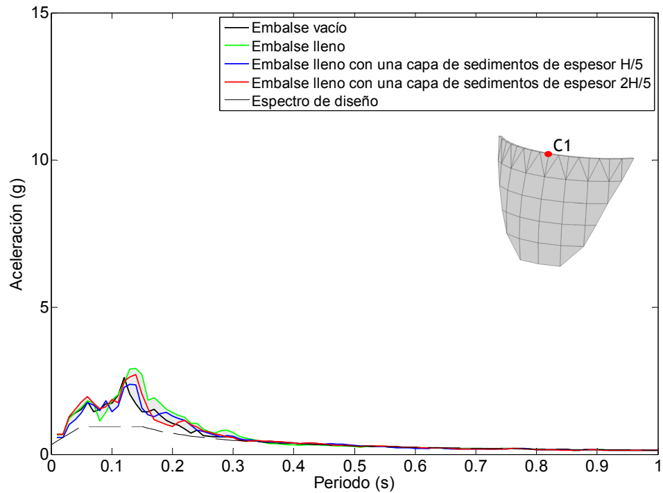
Figura 6.40. Nodo C1. Onda P. Espectro de aceleraciones en dirección z frente a diferentes condiciones del embalse.
