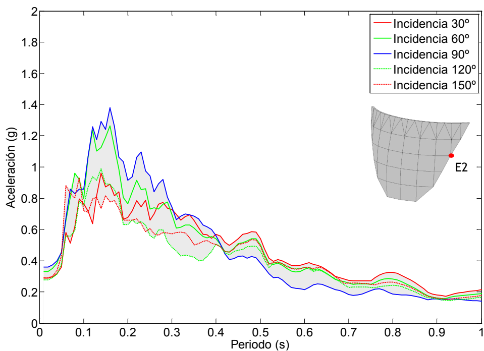
Figura 7.87. Nodo E2. Onda P+SH+SV. Embalse sin sedimentos. Espectro de aceleraciones en dirección z.
