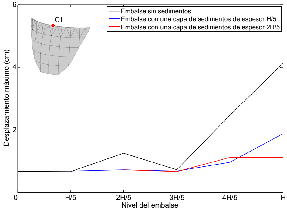
Figura 6.11. Nodo C1. Onda P. Desplazamientos máximos en dirección x frente al nivel de llenado del embalse.
