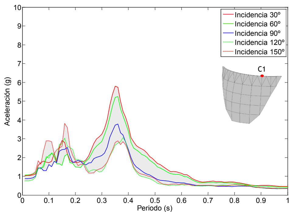
Figura 7.102. Nodo C1. Onda P+SV. Embalse con una capa de sedimentos de espesor 2H/5 . Espectro de aceleraciones en dirección y.
