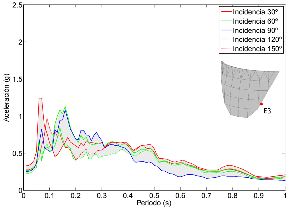
Figura 7.57. Nodo E3. Onda P+SV. Embalse con una capa de sedimentos de espesor 2H/5 . Espectro de aceleraciones en dirección z.
