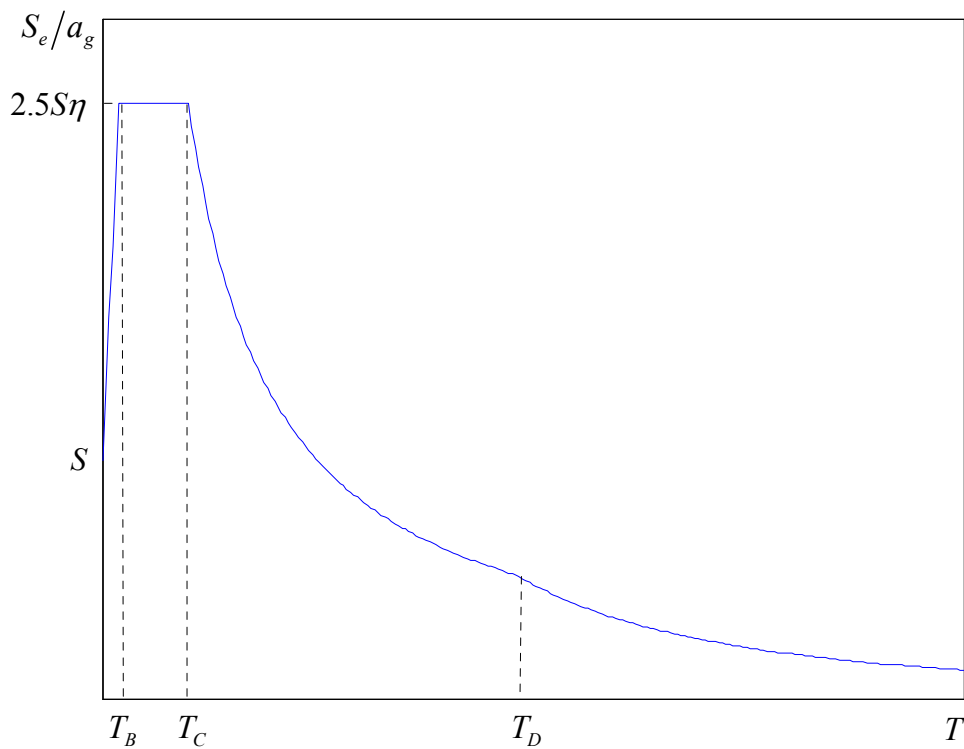
Figura 5.1. Forma características de los espectros de respuesta elástica según el Eurocódigo 8.
