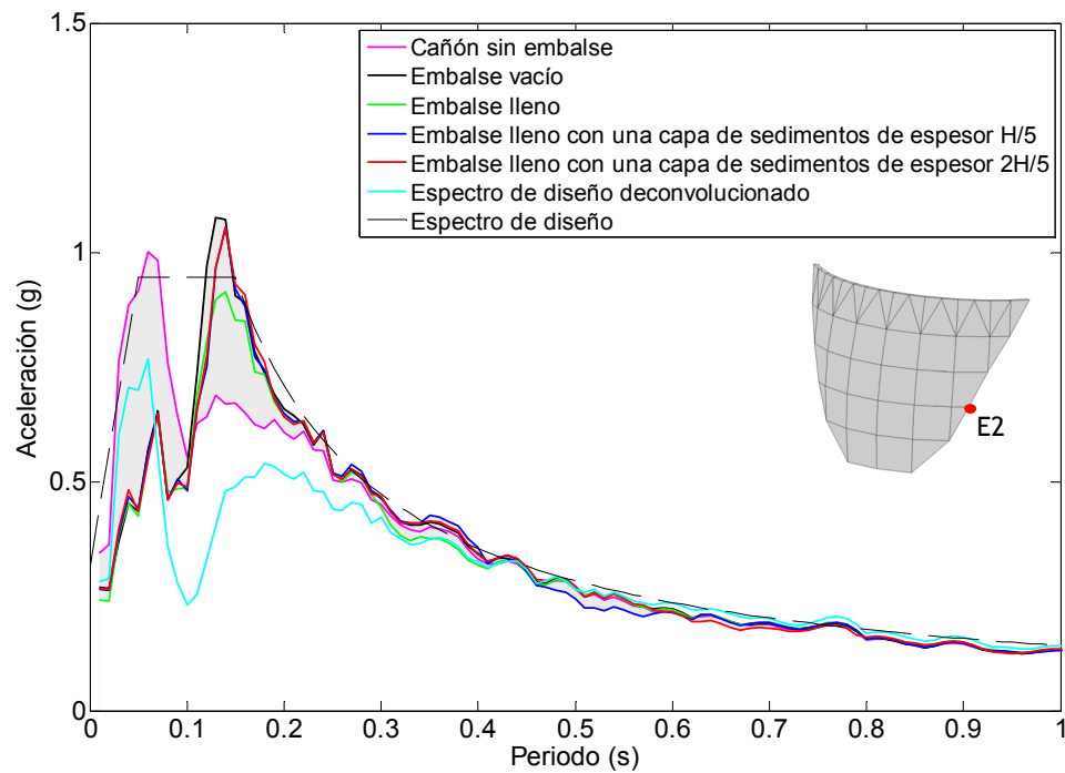
Figura 6.24. Nodo E2. Onda P. Espectro de aceleraciones en dirección z frente a diferentes condiciones del embalse.
