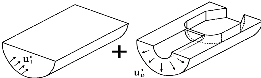
Figura 4.13. Modelo de la excitación sísmica. Campo total en suelo como superposición del campo incidente \mathbf{u}_I^s y difractado \mathbf{u}_D^s .
