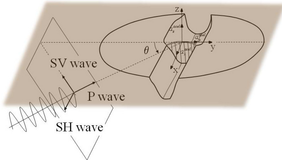
Figura 5.14. Sistema de referencia empleado en el modelo en relación con las componentes de los acelerogramas.
