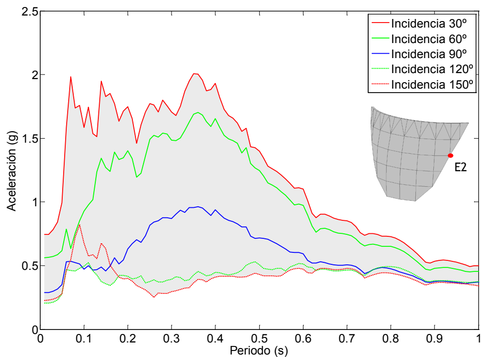
Figura 7.74. Nodo E2. Onda P+SH+SV. Embalse sin sedimentos. Espectro de aceleraciones de campo libre en dirección y.
