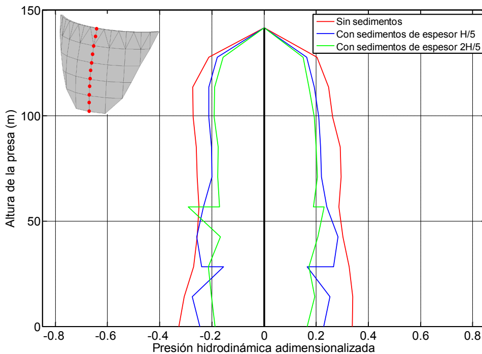
Figura 7.20. Onda P+SH+SV. Incidencia 90°.
