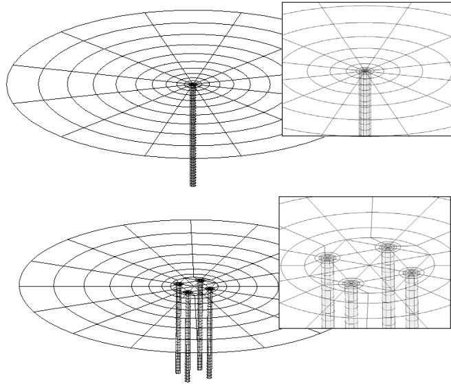
Figura 3.3. Discretizaciones de elementos de contorno para un pilote simple y para un grupo de pilotes 2×2 embebidos en un semi-espacio.
