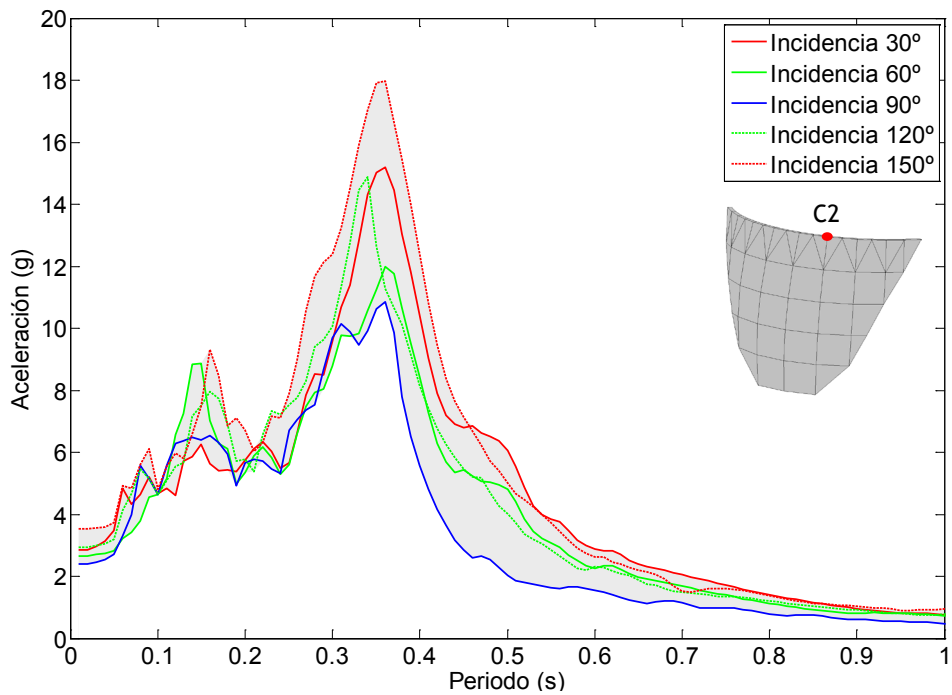
Figura 7.117. Nodo C2. Onda P+SH+SV. Embalse con una capa de sedimentos de espesor 2H/5 . Espectro de aceleraciones en dirección x.
