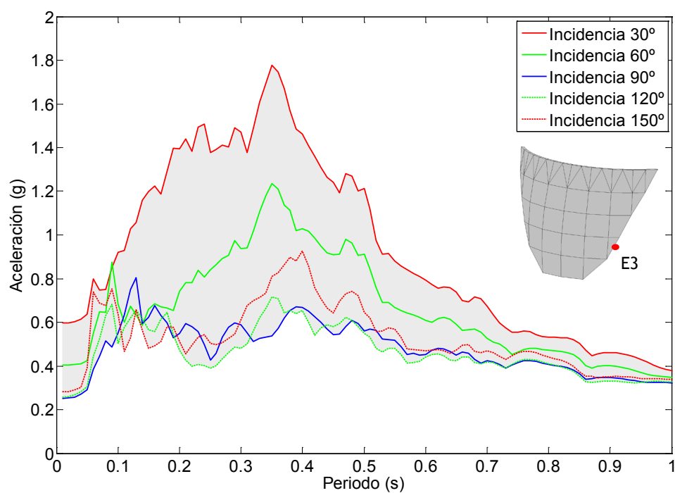
Figura 7.67. Nodo E3. Onda P+SH+SV. Embalse sin sedimentos. Espectro de aceleraciones en dirección x.
