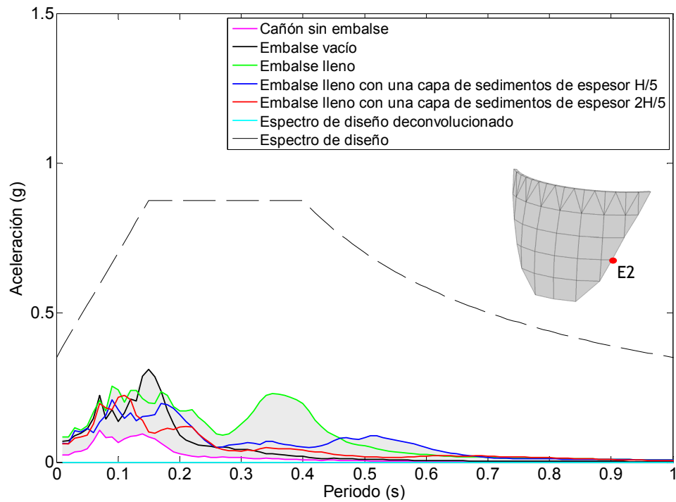
Figura 6.23. Nodo E2. Onda P. Espectro de aceleraciones en dirección x frente a diferentes condiciones del embalse.
