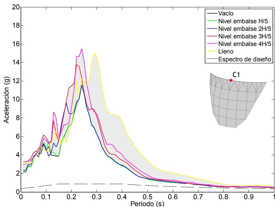
Figura 6.16. Nodo C1. Onda SH. Embalse sin sedimentos. Espectro de aceleraciones en dirección x frente diferentes niveles de llenado del embalse.
