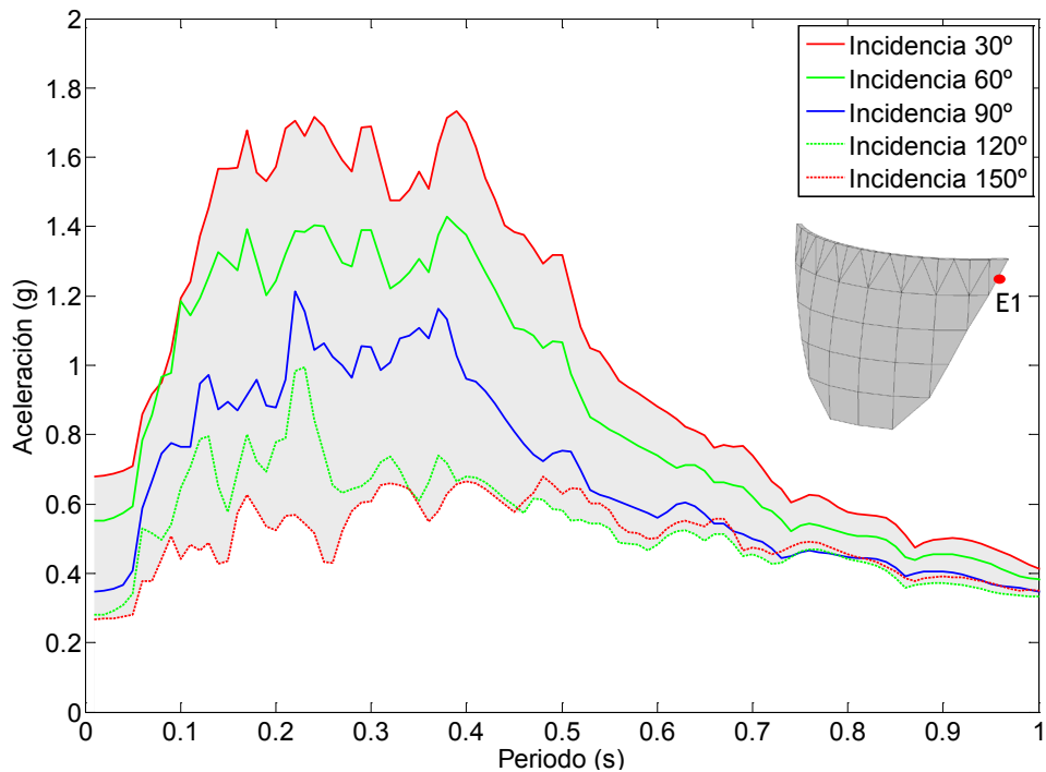
Figura 7.61. Nodo E1. Onda P+SH+SV. Embalse con una capa de sedimentos de espesor 2H/5 . Espectro de aceleraciones en dirección x.
