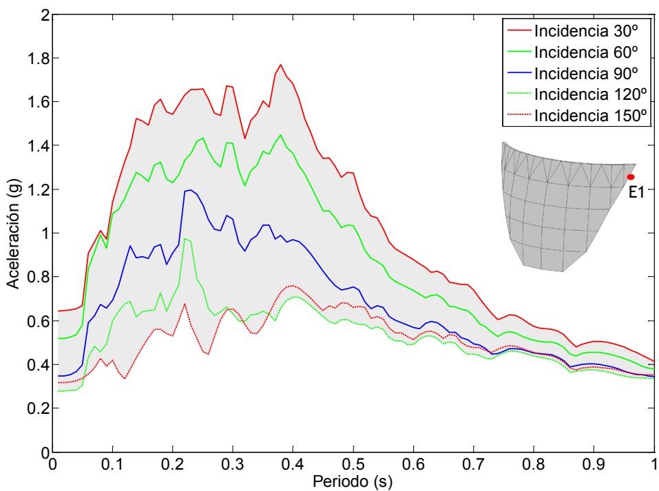
Figura 7.24. Nodo E1. Onda SH. Embalse con una capa de sedimentos de espesor H/5 . Espectro de aceleraciones en dirección x.
