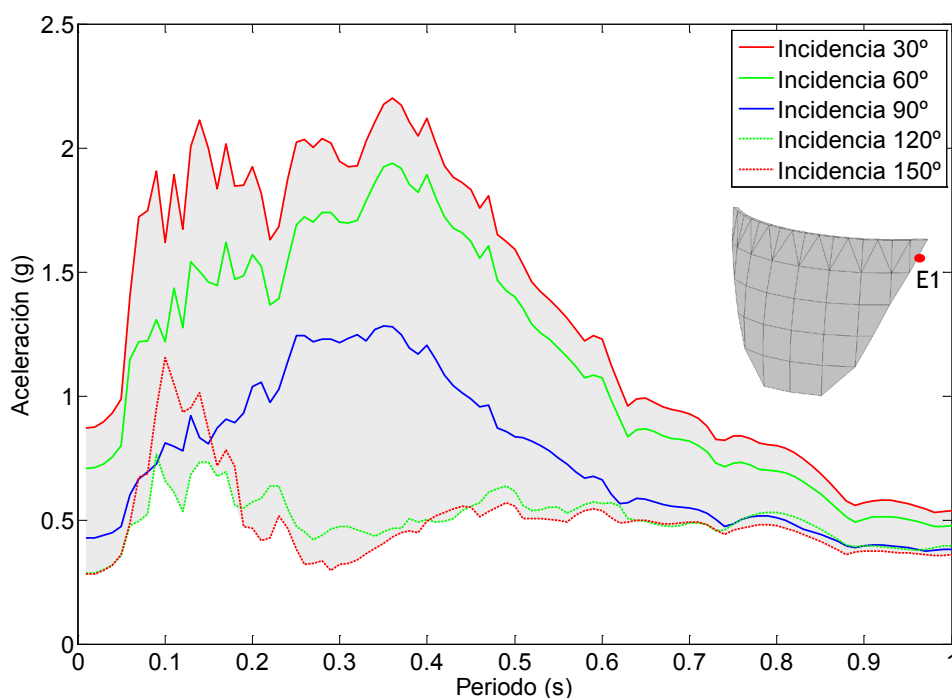
Figura 7.34. Nodo E1. Onda P+SV. Embalse sin sedimentos. Espectro de aceleraciones de campo libre en dirección y.
