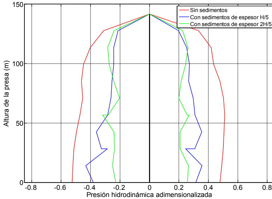
Figura 7.19. Onda P+SH+SV. Incidencia 60°.
