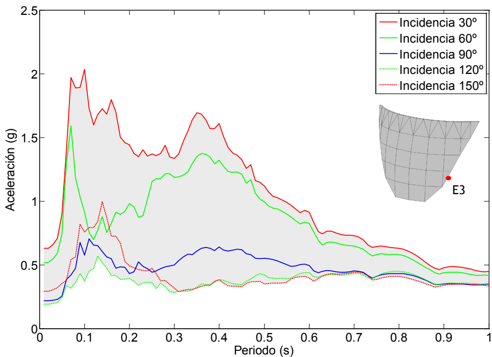
Figura 7.42. Nodo E3. Onda P+SV. Embalse sin sedimentos. Espectro de aceleraciones de campo libre en dirección y.
