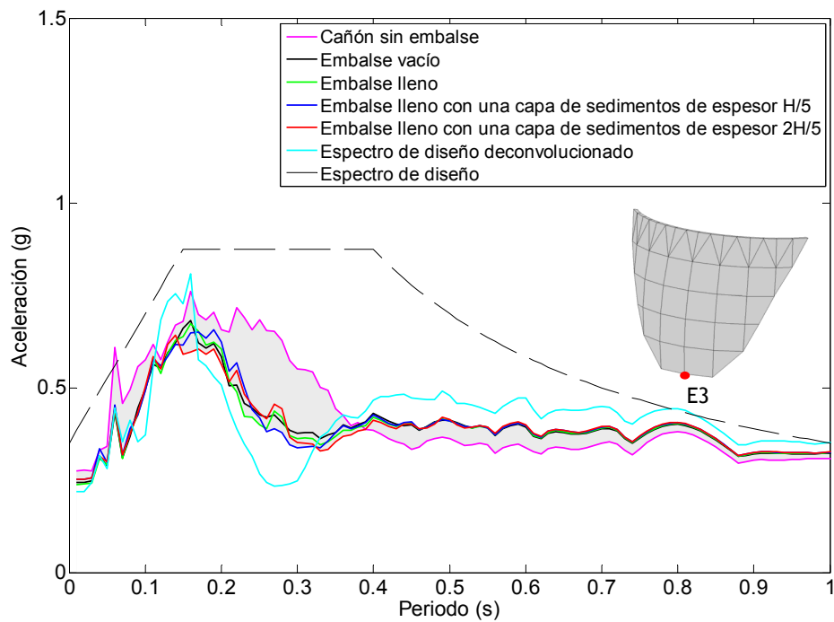
Figura 6.30. Nodo E3. Onda SV. Espectro de aceleraciones en dirección y frente a diferentes condiciones del embalse.
