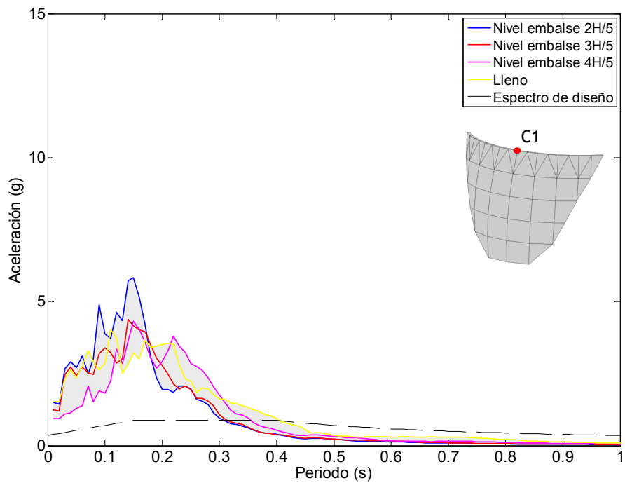
Figura 6.15. Nodo C1. Onda P. Embalse con una capa de sedimentos de espesor 2H/5 . Espectro de aceleraciones en dirección x frente diferentes niveles de llenado del embalse.
