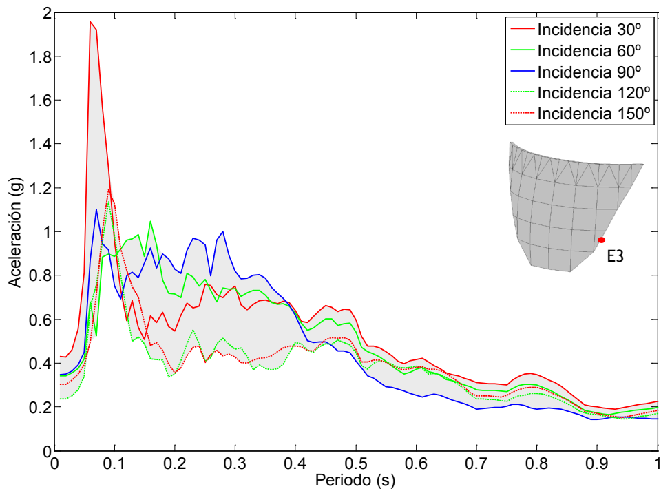
Figura 7.90. Nodo E3. Onda P+SH+SV. Embalse sin sedimentos. Espectro de aceleraciones de campo libre en dirección z.
