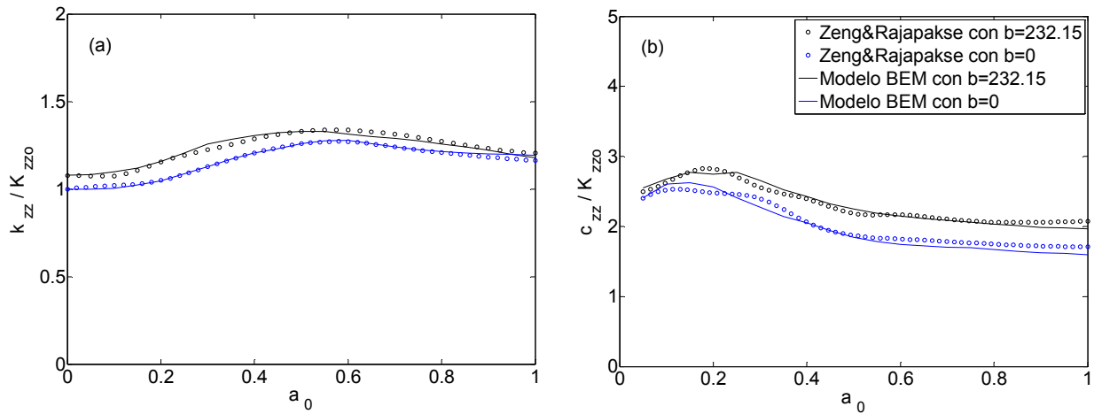
Figura 3.5. Impedancia vertical de un pilote simple en un medio poroelástico. Comparación con los resultados de Zeng & Rajapakse.
