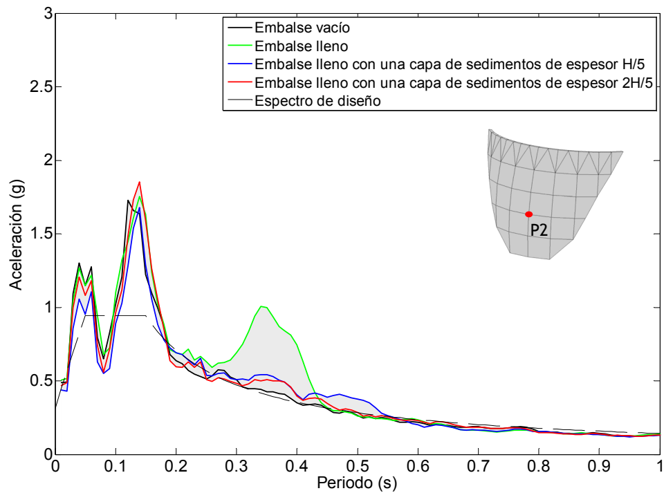
Figura 6.32. Nodo P2. Onda P. Espectro de aceleraciones en dirección z frente a diferentes condiciones del embalse.
