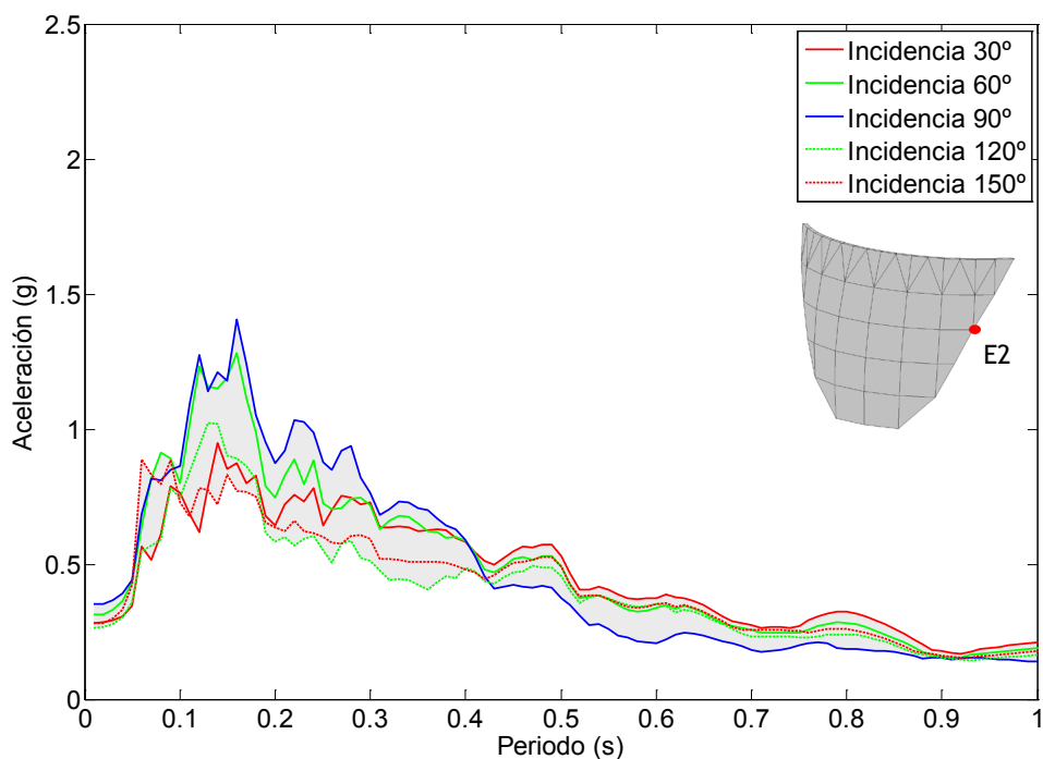
Figura 7.51. Nodo E2. Onda P+SV. Embalse sin sedimentos. Espectro de aceleraciones en dirección z.
