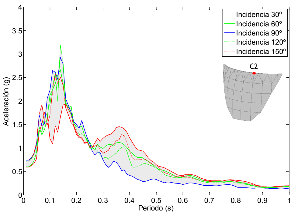
Figura 7.127. Nodo C2. Onda P+SH+SV. Embalse sin sedimentos. Espectro de aceleraciones en dirección z.
