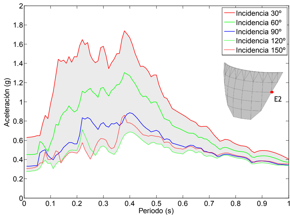
Figura 7.27. Nodo E2. Onda SH. Embalse sin sedimentos. Espectro de aceleraciones en dirección x.
