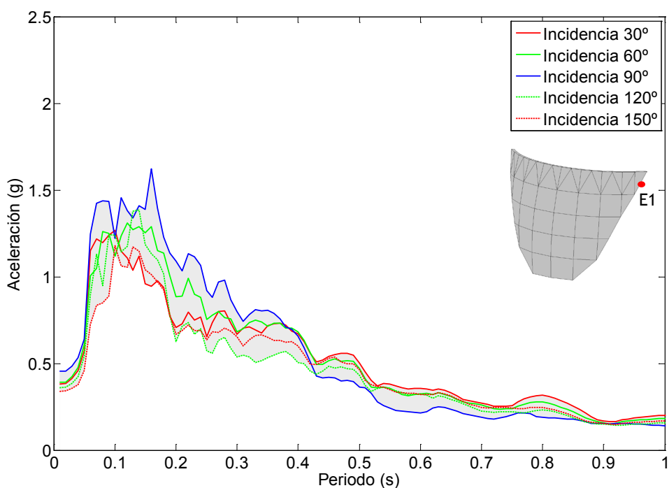
Figura 7.48. Nodo E1. Onda P+SV. Embalse con una capa de sedimentos de espesor H/5 . Espectro de aceleraciones en dirección z.
