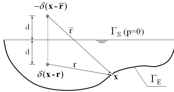
Figura 2.3. Posición de las cargas para la obtención de la solución fundamental fuente-imagen en problemas escalares.
