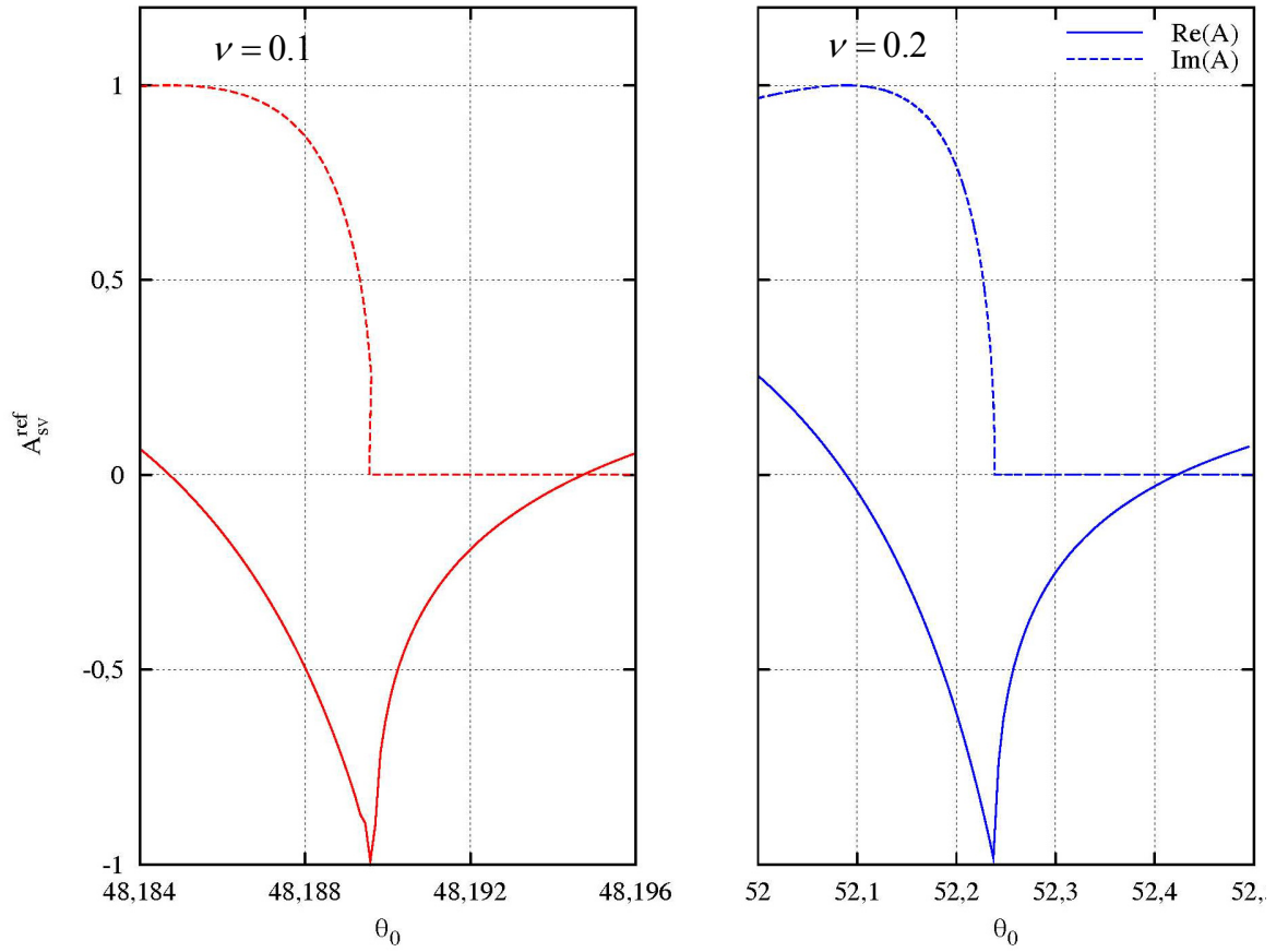
Figura 4.9. Detalle en las inmediaciones del ángulo crítico de la amplitud de la onda SV reflejada con el ángulo de Incidencia \theta_0 .
