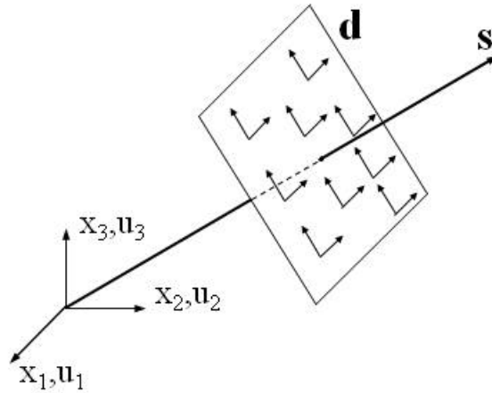
Figura 2.2. Desplazamiento y dirección de propagación para el caso de una onda plana S.
