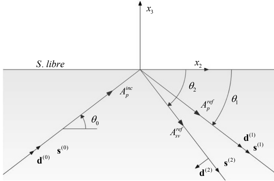
Figura 4.4. Ángulos de interés en el plano x_2x_3 para una onda P incidente.
