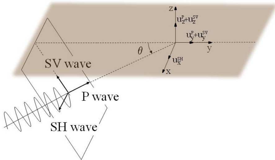
Figura 5.13. Desplazamientos provocados en el problema de campo libre por un tren de ondas planas con dirección de propagación contenida en el plano y-z.
