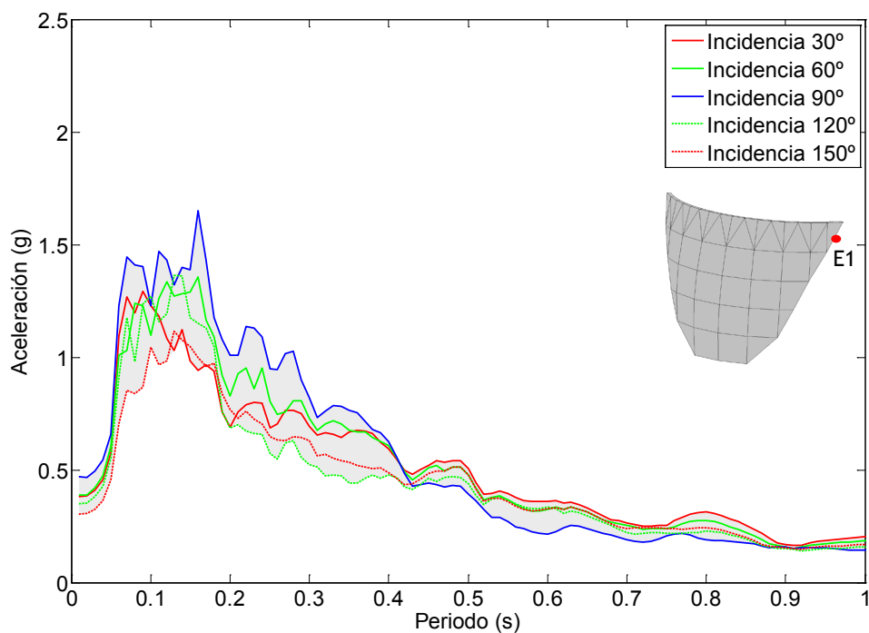
Figura 7.47. Nodo E1. Onda P+SV. Embalse sin sedimentos. Espectro de aceleraciones en dirección z.
