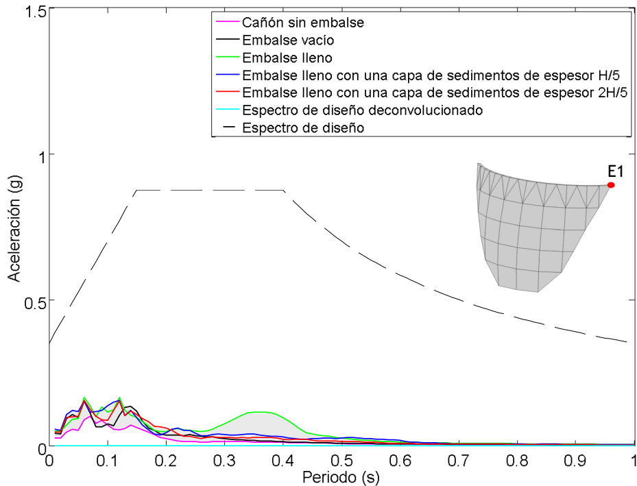
Figura 6.19. Nodo E1. Onda P. Espectro de aceleraciones en dirección x frente a diferentes condiciones del embalse.
