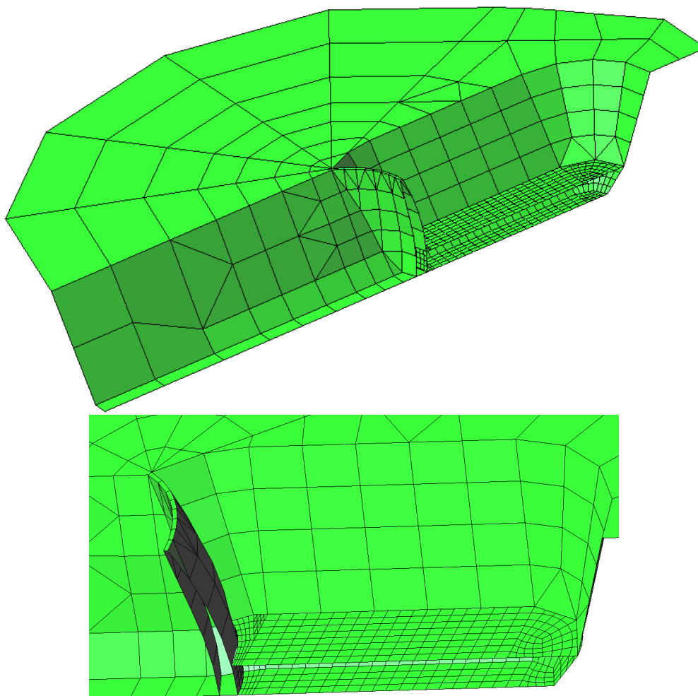
Figura 6.4. Discretización de elementos de contorno del sistema acoplado cuando el modelo incorpora una capa de sedimentos de espesor H/5 . 744 elementos y 3259 nodos.
