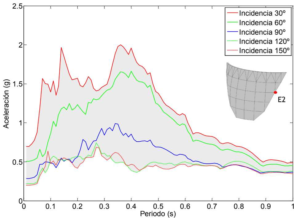
Figura 7.77. Nodo E2. Onda P+SH+SV. Embalse con una capa de sedimentos de espesor 2H/5 . Espectro de aceleraciones en dirección y.
