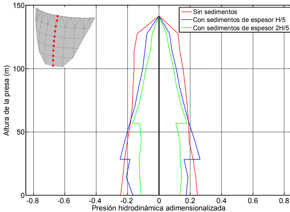
Figura 7.17. Onda P+SV. Incidencia 90°.
