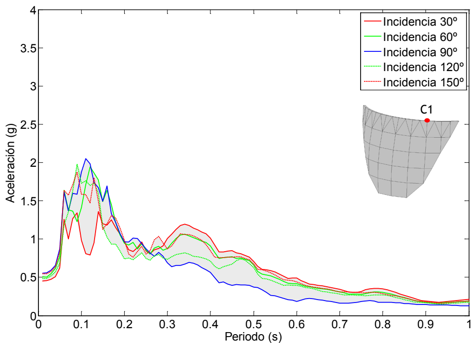
Figura 7.107. Nodo C1. Onda P+SV. Embalse con una capa de sedimentos de espesor H/5 . Espectro de aceleraciones en dirección z.
