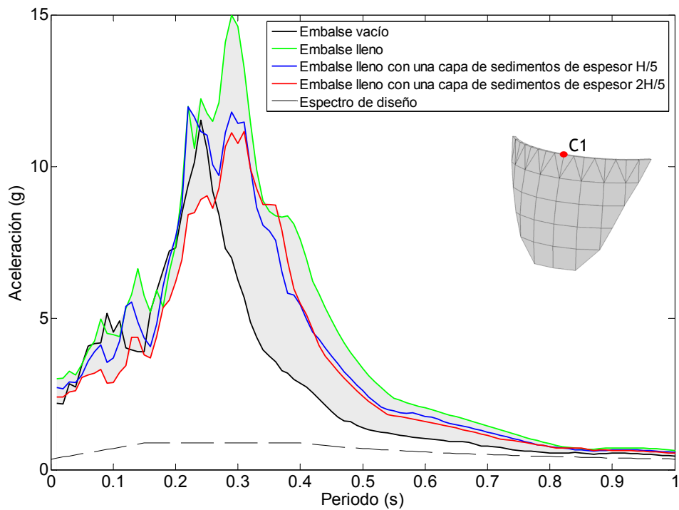
Figura 6.41. Nodo C1. Onda SH. Espectro de aceleraciones en dirección x frente a diferentes condiciones del embalse.
