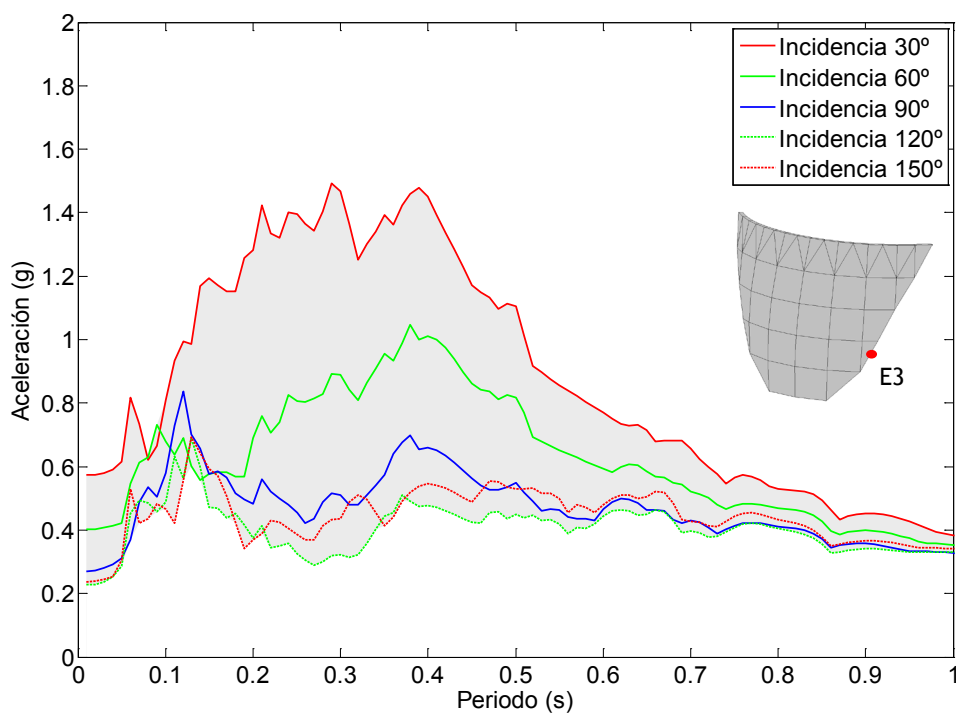
Figura 7.69. Nodo E3. Onda P+SH+SV. Embalse con una capa de sedimentos de espesor 2H/5 . Espectro de aceleraciones en dirección x.
