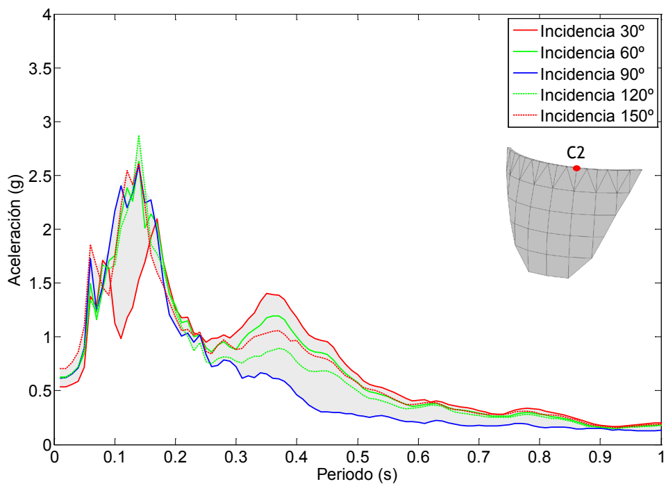
Figura 7.109. Nodo C2. Onda P+SV. Embalse sin sedimentos. Espectro de aceleraciones en dirección z.
