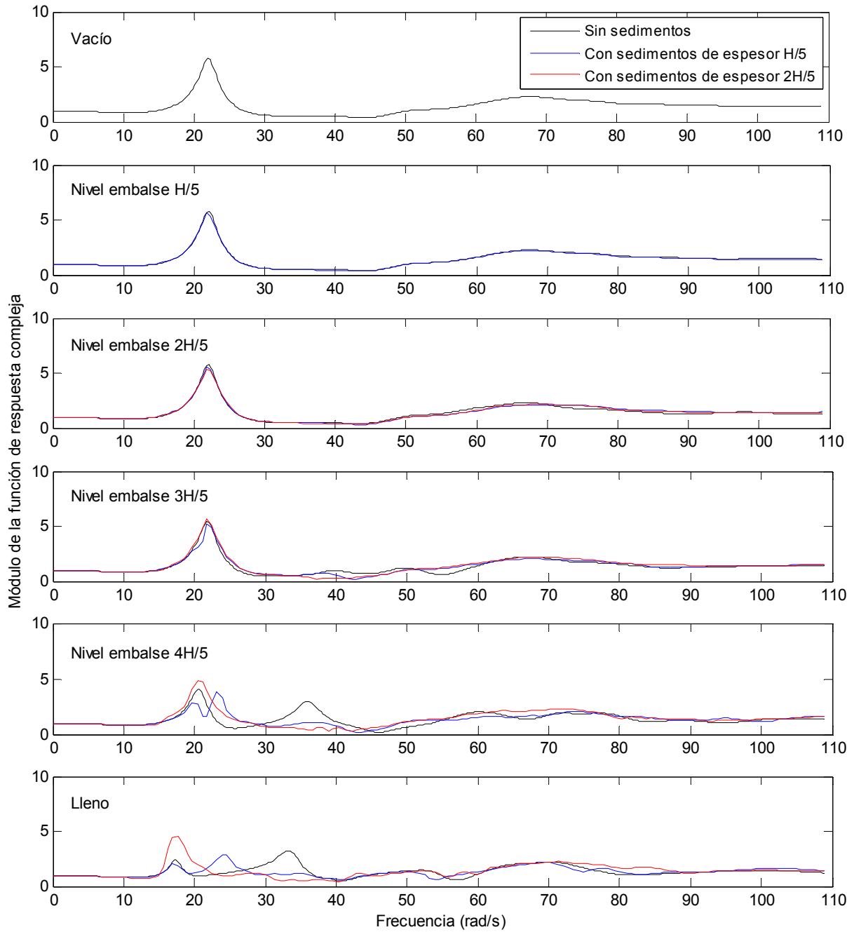
Figura 6.10. Módulo de la función de respuesta compleja en dirección y. Nodo C1. Onda SV con incidencia vertical.
