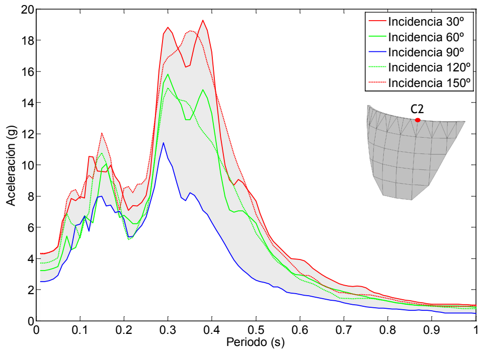
Figura 7.115. Nodo C2. Onda P+SH+SV. Embalse sin sedimentos. Espectro de aceleraciones en dirección x.
