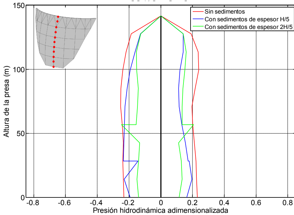
Figura 7.13. Onda SH. Incidencia 60°.
