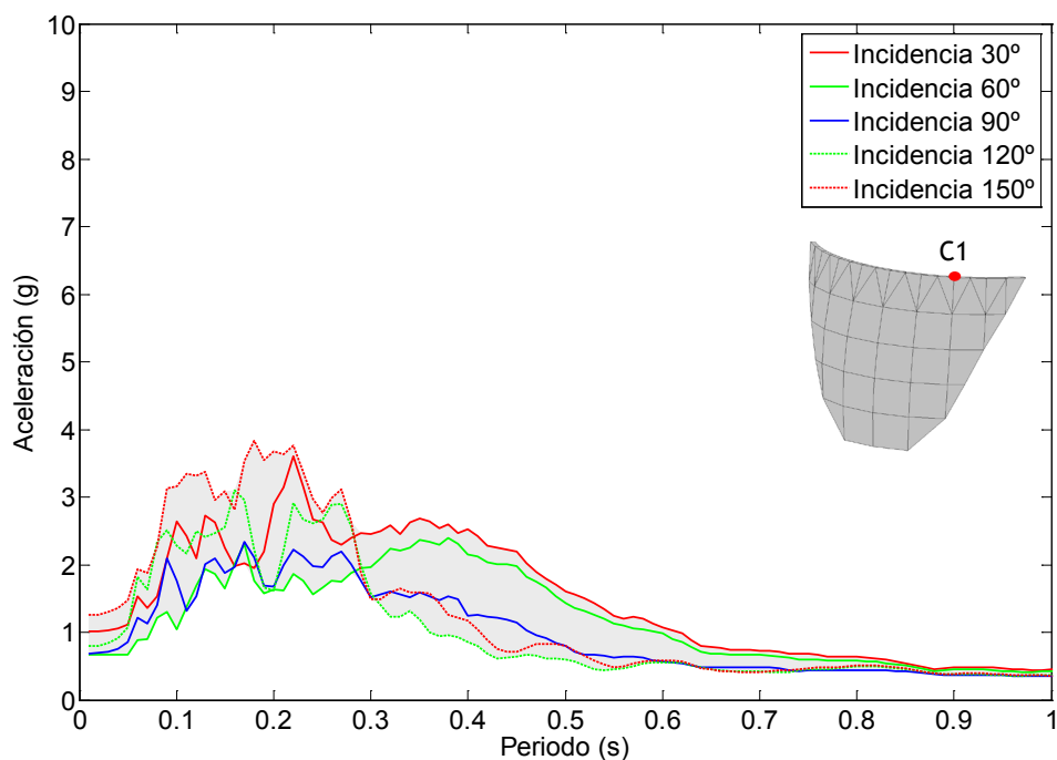
Figura 7.101. Nodo C1. Onda P+SV. Embalse con una capa de sedimentos de espesor H/5 . Espectro de aceleraciones en dirección y.
