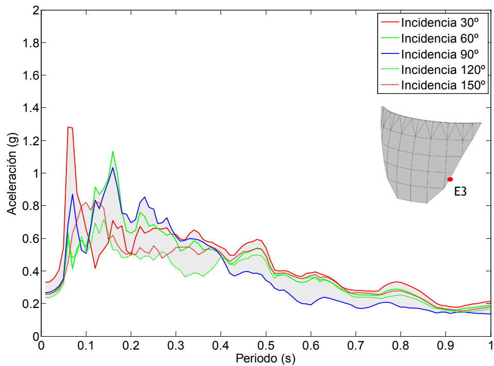
Figura 7.91. Nodo E3. Onda P+SH+SV. Embalse sin sedimentos. Espectro de aceleraciones en dirección z.
