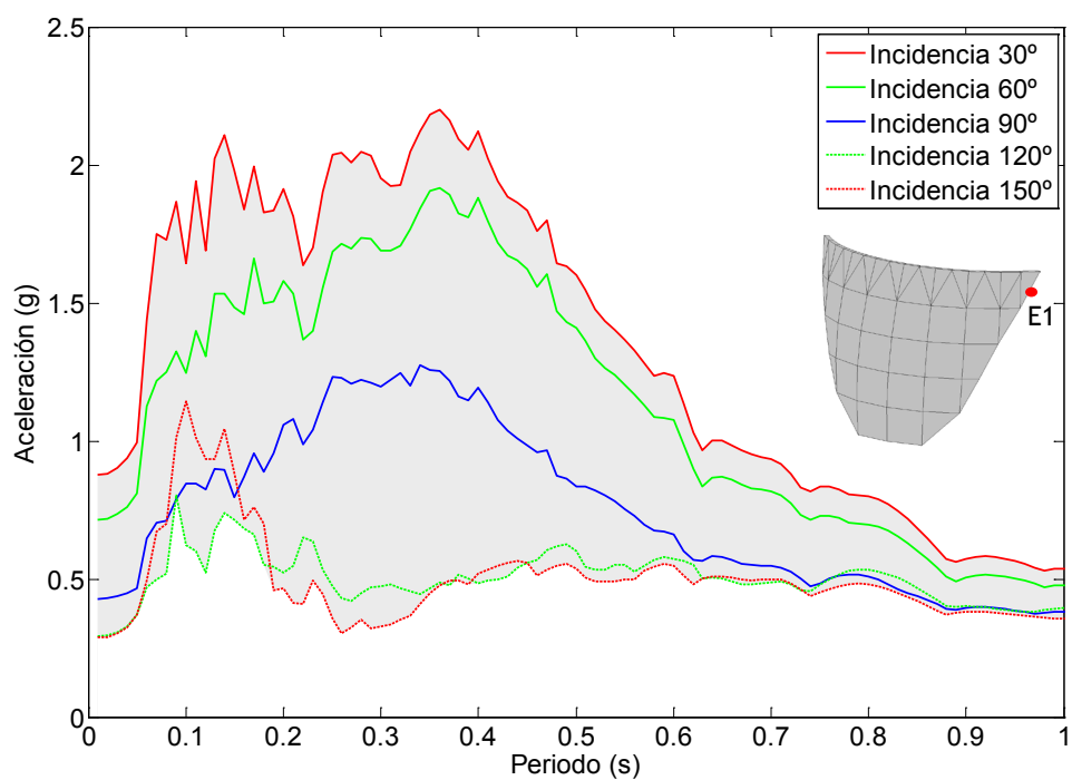
Figura 7.70. Nodo E1. Onda P+SH+SV. Embalse sin sedimentos. Espectro de aceleraciones de campo libre en dirección y.
