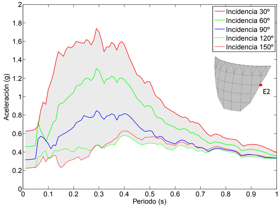
Figura 7.26. Nodo E2. Onda SH. Embalse sin sedimentos. Espectro de aceleraciones de campo libre en dirección x.
