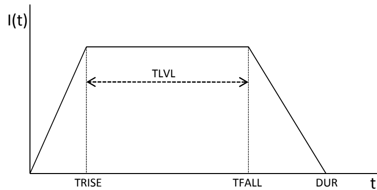
Figura 5.4. Función de modulación de intensidad trapezoidal y parámetros para su definición.
