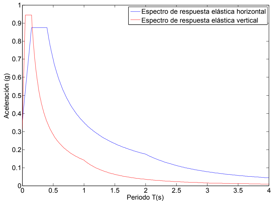
Figura 5.3. Espectros de diseño tipo 1 según EN 1998-1:2004 (E) para un suelo A tomando como aceleración pico 0.35g y un 5% de amortiguamiento.
