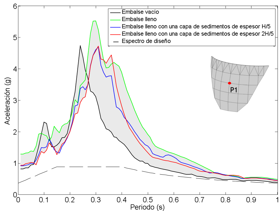
Figura 6.37. Nodo P1. Onda SH. Espectro de aceleraciones en dirección x frente a diferentes condiciones del embalse.
