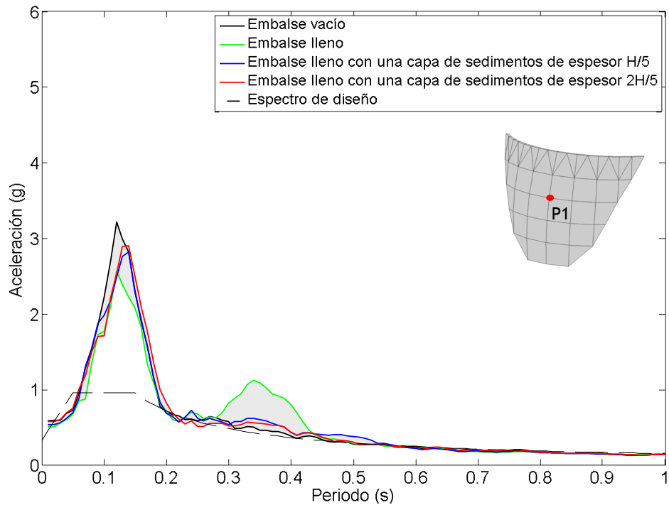
Figura 6.36. Nodo P1. Onda P. Espectro de aceleraciones en dirección z frente a diferentes condiciones del embalse.
