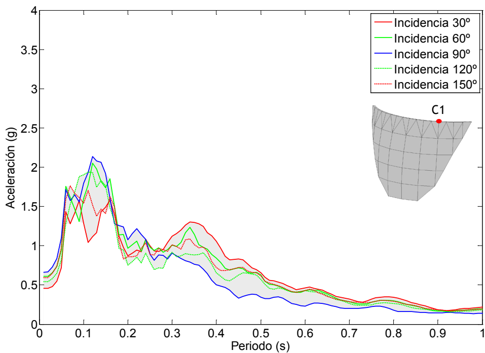
Figura 7.126. Nodo C1. Onda P+SH+SV. Embalse con una capa de sedimentos de espesor 2H/5 . Espectro de aceleraciones en dirección z.
