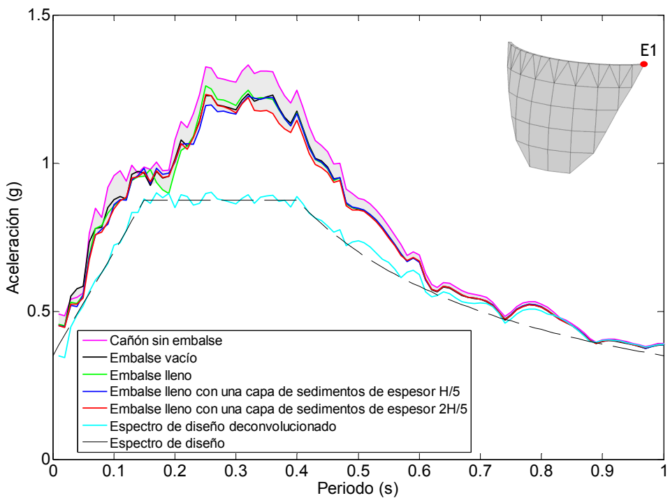
Figura 6.22. Nodo E1. Onda SV. Espectro de aceleraciones en dirección y frente a diferentes condiciones del embalse.
