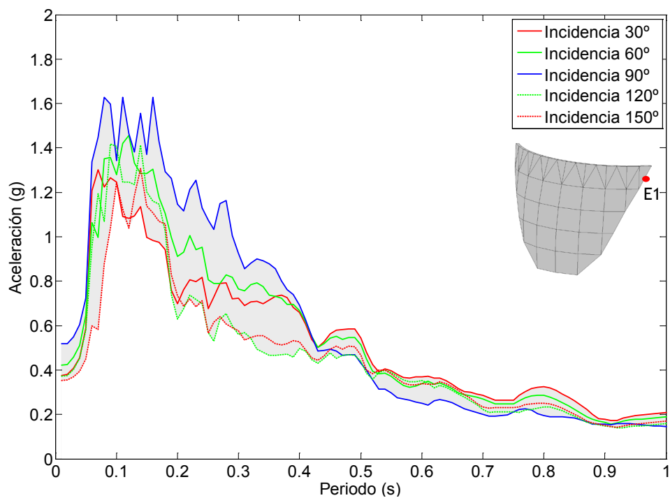
Figura 7.82. Nodo E1. Onda P+SH+SV. Embalse sin sedimentos. Espectro de aceleraciones de campo libre en dirección z.
