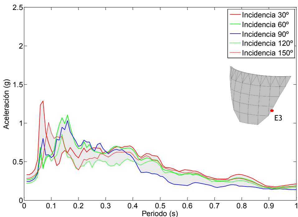
Figura 7.56. Nodo E3. Onda P+SV. Embalse con una capa de sedimentos de espesor H/5 . Espectro de aceleraciones en dirección z.
