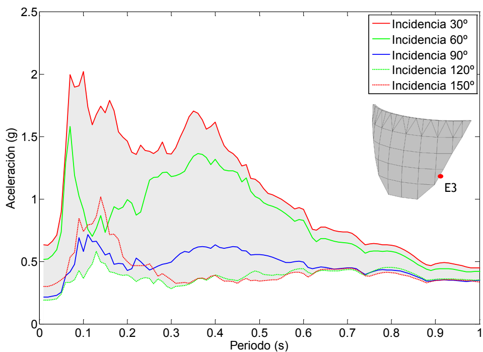
Figura 7.78. Nodo E3. Onda P+SH+SV. Embalse sin sedimentos. Espectro de aceleraciones de campo libre en dirección y.
