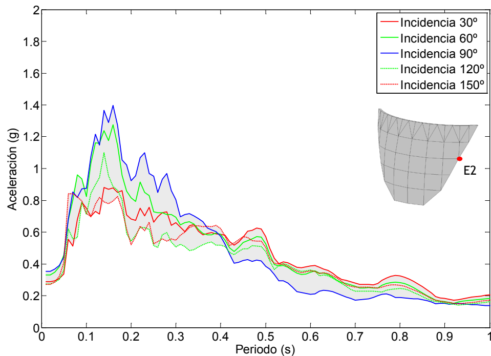
Figura 7.89. Nodo E2. Onda P+SH+SV. Embalse con una capa de sedimentos de espesor 2H/5 . Espectro de aceleraciones en dirección z.
