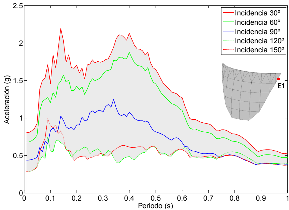
Figura 7.72. Nodo E1. Onda P+SH+SV. Embalse con una capa de sedimentos de espesor H/5 . Espectro de aceleraciones en dirección y.
