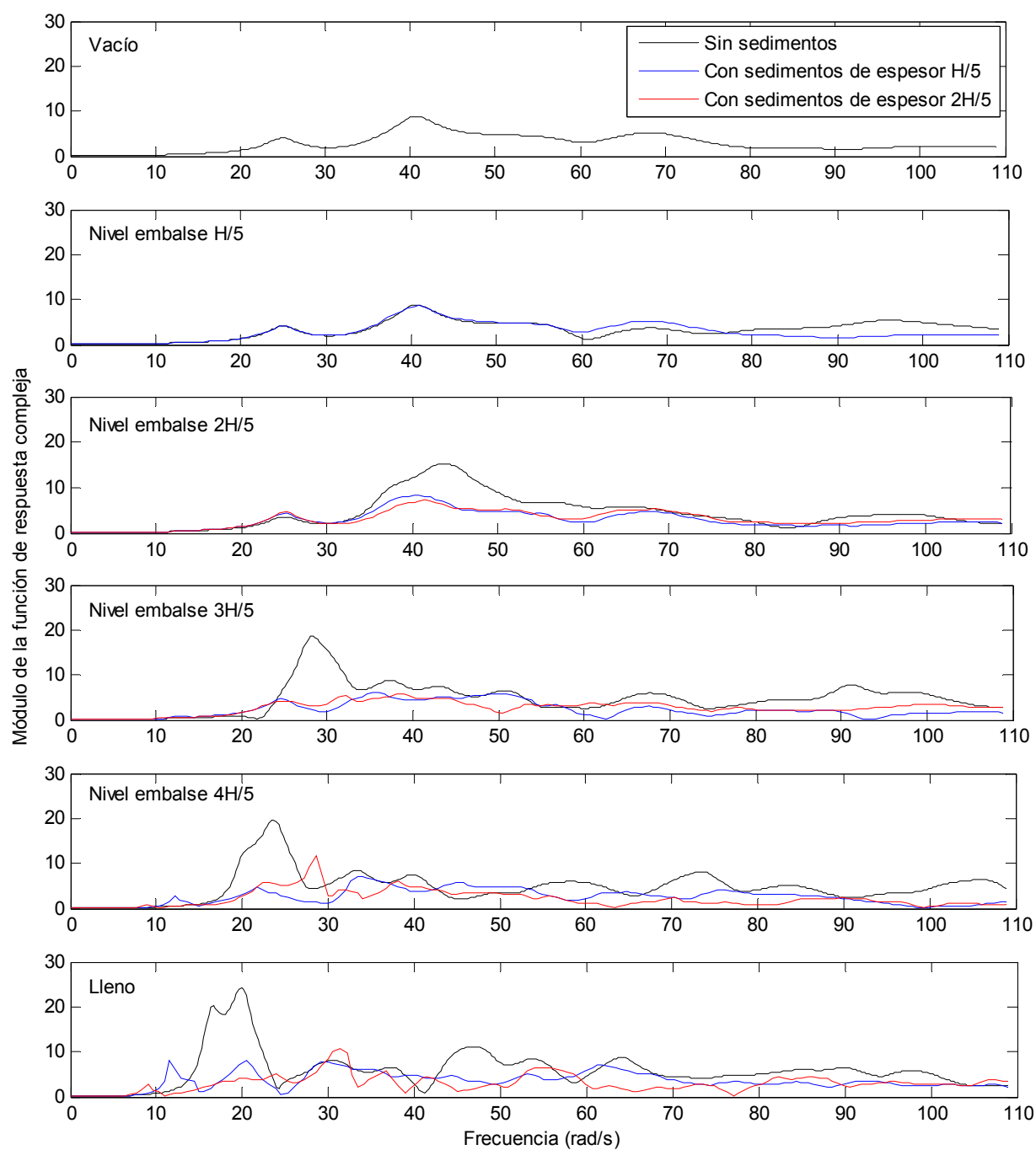
Figura 6.7. Módulo de la función de respuesta compleja en dirección x. Nodo C1. Onda P con incidencia vertical.
