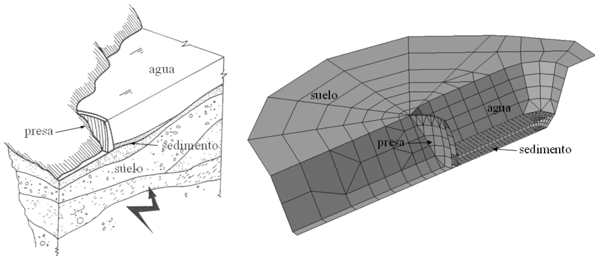
Figura 1.3. Sistema acoplado presa-suelo-agua-sedimento y modelo correspondiente de elementos de contorno.
