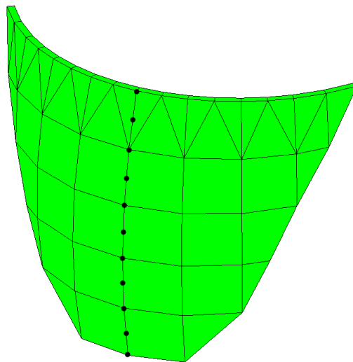
Figura 7.2. Puntos del plano de simetría de la bóveda en los que se han calculado las envolventes del empuje hidrodinámico normal.
