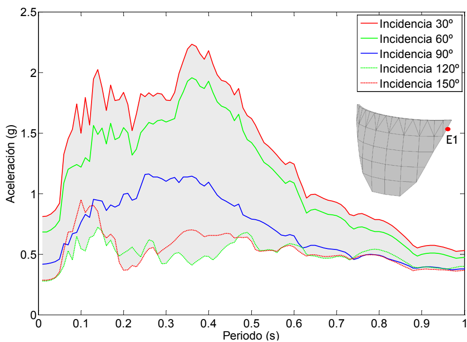
Figura 7.35. Nodo E1. Onda P+SV. Embalse sin sedimentos. Espectro de aceleraciones en dirección y.
