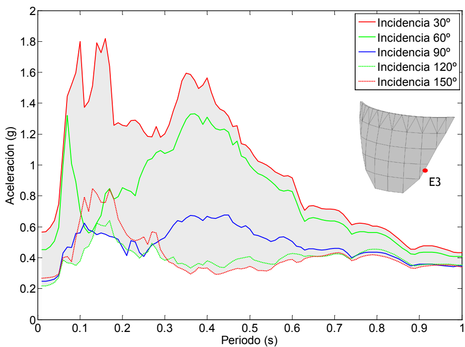
Figura 7.44. Nodo E3. Onda P+SV. Embalse con una capa de sedimentos de espesor H/5 . Espectro de aceleraciones en dirección y.
