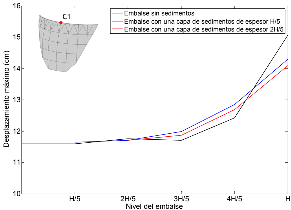
Figura 6.12. Nodo C1. Onda SH. Desplazamientos máximos en dirección x frente al nivel de llenado del embalse.
