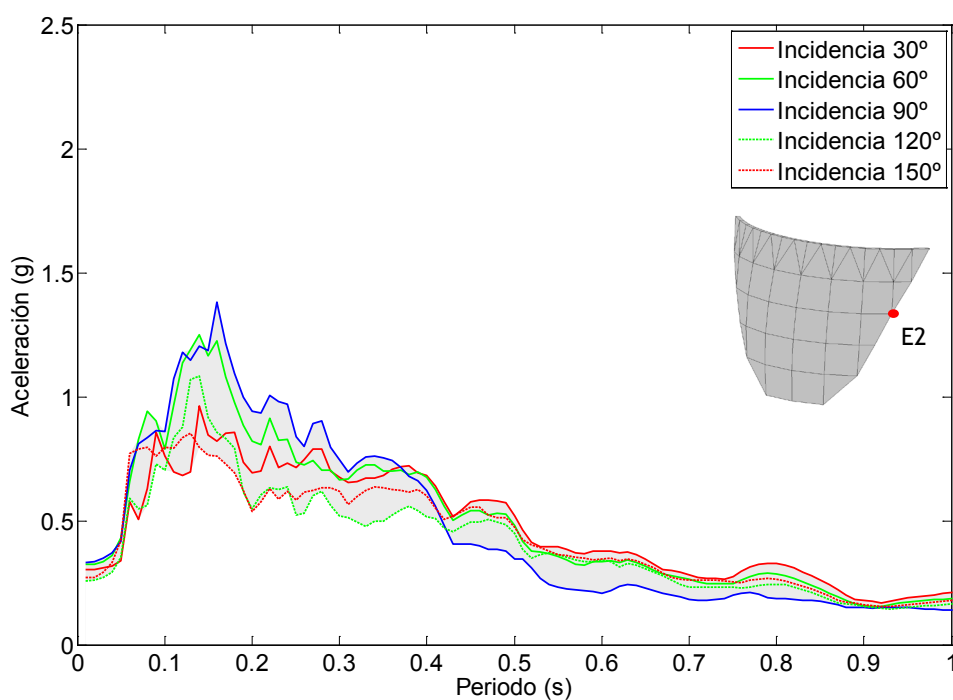
Figura 7.52. Nodo E2. Onda P+SV. Embalse con una capa de sedimentos de espesor H/5 . Espectro de aceleraciones en dirección z.
