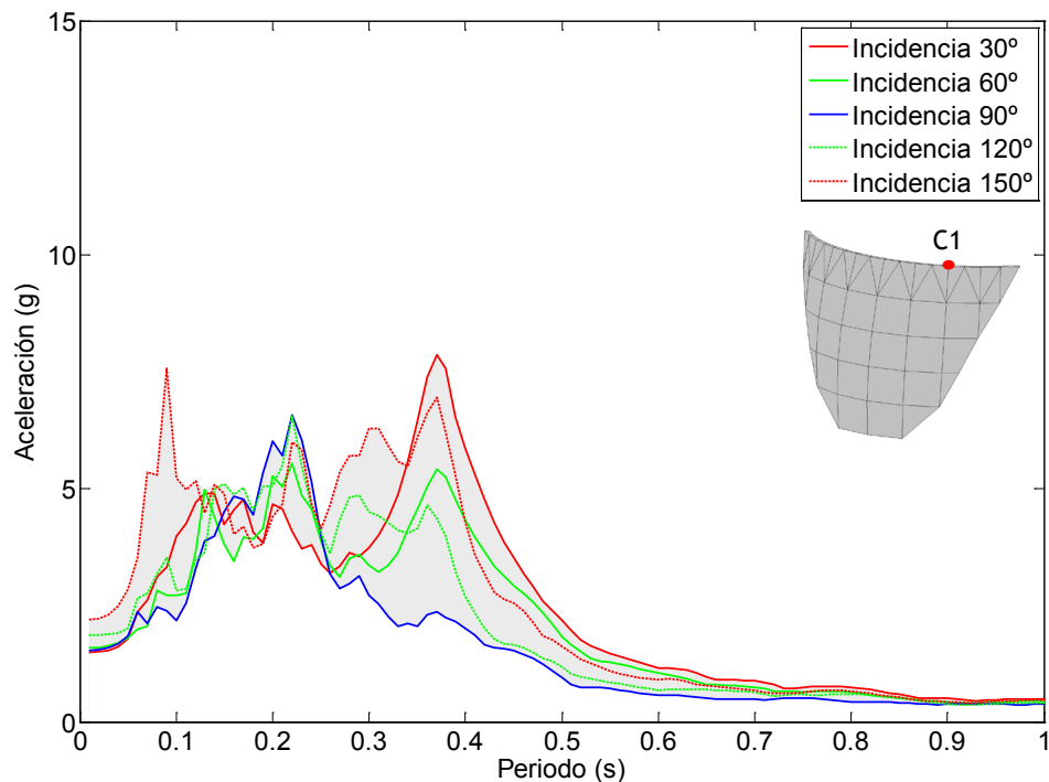
Figura 7.118. Nodo C1. Onda P+SH+SV. Embalse sin sedimentos. Espectro de aceleraciones en dirección y.
