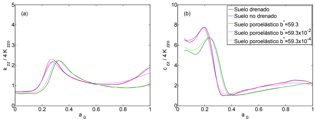
Figura 3.13. Influencia de la permeabilidad del suelo. Impedancia vertical. Grupo de pilotes 2 x 2 con s/d = 10 .
