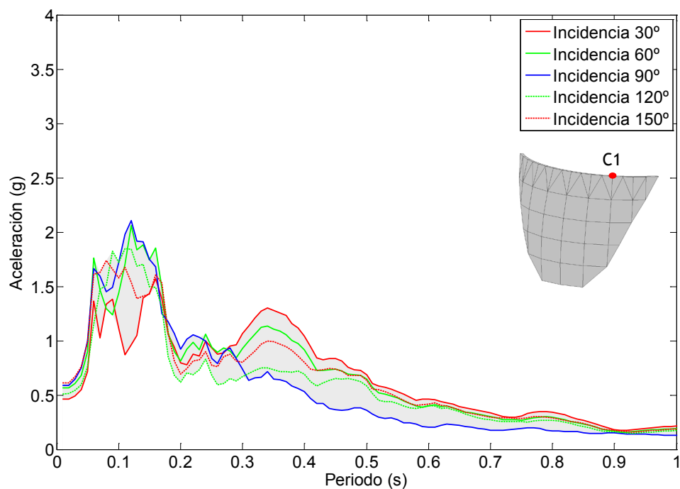
Figura 7.108. Nodo C1. Onda P+SV. Embalse con una capa de sedimentos de espesor 2H/5 . Espectro de aceleraciones en dirección z.
