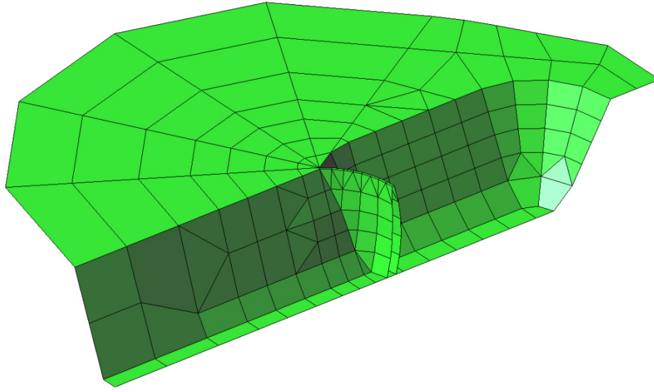
Figura 4.14. Modelo de elementos de contorno para la presa de Morrow Point.
