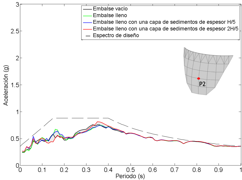
Figura 6.34. Nodo P2. Onda SV. Espectro de aceleraciones en dirección y frente a diferentes condiciones del embalse.
