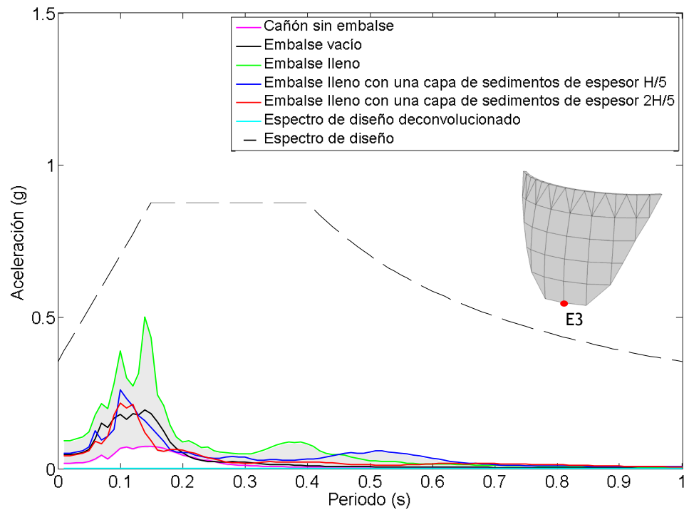
Figura 6.27. Nodo E3. Onda P. Espectro de aceleraciones en dirección x frente a diferentes condiciones del embalse.
