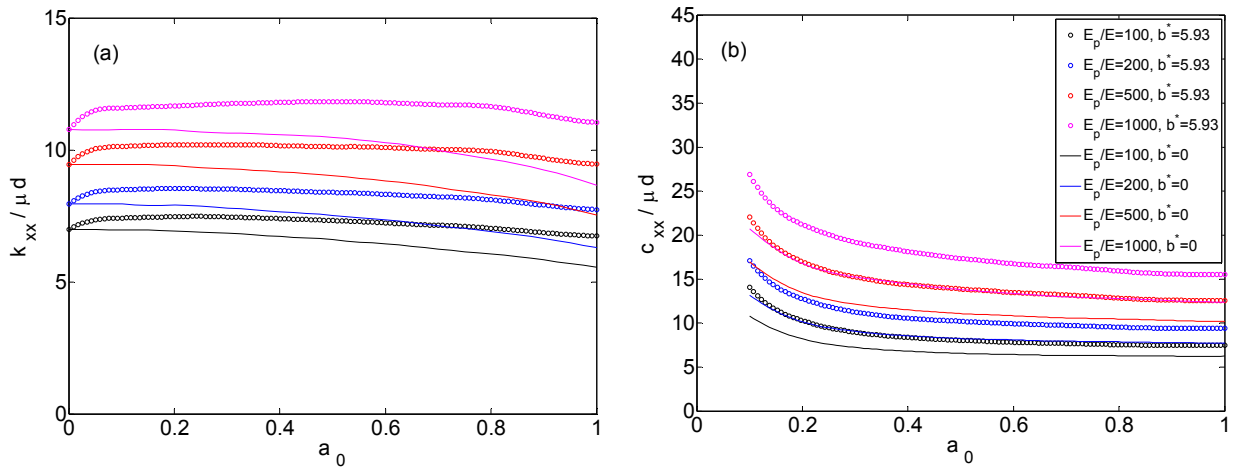
Figura 3.6. Influencia de la flexibilidad de los pilotes sobre la impedancia horizontal de pilotes simples.
