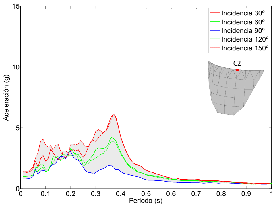
Figura 7.121. Nodo C2. Onda P+SH+SV. Embalse sin sedimentos. Espectro de aceleraciones en dirección y.
