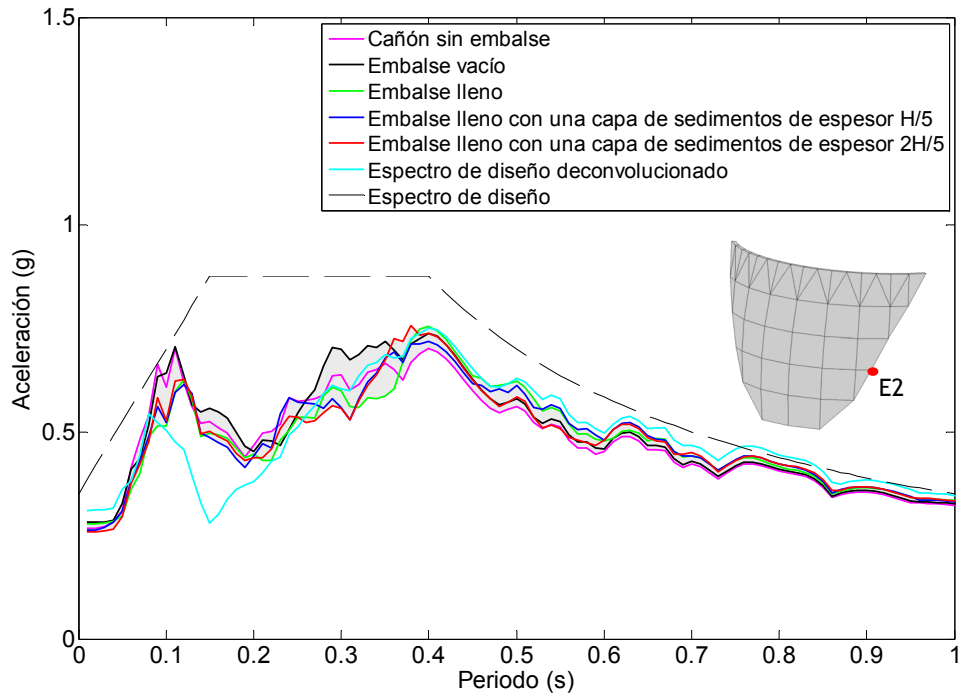
Figura 6.25. Nodo E2. Onda SH. Espectro de aceleraciones en dirección x frente a diferentes condiciones del embalse.
