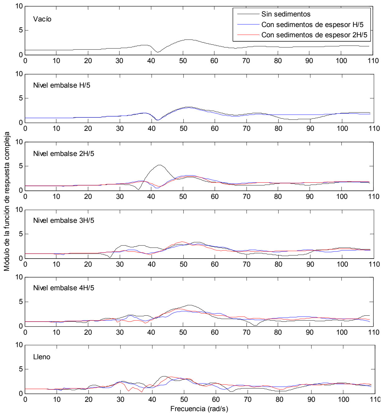
Figura 6.9. Módulo de la función de respuesta compleja en dirección z. Nodo C1. Onda P con incidencia vertical.
