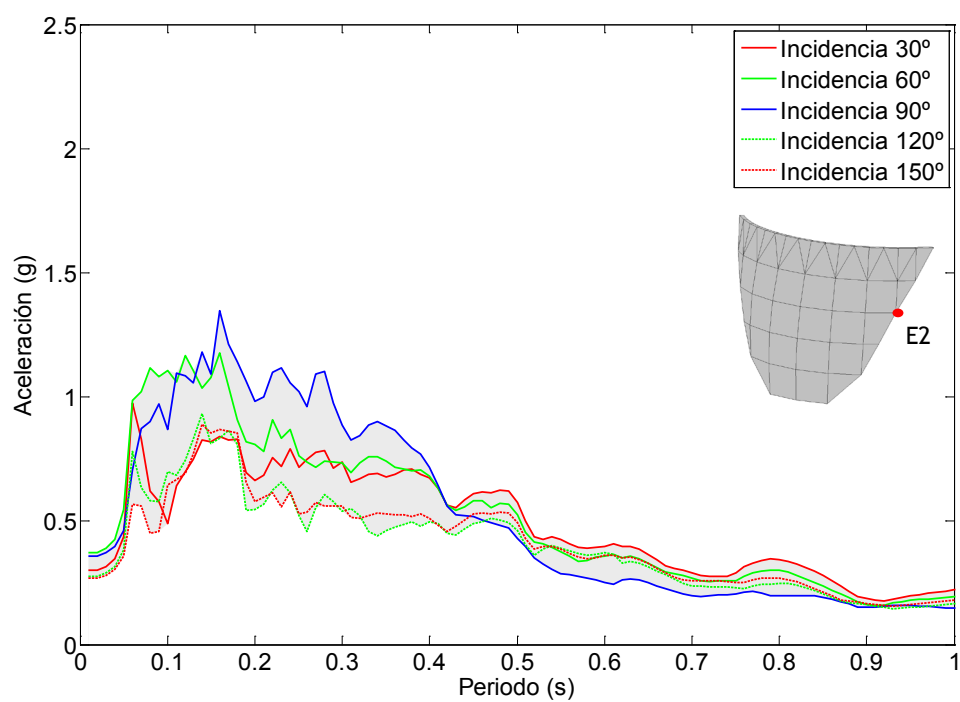
Figura 7.50. Nodo E2. Onda P+SV. Embalse sin sedimentos. Espectro de aceleraciones de campo libre en dirección z.
