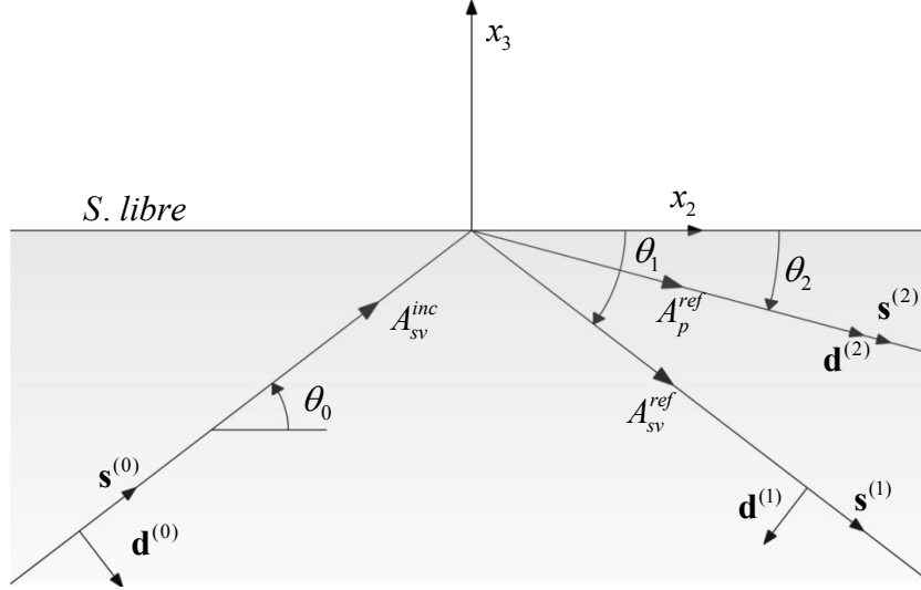
Figura 4.7. Ángulos de interés en el plano x_2x_3 para una onda SV incidente.
