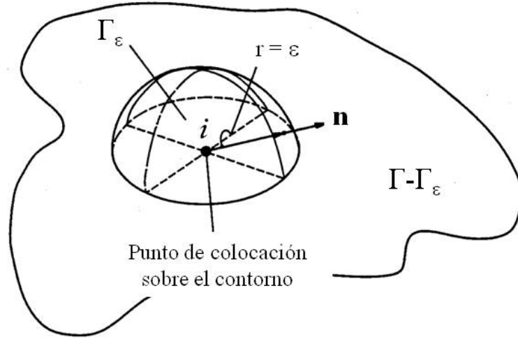
Figura 2.4. Descomposición en contornos \Gamma - \Gamma_\varepsilon y \Gamma_\varepsilon para “esquivar” la singularidad.
