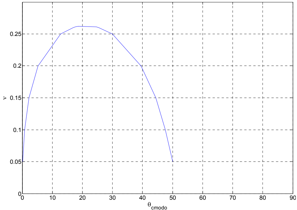
Figura 4.6. Ángulos de cambio de modo ( \theta_{cmodo} ) para una onda incidente tipo P en función del coeficiente de Poisson del terreno.
