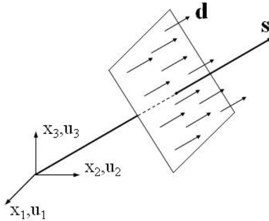
Figura 2.1. Desplazamiento y dirección de propagación para el caso de una onda plana P.
