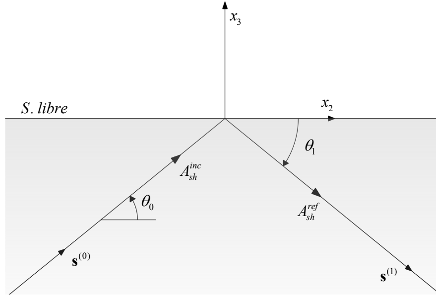
Figura 4.3. Ángulos de interés en el plano x_2x_3 para una onda SH incidente.
