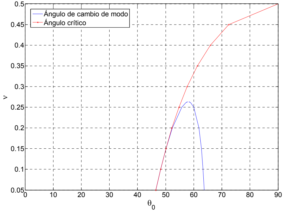
Figura 4.10. Ángulo de cambio de modo ( \theta_{cmodo} ) y ángulo crítico ( \theta_{cr} ) para una onda incidente tipo SV en función del coeficiente de Poisson del terreno.
