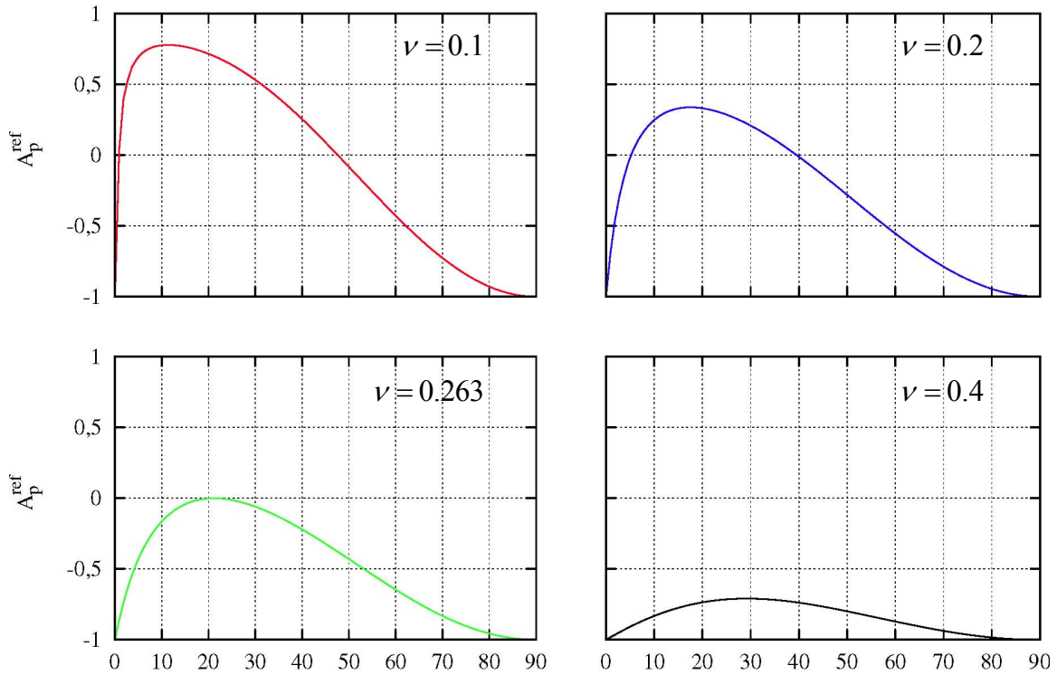
Figura 4.5. Variación de la amplitud de la onda P reflejada con el ángulo de incidencia \theta_0 y el coeficiente de Poisson \nu del terreno.
