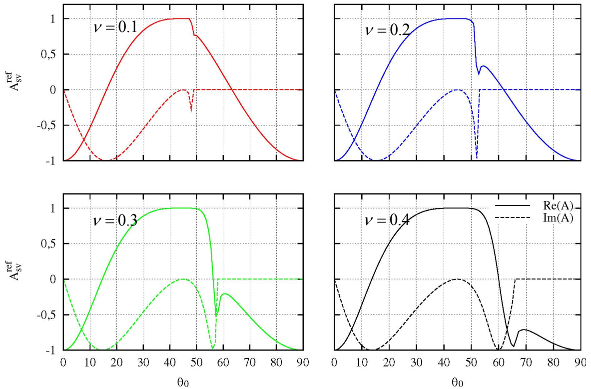
Figura 4.8. Variación de la amplitud de la onda SV reflejada con el ángulo de Incidencia \theta_0 .
