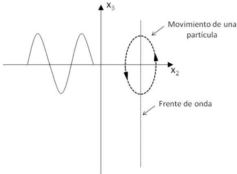
Figura 4.11. Propagación y movimiento de una partícula provocado por una onda de Rayleigh.
