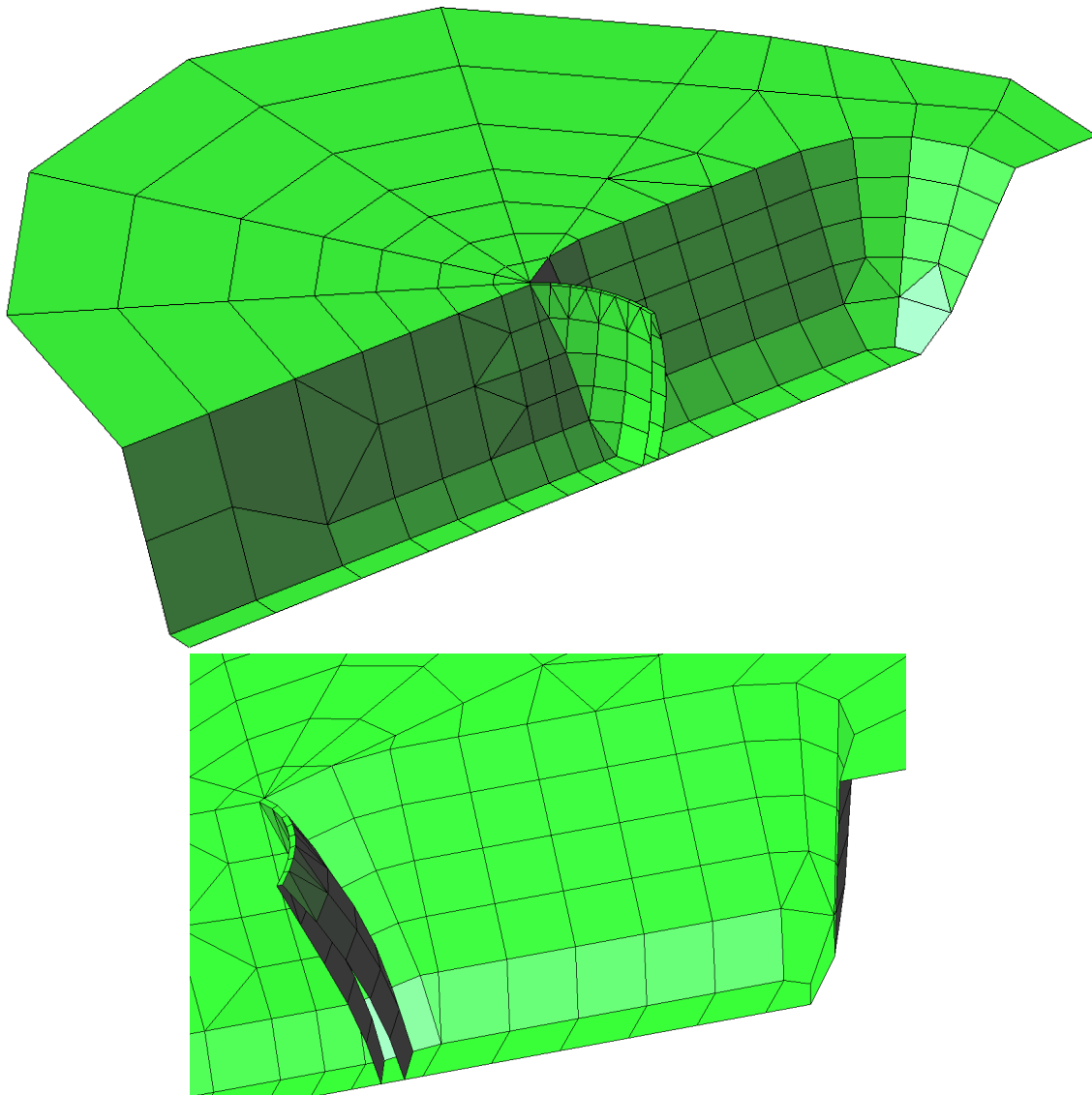
Figura 6.3. Discretización de elementos de contorno del sistema acoplado sin sedimentos. 218 elementos y 1004 nodos.
