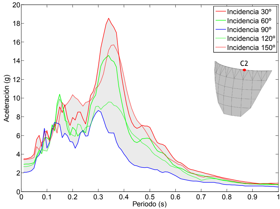
Figura 7.116. Nodo C2. Onda P+SH+SV. Embalse con una capa de sedimentos de espesor H/5 . Espectro de aceleraciones en dirección x.
