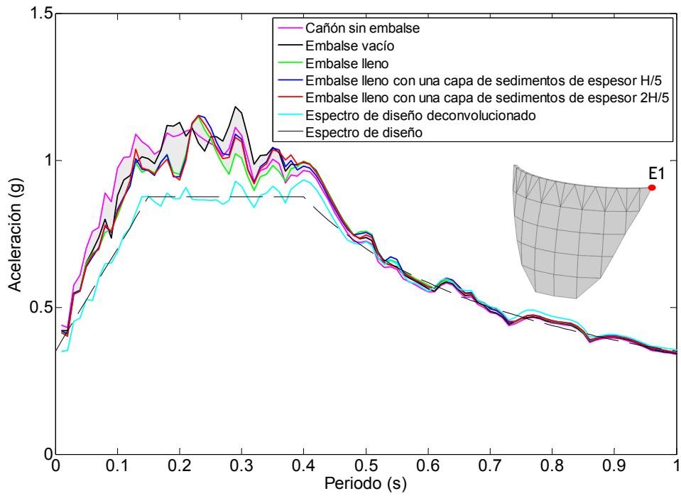
Figura 6.21. Nodo E1. Onda SH. Espectro de aceleraciones en dirección x frente a diferentes condiciones del embalse.
