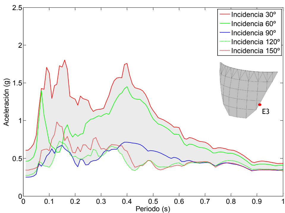
Figura 7.79. Nodo E3. Onda P+SH+SV. Embalse sin sedimentos. Espectro de aceleraciones en dirección y.
