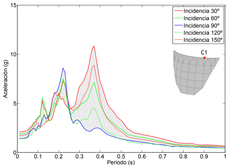
Figura 7.94. Nodo C1. Onda SH. Embalse sin sedimentos. Espectro de aceleraciones en dirección x.
