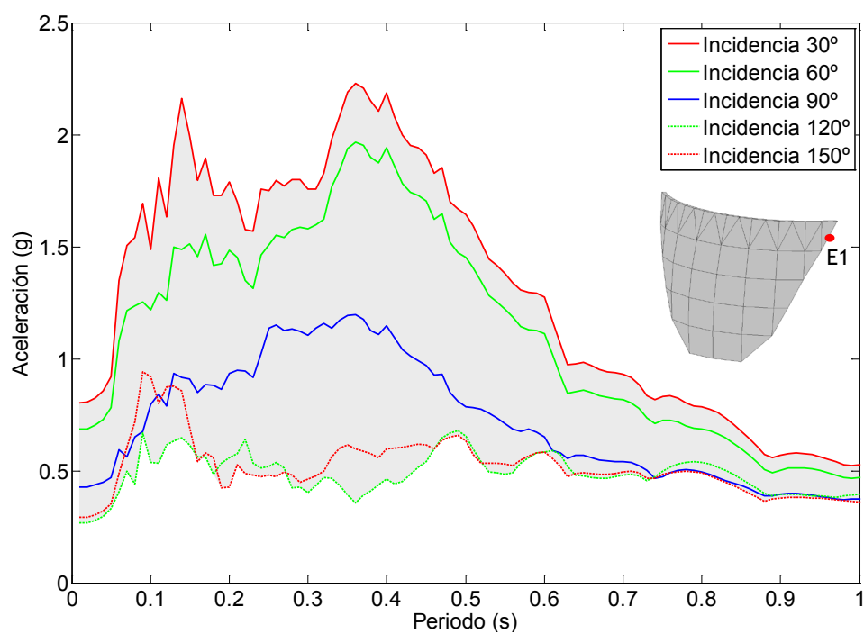
Figura 7.36. Nodo E1. Onda P+SV. Embalse con una capa de sedimentos de espesor H/5 . Espectro de aceleraciones en dirección y.
