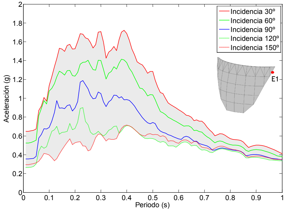
Figura 7.25. Nodo E1. Onda SH. Embalse con una capa de sedimentos de espesor 2H/5 . Espectro de aceleraciones en dirección x.
