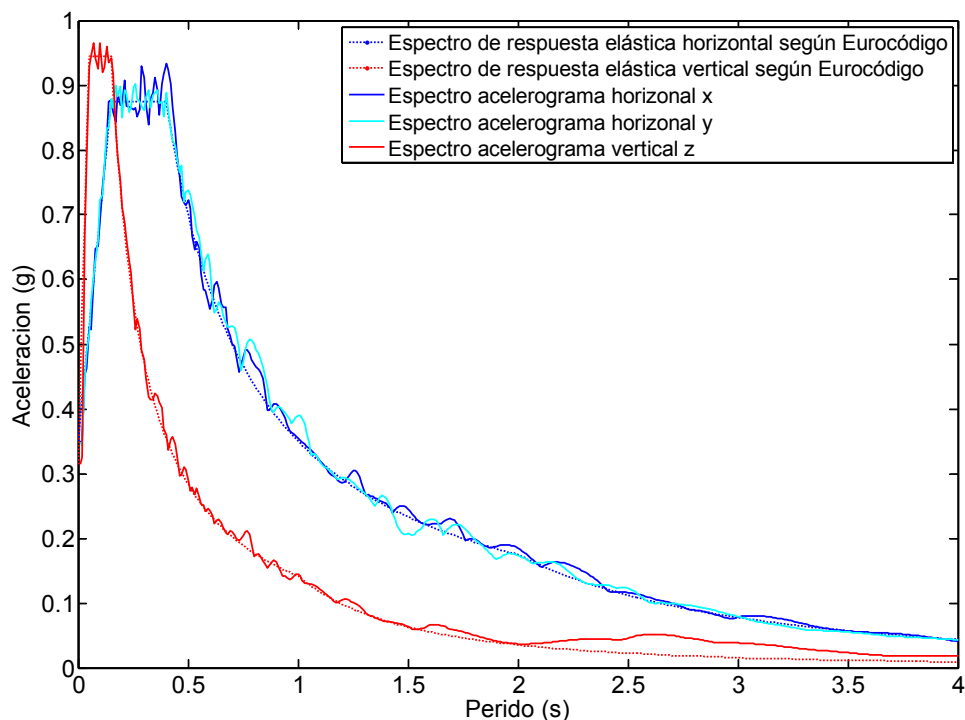
Figura 5.10. Espectros de los acelerogramas artificiales una vez corregidos comparados con los de diseño.
