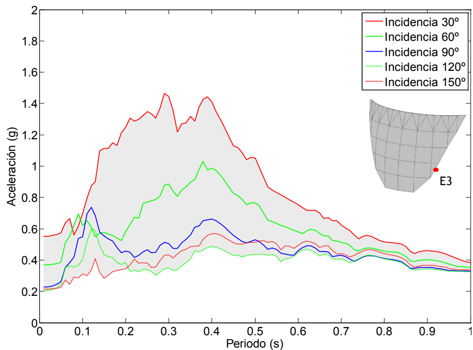
Figura 7.33. Nodo E3. Onda SH. Embalse con una capa de sedimentos de espesor 2H/5 . Espectro de aceleraciones en dirección x.
