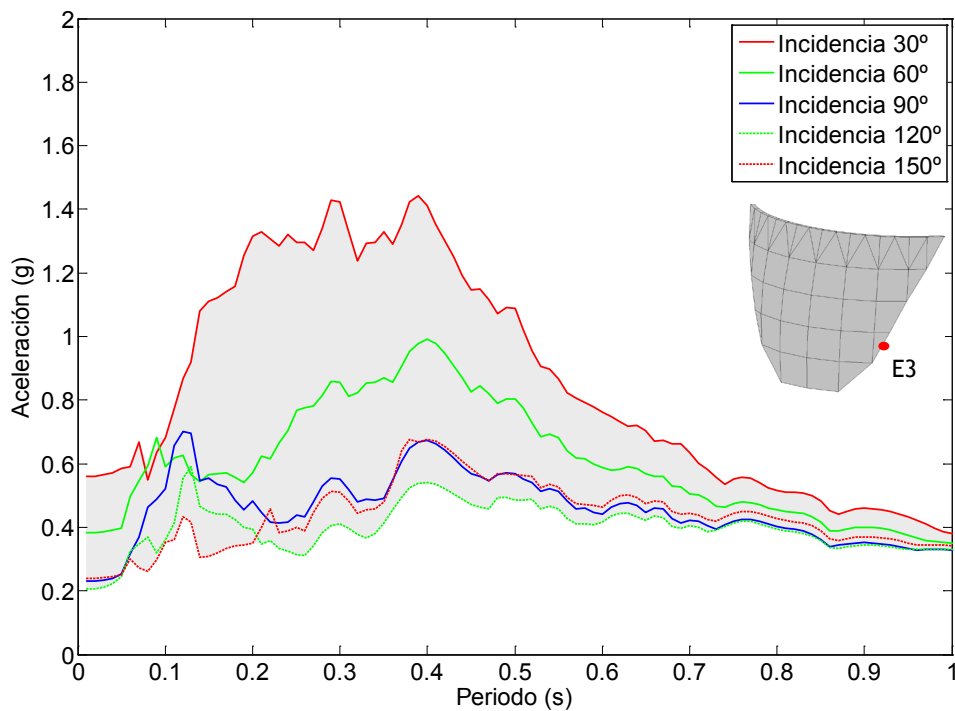
Figura 7.31. Nodo E3. Onda SH. Embalse sin sedimentos. Espectro de aceleraciones en dirección x.
