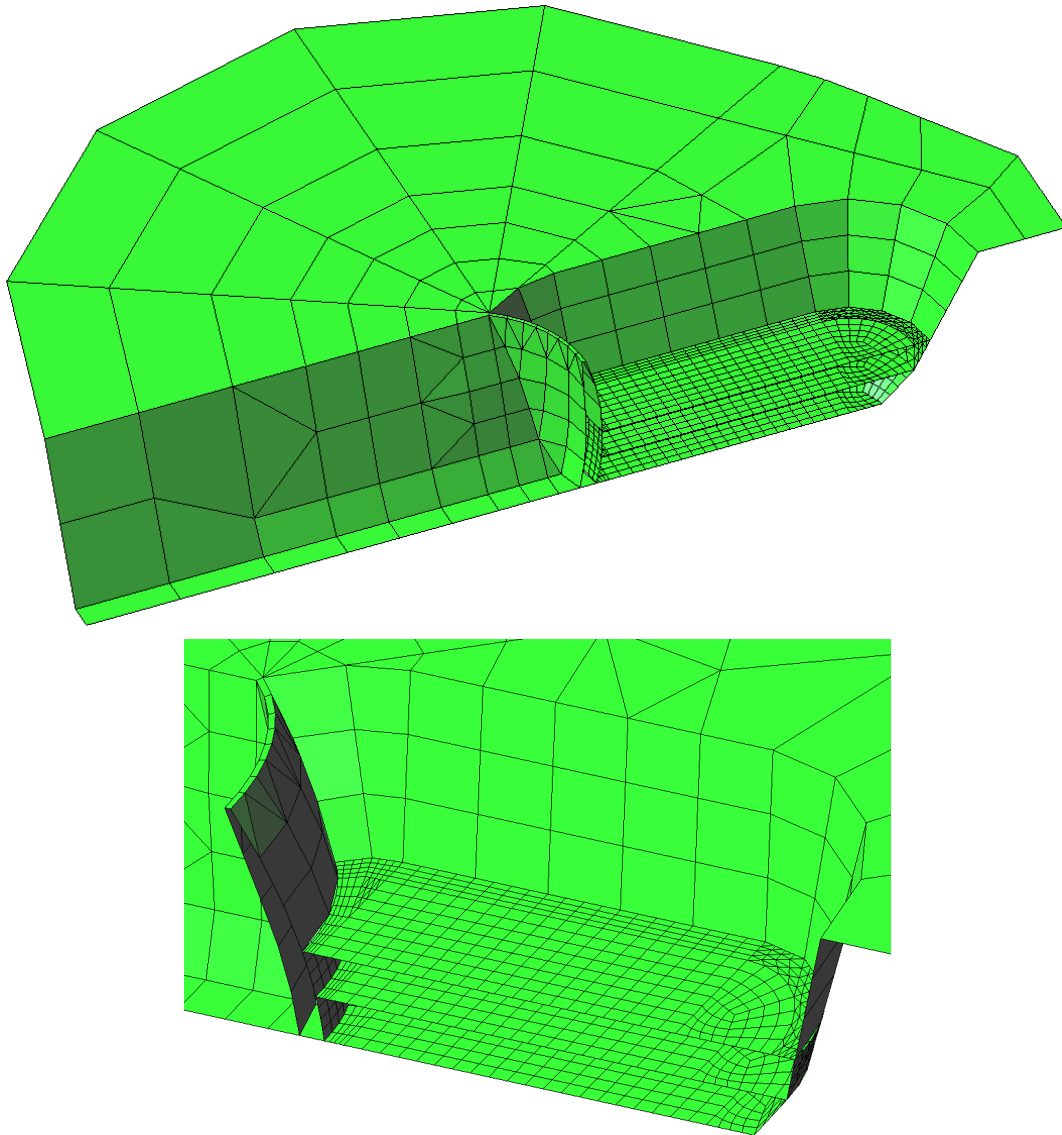
Figura 6.5. Discretización de elementos de contorno del sistema acoplado cuando el modelo incorpora una capa de sedimentos de espesor 2H/5 . 1448 elementos y 5727 nodos.
