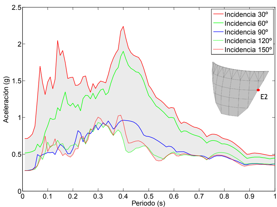
Figura 7.75. Nodo E2. Onda P+SH+SV. Embalse sin sedimentos. Espectro de aceleraciones en dirección y.
